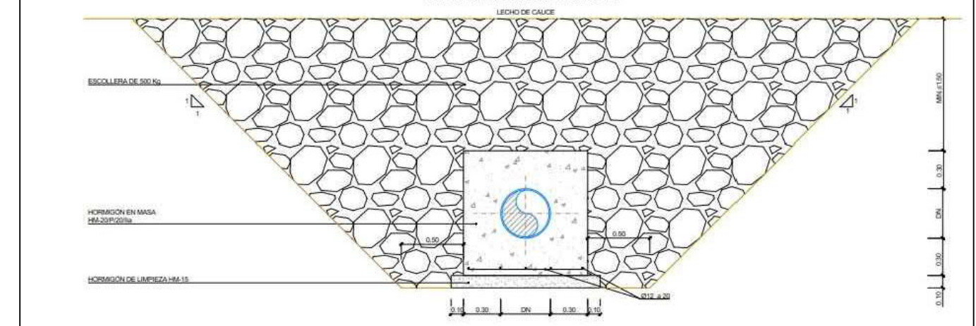
ST-3. SECCIÓN BAJO ARROYO
