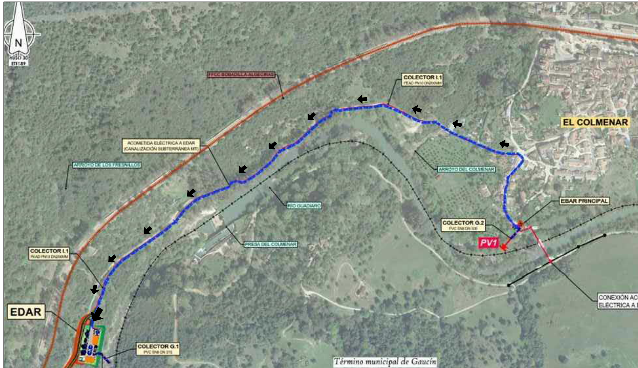
ACCESO ACTUACION EN EDAR
