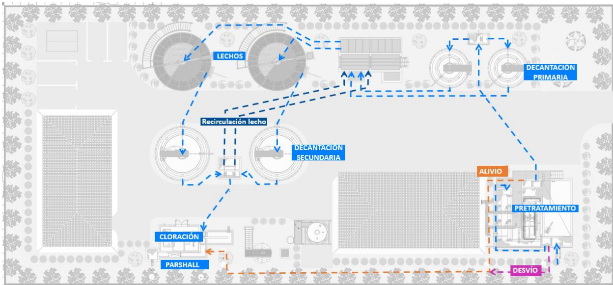
Esquema línea agua EDAR
