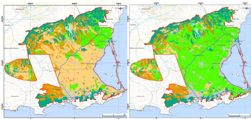
Figura 4: Usos del Suelo en la masa de agua subterránea Campo de Cartagena. Periodo 1980-1990 (izquierda) y Periodo 2000-2009 (derecha) según el “Mapa de Cultivos y Aprovechamientos de España” MCA (MAPAMA, 2009)
