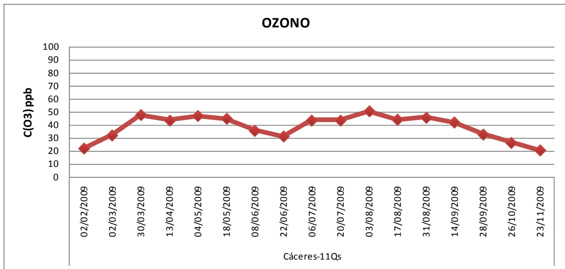
Figura 19: Concentraciones promedio de ozono (ppb) en el año 2009
