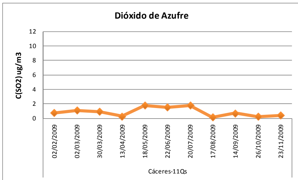
Figura 20: Concentraciones promedio de Dióxido de Azufre (SO 2 µg/m 3 ) durante el año 2009
