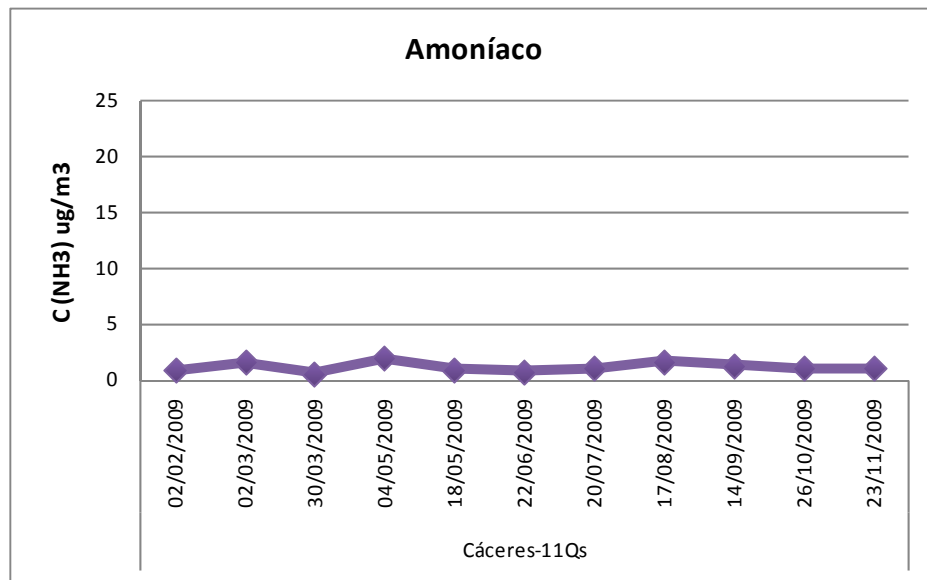
Figura 21: Concentraciones promedio de Amoníaco (NH 3 ug/m 3 ) entre durante el año 2009
