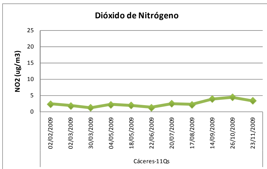
Figura 18: Concentraciones promedio de Dióxido de Nitrógeno (NO 2 µg/m 3 ) en el año 2009
