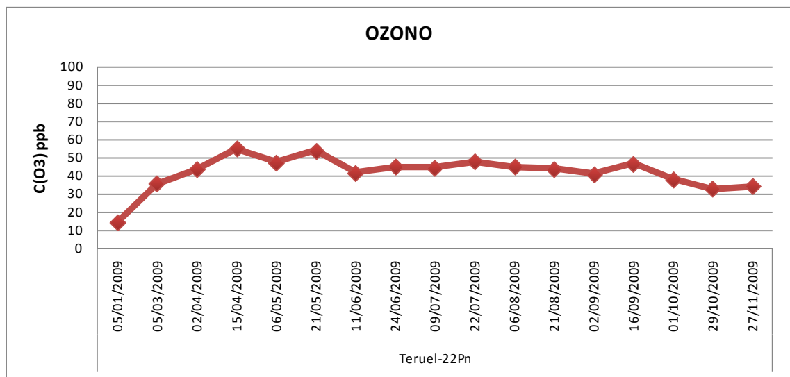
Figura 27: Concentraciones promedio de ozono (ppb) en el año 2009
