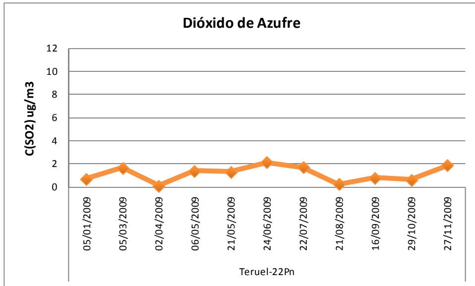
Figura 28: Concentraciones promedio de Dióxido de Azufre (SO 2 ug/m 3 ) durante el año 2009
