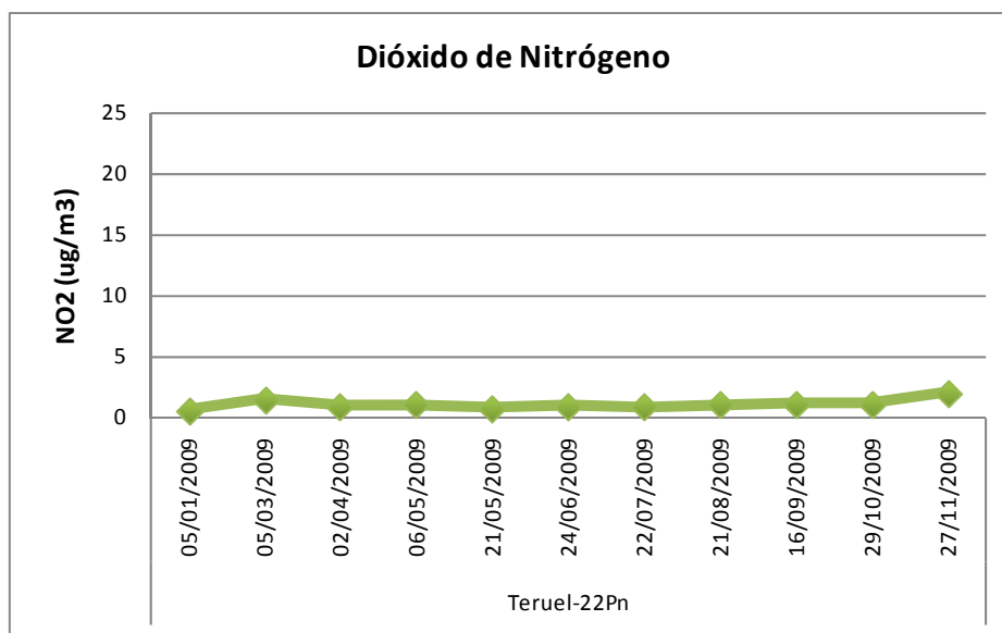
Figura 26: Concentraciones promedio de Dióxido de Nitrógeno (NO 2 µg/m 3 ) en el año 2009
