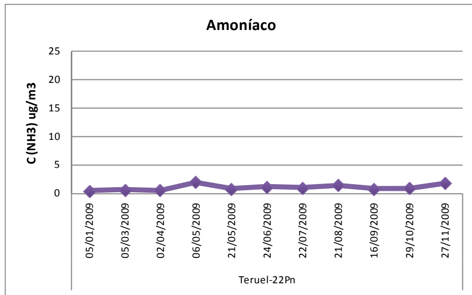
Figura 29: Concentraciones promedio de Amoníaco (NH 3 ug/m 3 ) entre durante el año 2009
