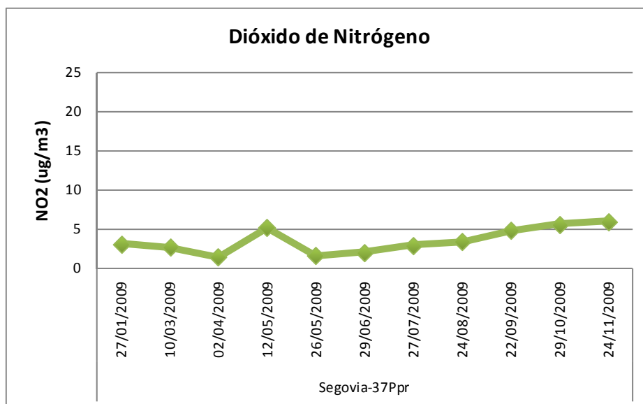
Figura 46: Concentraciones promedio de Dióxido de Nitrógeno (NO 2 µg/m 3 ) en el año 2009
