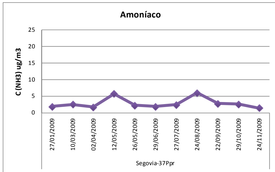
Figura 49: Concentraciones promedio de Amoníaco (NH 3 ug/m 3 ) entre durante el año 2009
