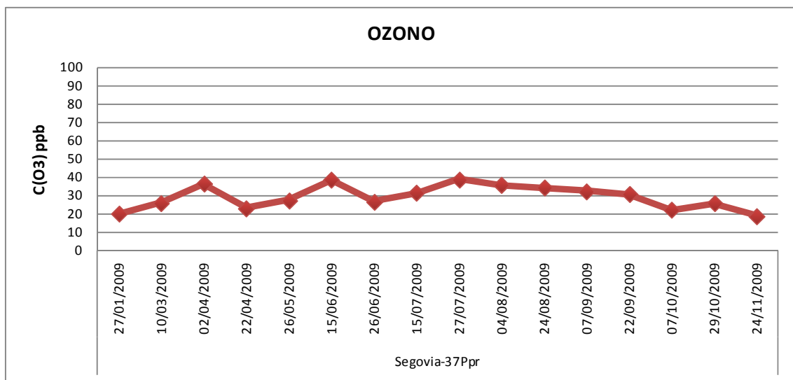
Figura 47: Concentraciones promedio de ozono (ppb) en el año 2009
