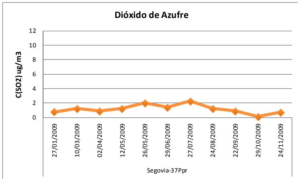
Figura 48: Concentraciones promedio de Dióxido de Azufre (SO 2 µg/m 3 ) durante el año 2009
