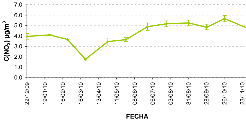
Figura 15: Concentraciones de Dióxido de Nitrógeno (NO 2 µg/m 3 ) en el año 2010 en la parcela de Almonte.
