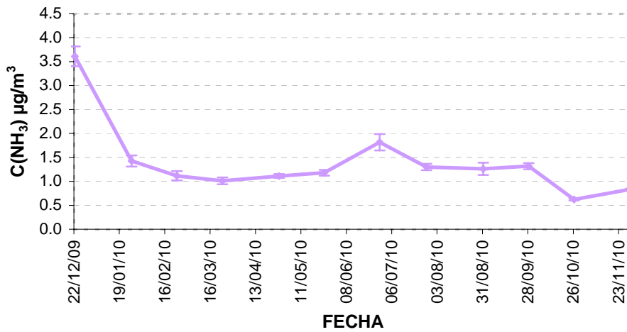
Figura 17: Concentraciones de Amoniac (NH 3 µg/m 3 ) entre durante el año 2010 en la parcela de Almonte.
