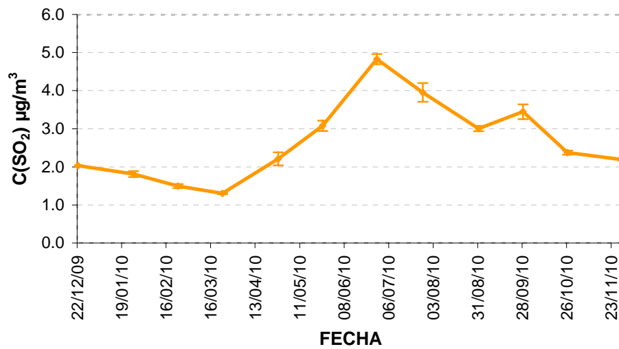
Figura 16: Concentraciones de Dióxido de Azufre (SO 2 µg/m 3 ) durante el año 2010 en la parcela de Almonte.
