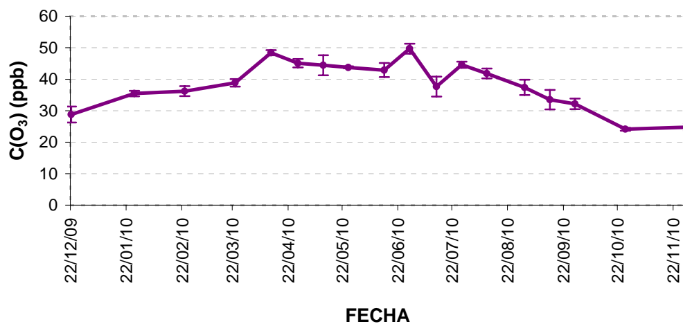
Figura 14: Concentraciones de ozono (ppb) en el año 2010 en la parcela de Almonte.
