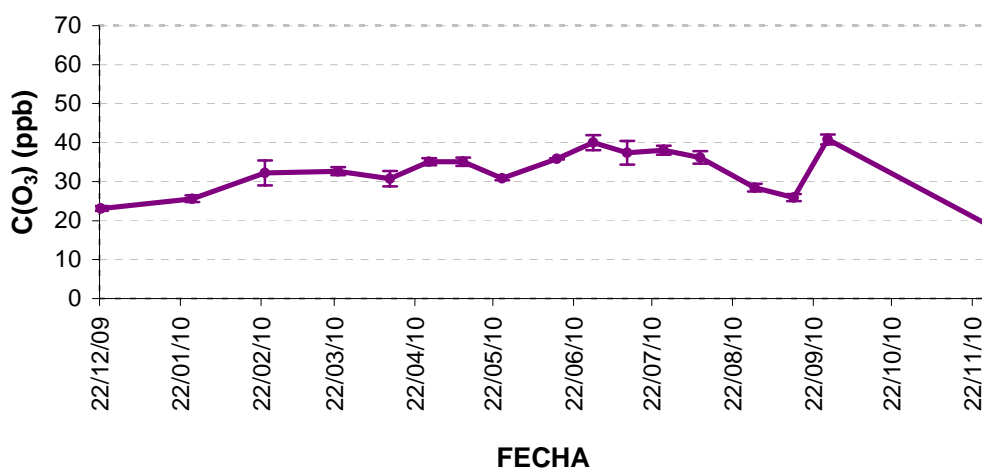
Figura 46: Concentraciones de ozono (ppb) en el año 2010 en la parcela de Cuéllar.
