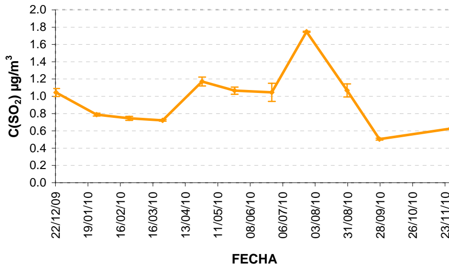
Figura 48: Concentraciones de Dióxido de Azufre (SO 2 µg/m 3 ) durante el año 2010 en la parcela de Cuéllar.
