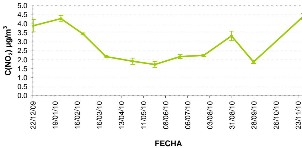
Figura 47: Concentraciones de Dióxido de Nitrógeno (NO 2 µg/m 3 ) en el año 2010 en la parcela de Cuéllar.
