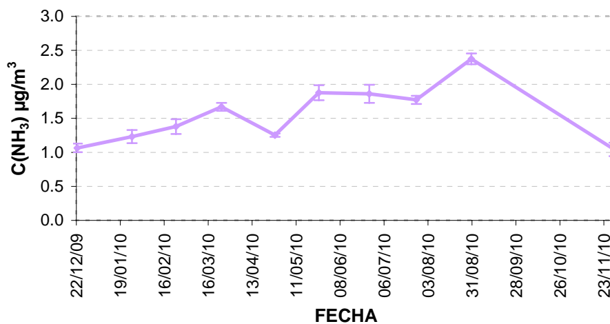
Figura 49: Concentraciones de Amoniacó (NH 3 µg/m 3 ) entre durante el año 2010 en la parcela de Cuéllar.
