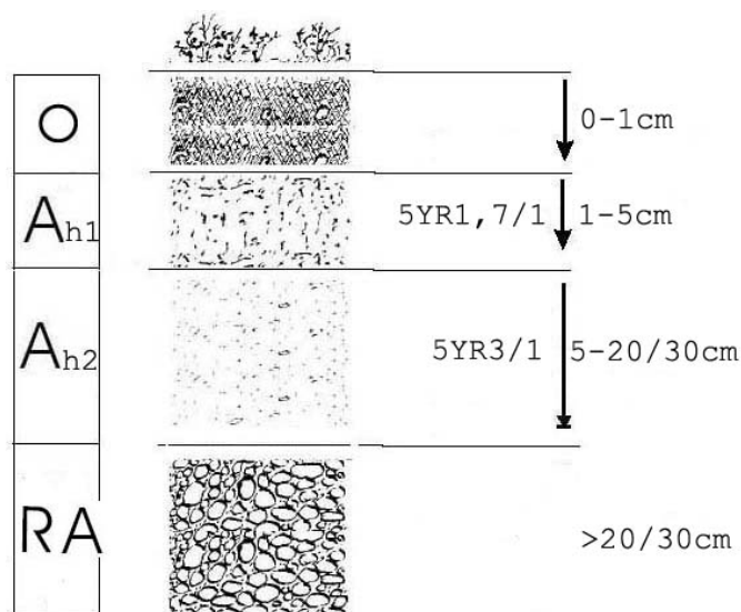
FIG 3: Esquema del perfil del suelo Rendzic Leptosol , fase rúdica de la parcela 40Qi
