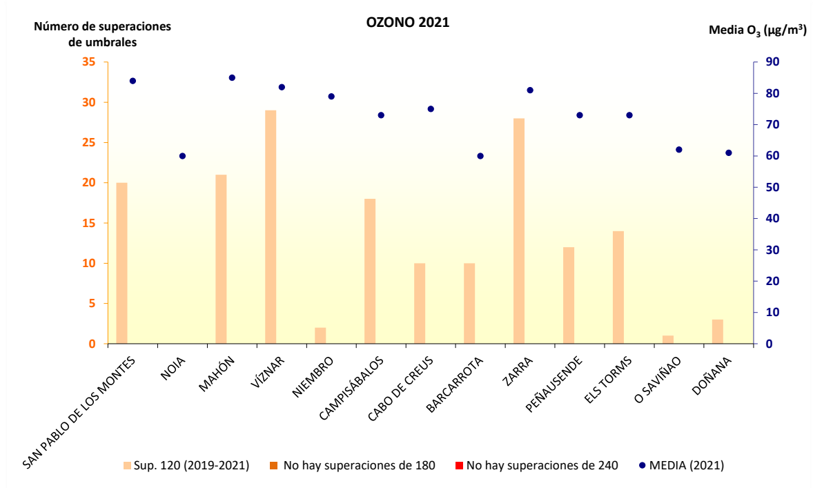
Figura 272. Media anual de O 3 : número de superaciones del máximo diario móvil octohorario (120 µg/m 3 )
