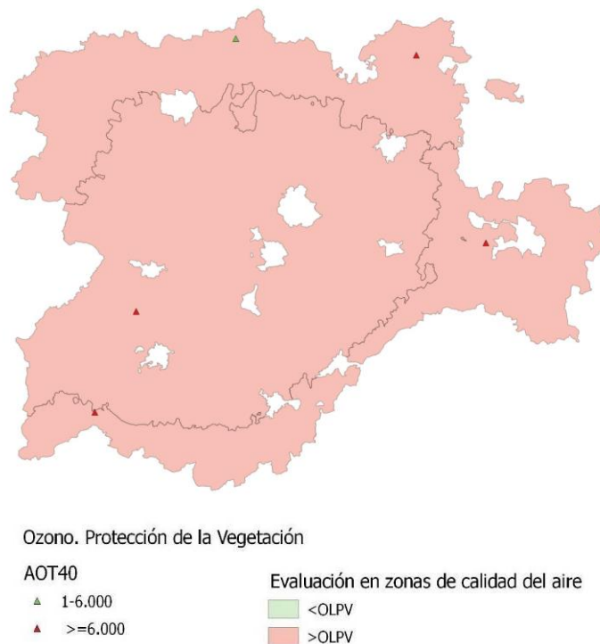
Figura 137. Número de superaciones en estaciones y evaluación por zonas del OLP de \text{O}_3 para la protección de la vegetación
