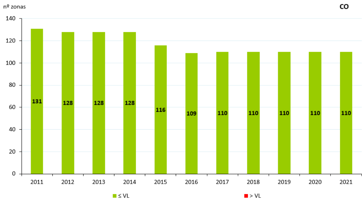
Figura 31. Evolución de las zonas de calidad del aire respecto al VL de CO (2011-2021)
