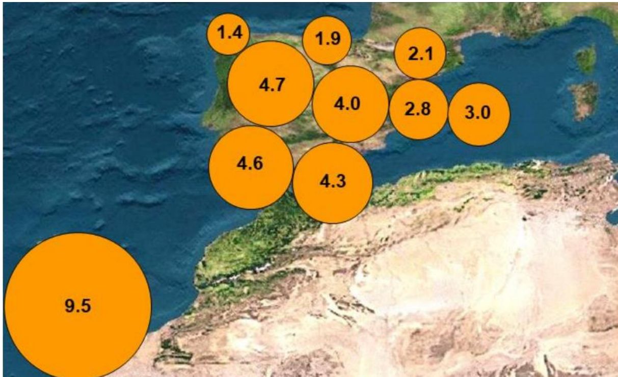
Figura 4. Contribución de polvo africano a PM10 en 2021 (fuente: CSIC)
