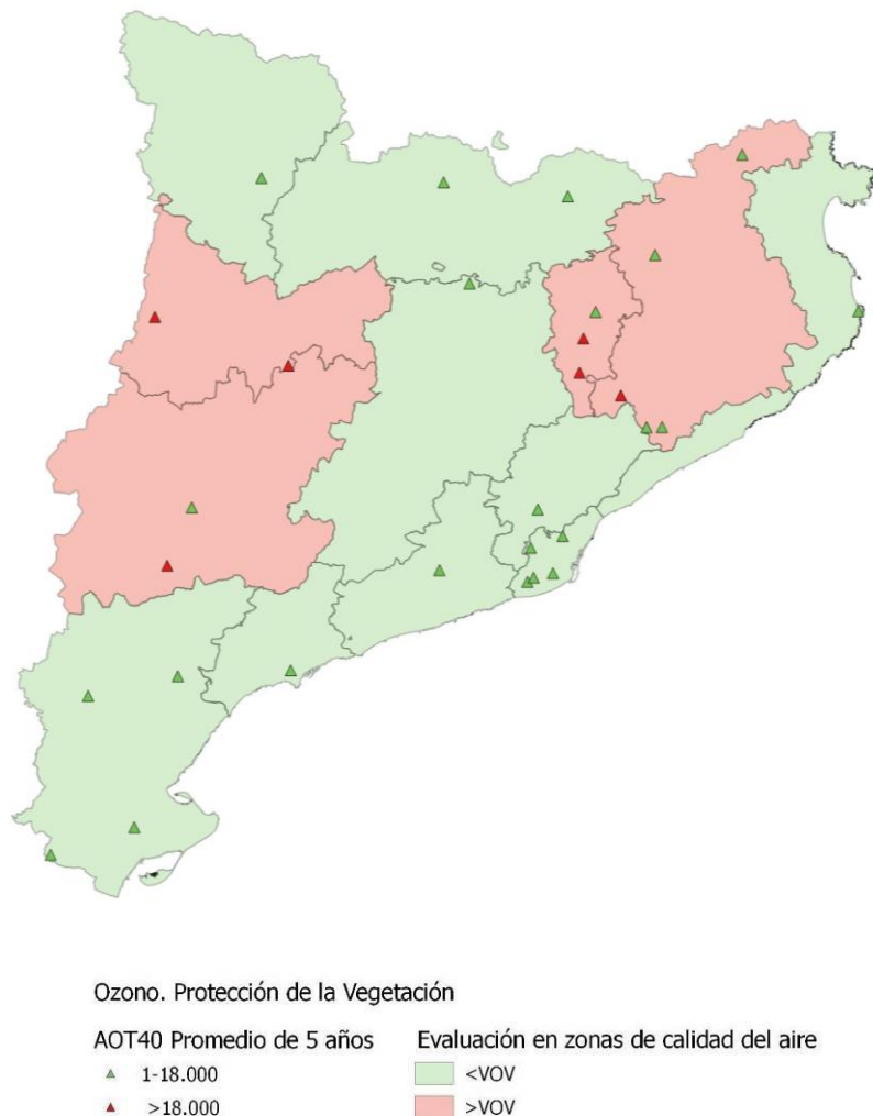
Figura 146. Número de superaciones en estaciones y evaluación por zonas del VO de \text{O}_3 para la protección de la vegetación
