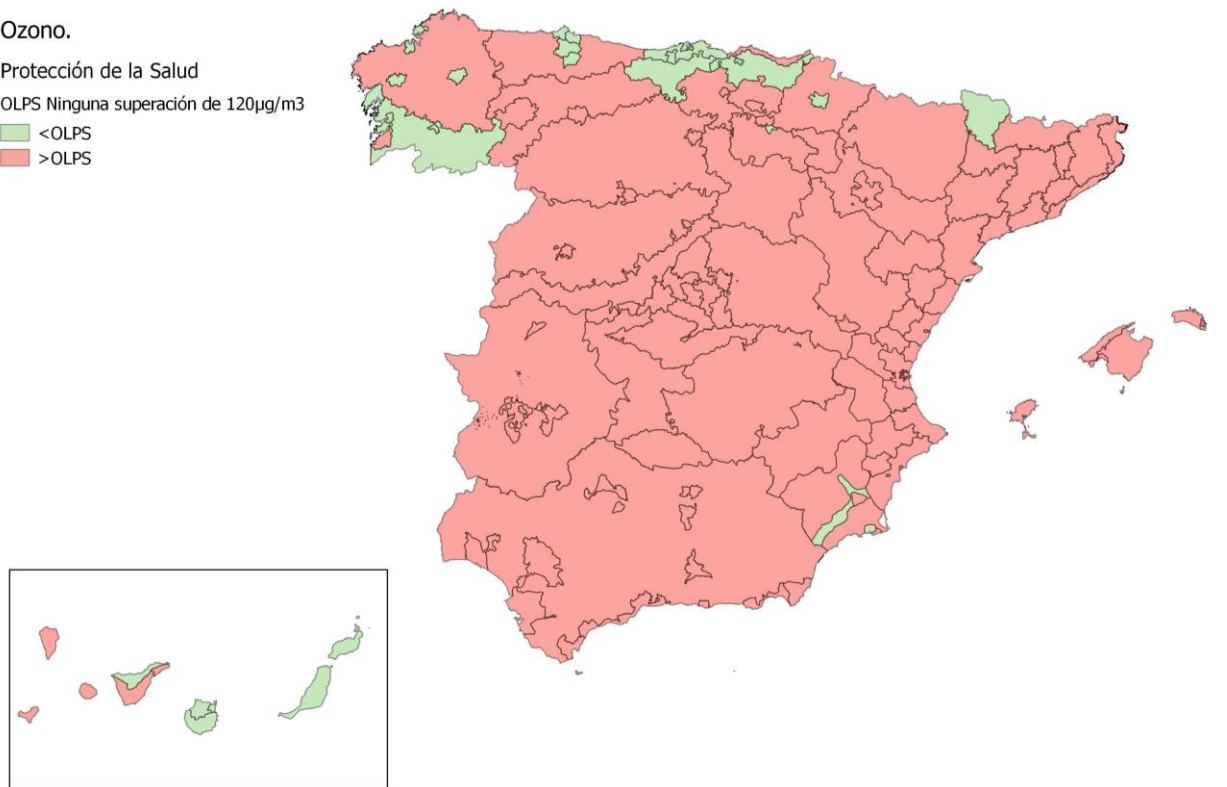
Figura 17. Situación de la calidad del aire de 2021 respecto al OLP de O 3 para la protección de la salud La evolución de las zonas de evaluación de O 3 y su situación respecto al VO-salud desde 2011 se muestra en la Figura 18, y respecto al OLP- salud, en la ¡Error! No se encuentra el origen de la referencia.:
