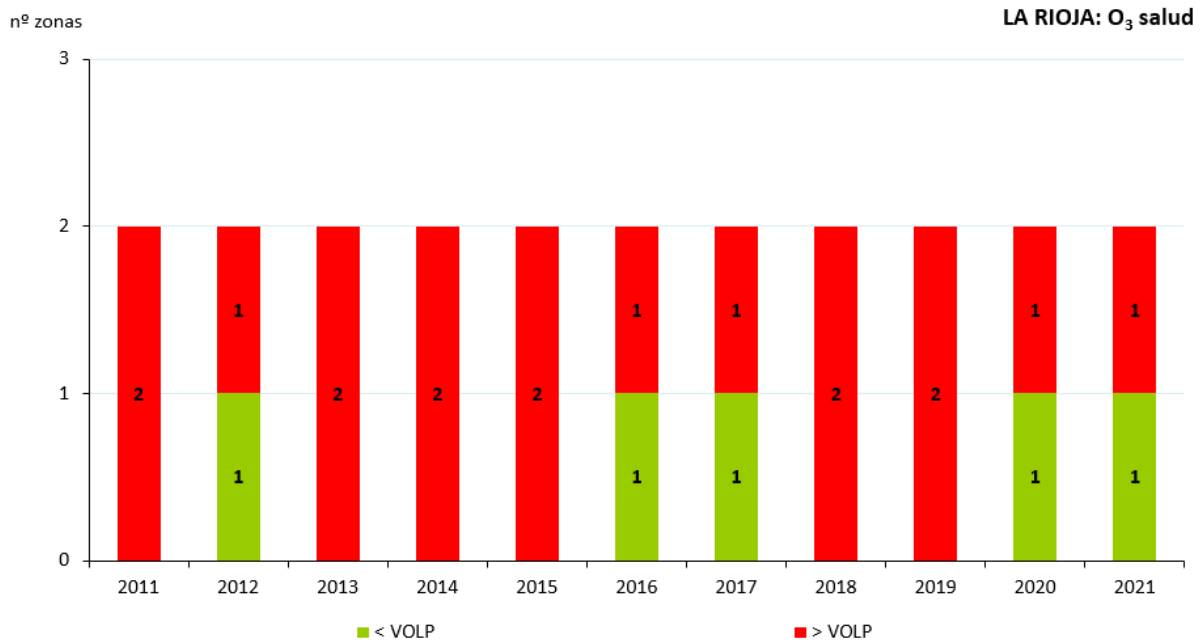
Figura 264. Evolución de las zonas de calidad del aire respecto al OLP-Salud de O 3 (2011-2021)
