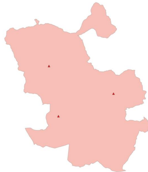
Ozono. Protección de la Vegetación AOT40 ▲ 1-6.000 ▲ \geq 6.000 Evaluación en zonas de calidad del aire ■ <OLPV ■ >OLPV
