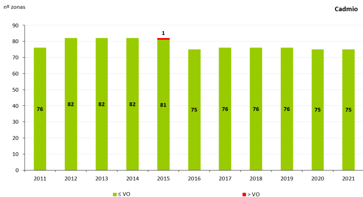
Figura 39. Evolución de las zonas de calidad del aire respecto al VO de Cd (2011-2021)
