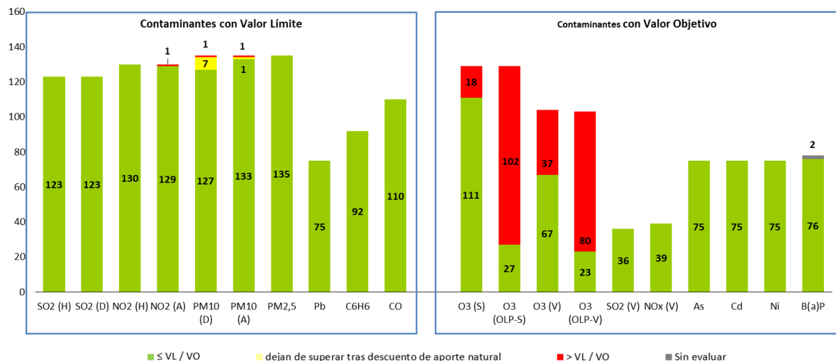
Figura 1. Resumen de la evaluación de la calidad del aire en 2021 por contaminante
