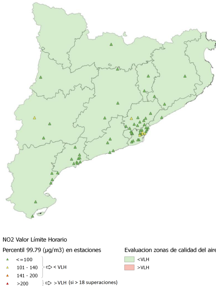
Figura 136. Percentil 99,79 en estaciones y evaluación por zonas del VLH de NO 2
