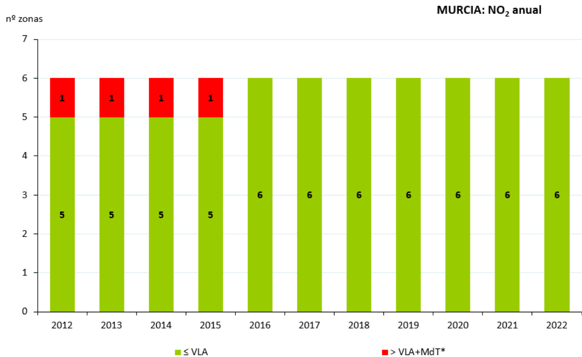
Figura 219. Evolución de las zonas de calidad del aire respecto al VLA de NO 2 (2012-2022)
