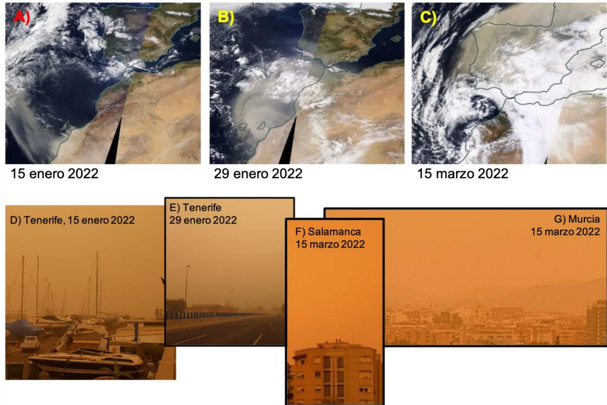
Figura 273. Imagen satélite (NASA) (A-C) y fotografías de varias zonas de España durante los eventos de super calima de polvo sahariano de 2022 (D-G).
