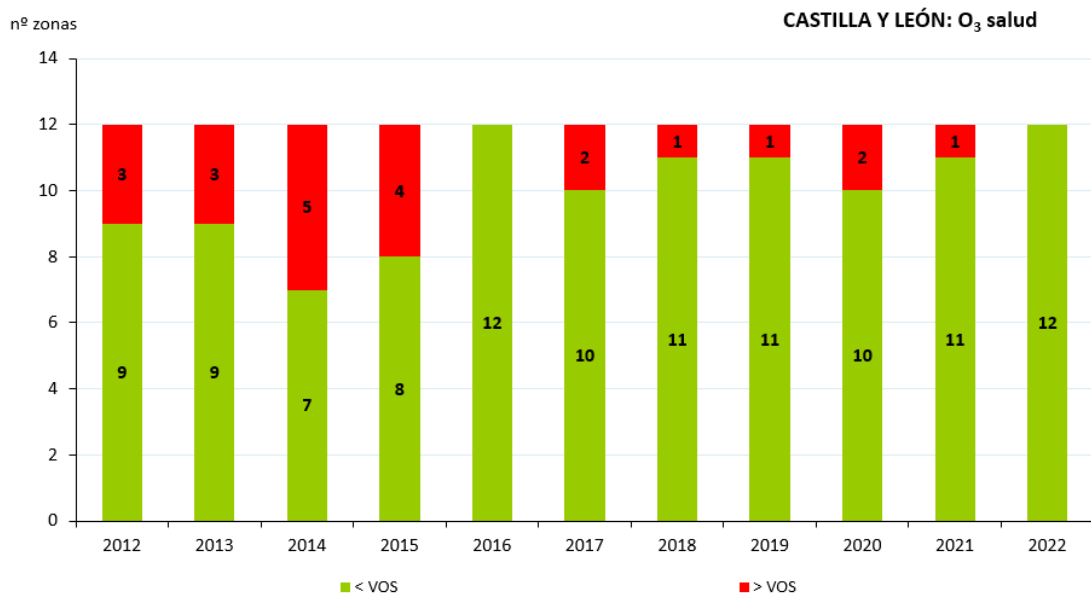
Figura 134. Evolución de las zonas de calidad del aire respecto al VO-Salud de O 3 (2012-2022)
