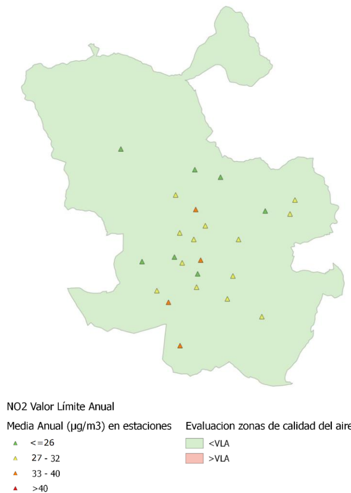
Figura 200. Media anual en estaciones y evaluación por zonas del VLA de \text{NO}_2
