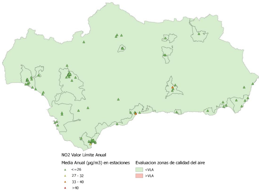
Figura 43. Media anual en estaciones y evaluación por zonas respecto al VLA de \text{NO}_2
