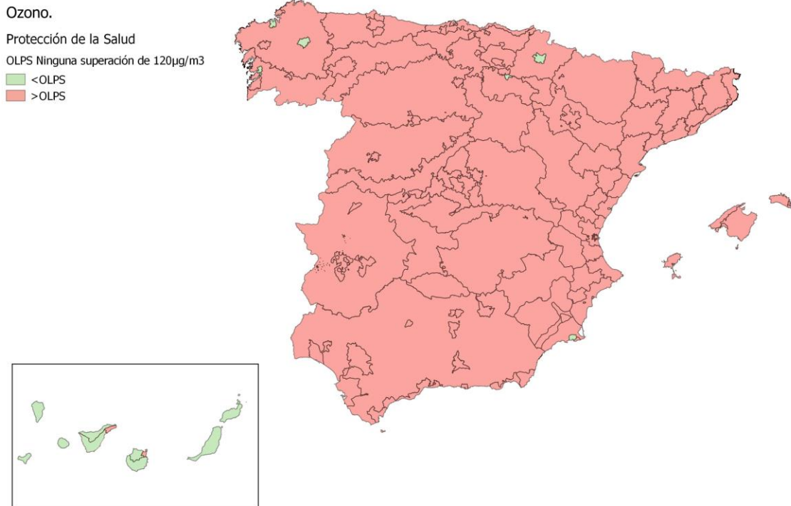
Figura 17. Situación de la calidad del aire de 2022 respecto al OLP de O 3 para la protección de la salud La evolución de las zonas de evaluación de O 3 y su situación respecto al VO-salud desde 2012 se muestra en la Figura 18, y respecto al OLP- salud, en la Figura 19:
