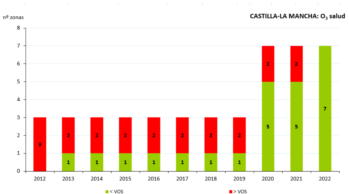
Figura 124. Evolución de las zonas de calidad del aire respecto al VO-Salud de O 3 (2012-2022)
