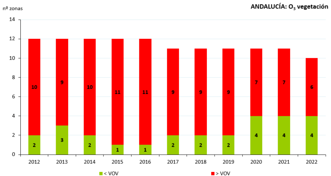
Figura 54. Evolución de las zonas de calidad del aire respecto al VO-Vegetación de O 3 (2012-2022)
