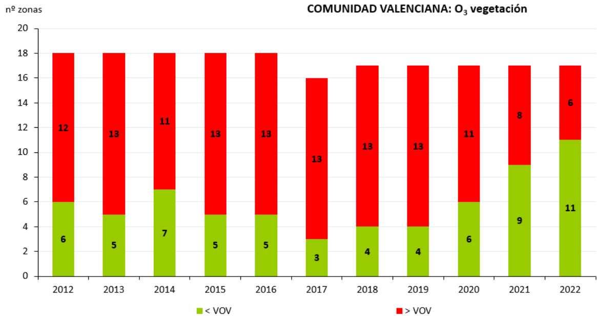
Figura 162. Evolución de las zonas de calidad del aire respecto al VO-Vegetación de O 3 (2012-2022)
