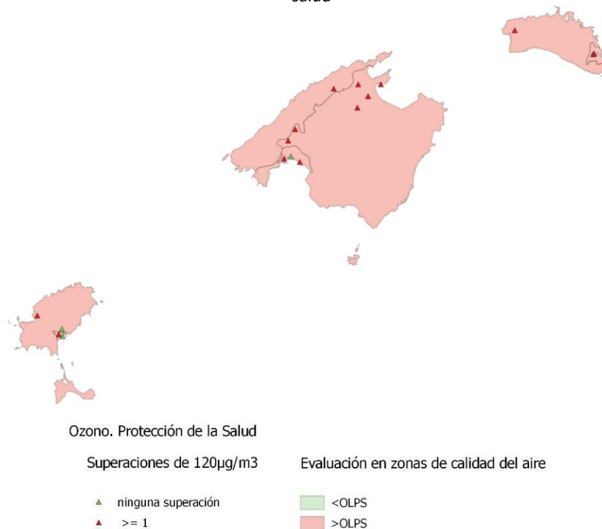
Figura 91. Número de superaciones en estaciones y evaluación por zonas del OLP de O 3 para la protección de la salud
