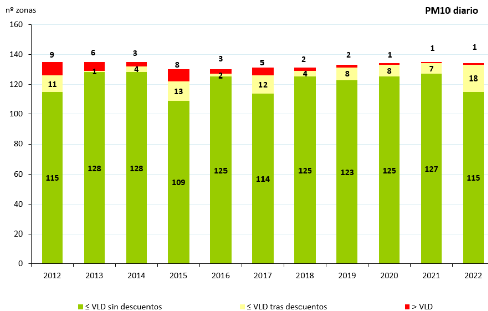
Figura 10. Evolución de las zonas de calidad del aire respecto al VLD de PM10 (2012-2022)
