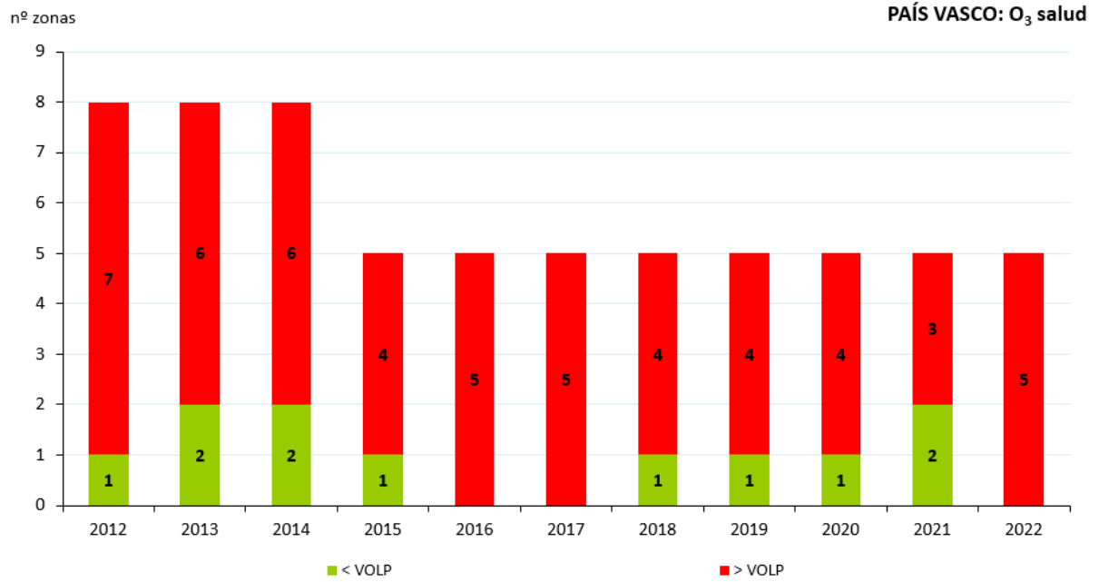
Figura 248. Evolución de las zonas respecto al OLP de ozono para protección de la salud (2012-2022)
