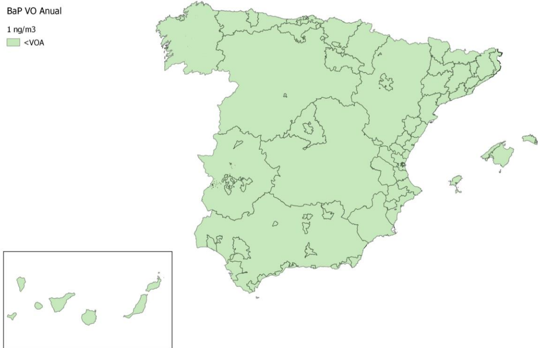
Figura 28. Situación de la calidad del aire de 2022 respecto al VO de B(a)P
