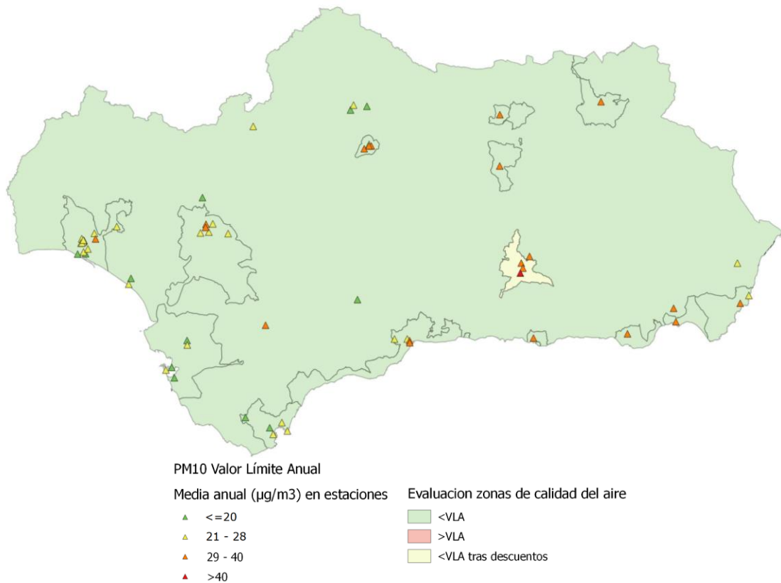
Figura 45. Media anual en estaciones y evaluación por zonas del VLA de PM10
