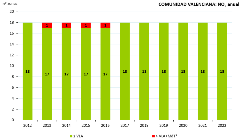
Figura 160. Evolución de las zonas de calidad del aire respecto al VLA de NO 2 (2012-2022)
