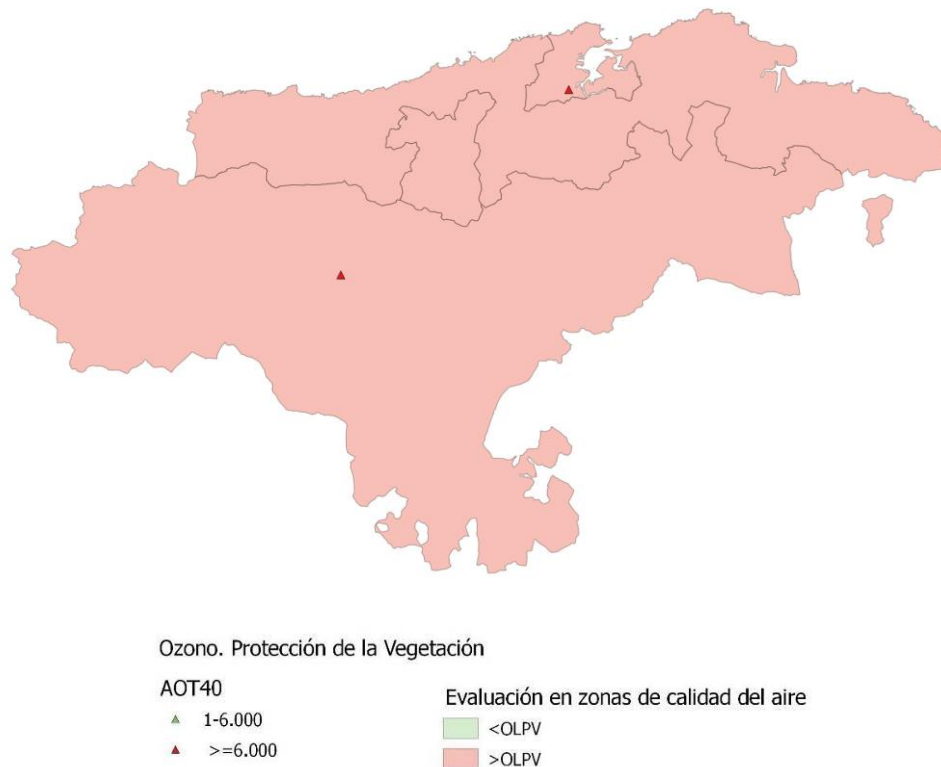
Figura 112. Número de superaciones en estaciones y evaluación por zonas del VO de O 3 para la protección de la vegetación
