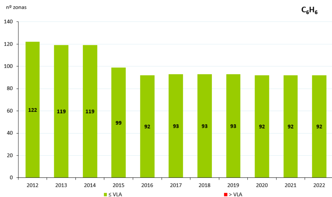
Figura 35. Evolución de las zonas de calidad del aire respecto al VL de C 6 H 6 (2012-2022)
