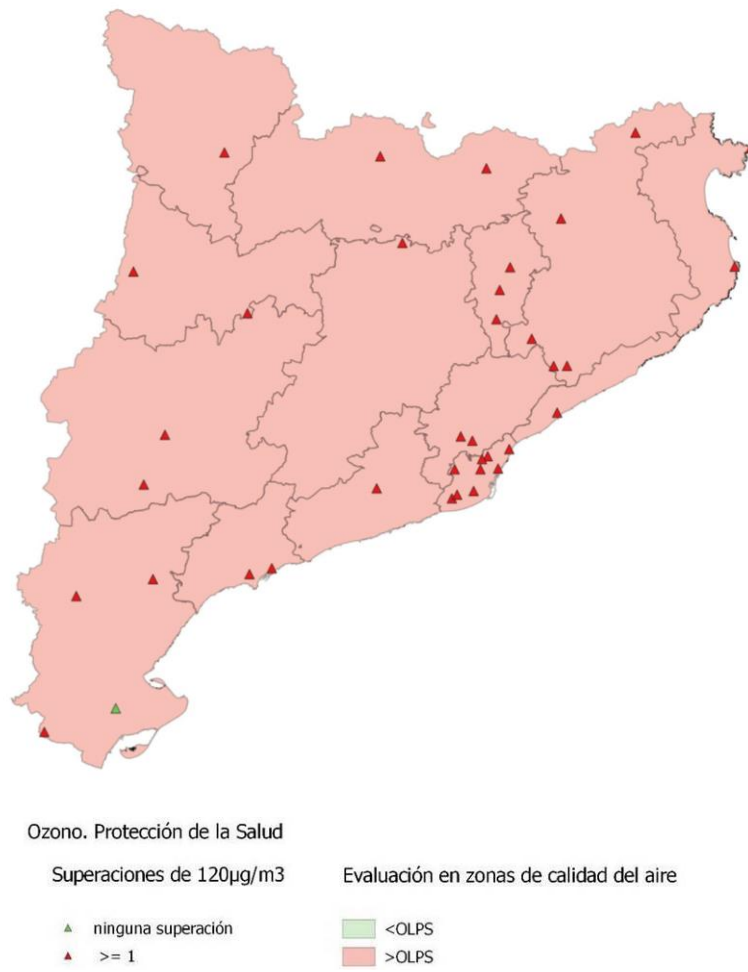
Figura 141. Número de superaciones en estaciones y evaluación por zonas del OLP de \text{O}_3 para la protección de la salud
