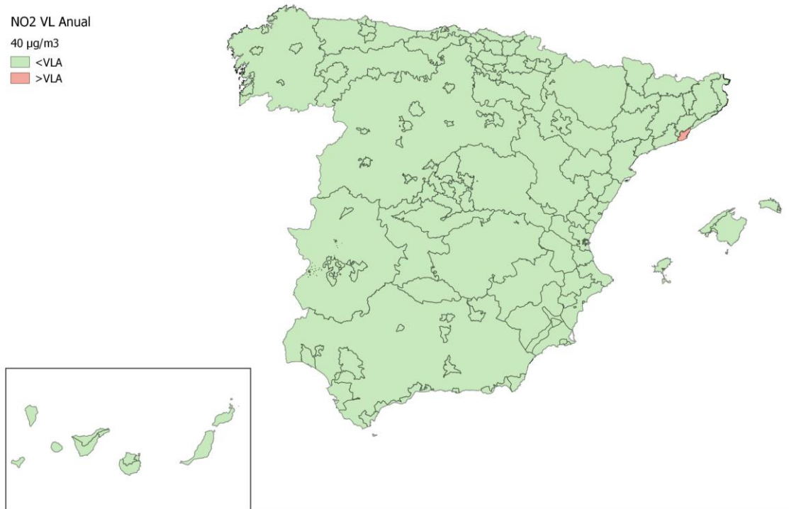
Figura 7. Situación de la calidad del aire de 2022 respecto al VLA de NO 2
