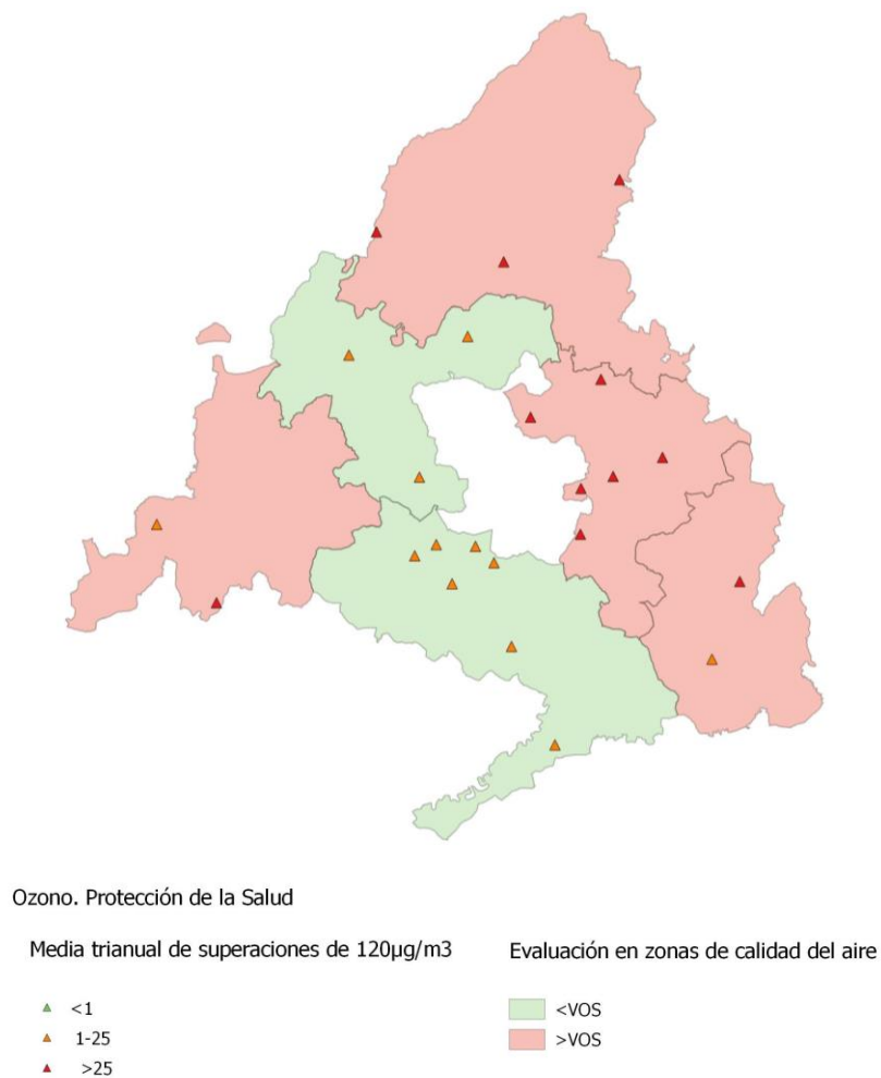
Figura 191. Número de superaciones en estaciones y evaluación por zonas del VO de O 3 para la protección de la salud
