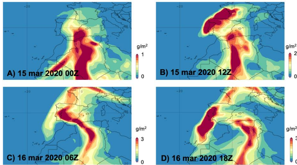
Figura 277. Evolución de la carga de polvo en columna durante los días 15, 16 y 17 de marzo 2022. modelo MERRA-2
