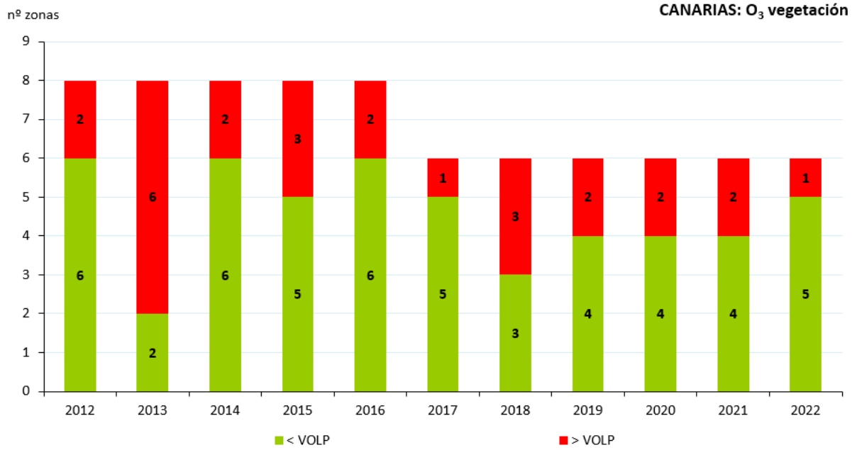
Figura 105. Evolución de las zonas respecto al OLP de ozono para protección de la vegetación (2012-2022)
