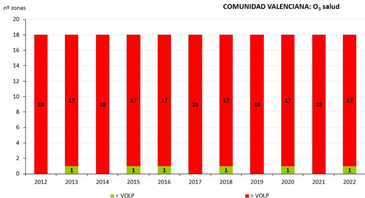
Figura 163. Evolución de las zonas respecto al OLP de ozono para protección de la salud (2012-2022)
