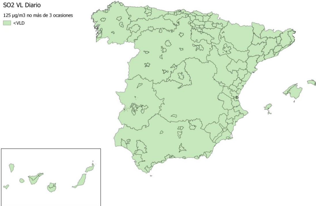
Figura 26. Situación de la calidad del aire de 2022 respecto al VLD de SO 2
