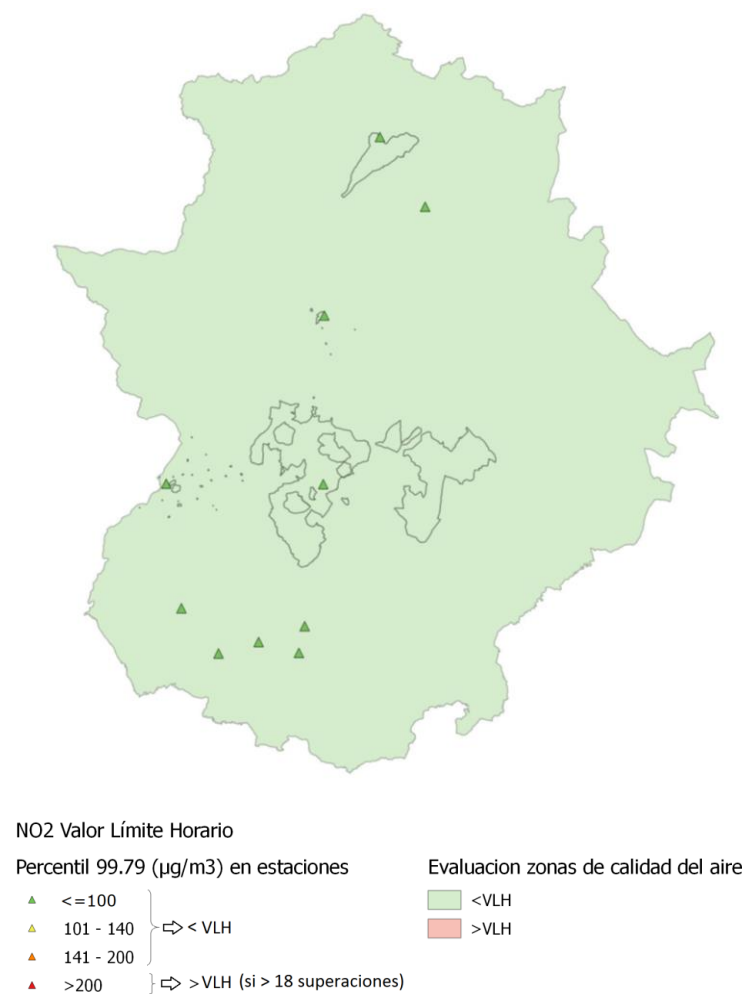
Figura 165. Percentil 99,79 en estaciones y evaluación por zonas del VLH de NO 2
