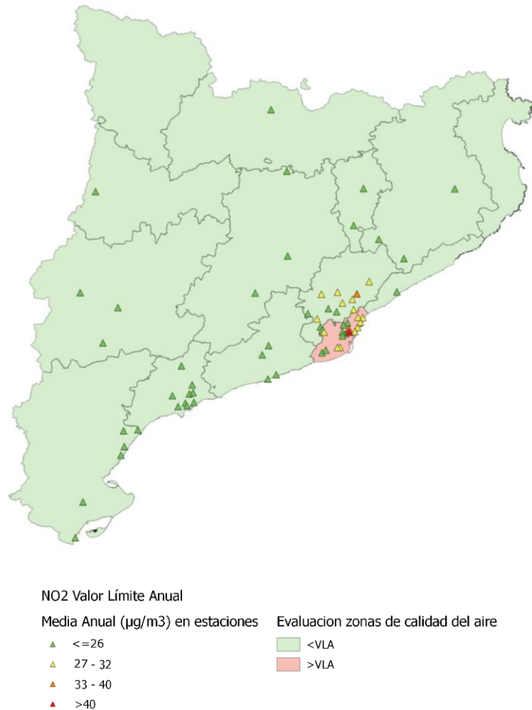
Figura 137. Media anual en estaciones y evaluación por zonas del VLA de NO 2
