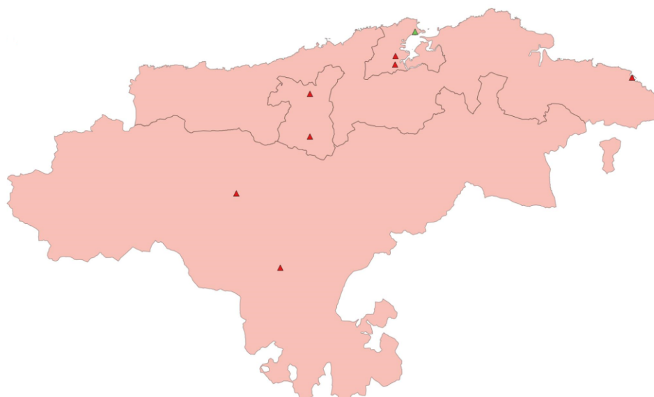
Figura 110. Número de superaciones en estaciones y evaluación por zonas del VO de \text{O}_3 para la protección de la salud
