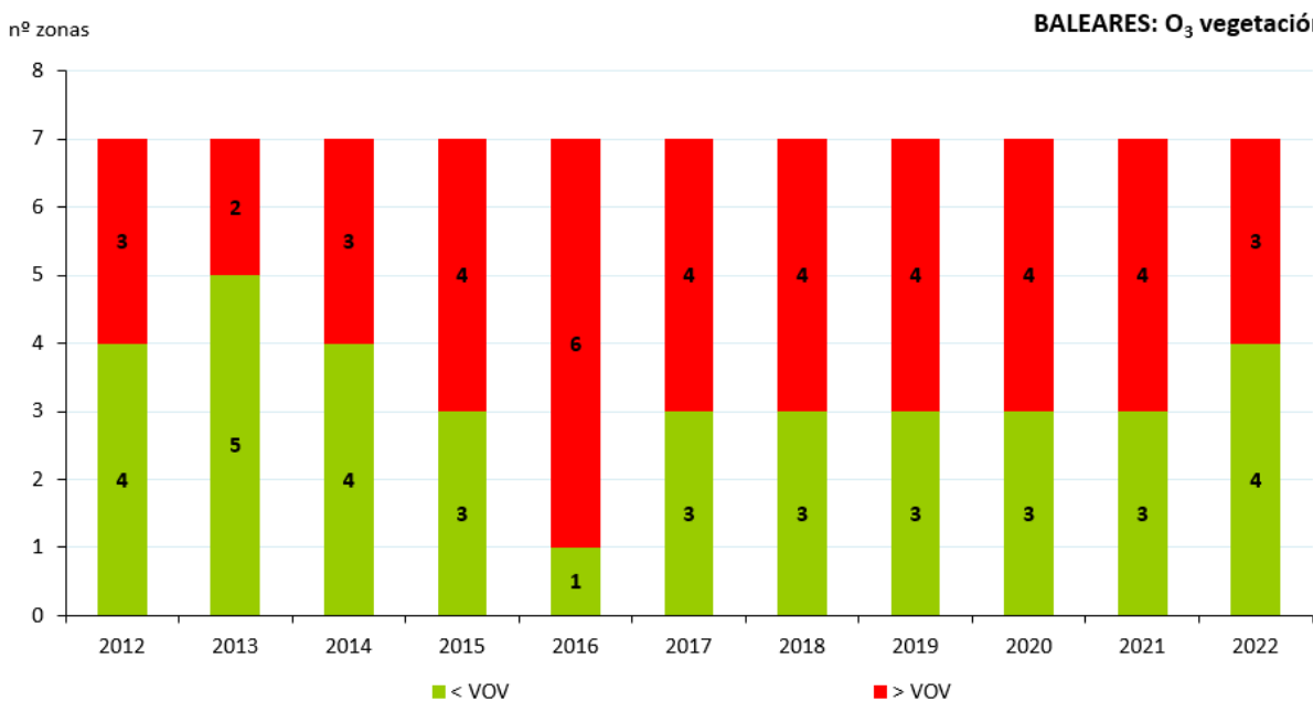
Figura 95. Evolución de las zonas de calidad del aire respecto al VO-Vegetación de O 3 (2012-2022)
