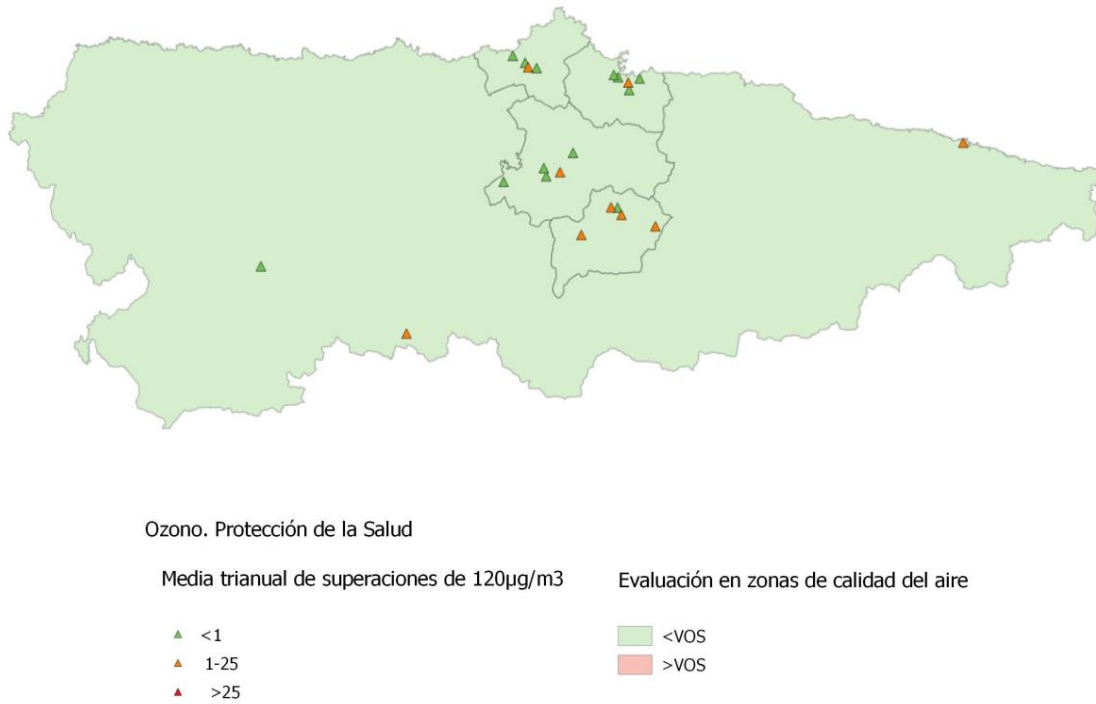
Figura 78. Número de superaciones en estaciones y evaluación por zonas del VO de O 3 para la protección de la salud
