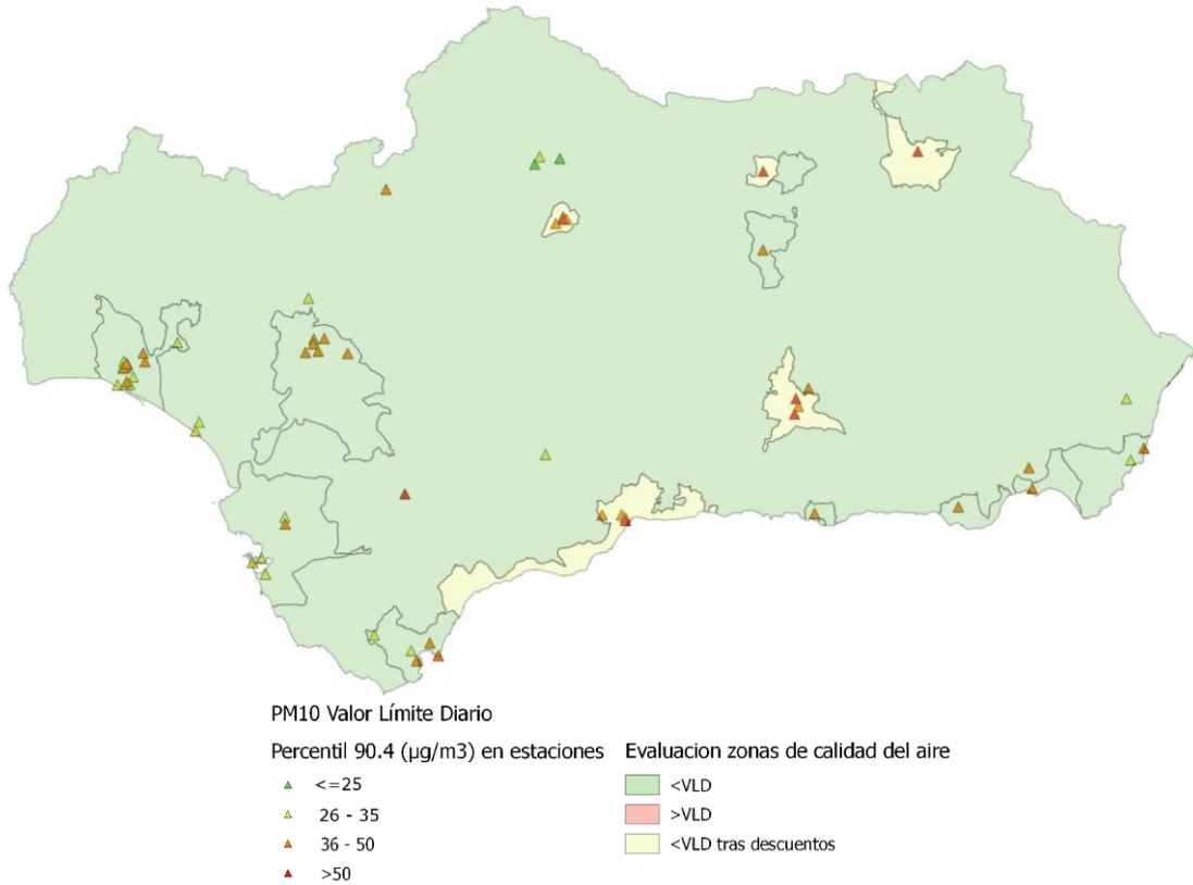
Figura 44. Percentil 90,4 en estaciones y evaluación por zonas de VLD de PM10
