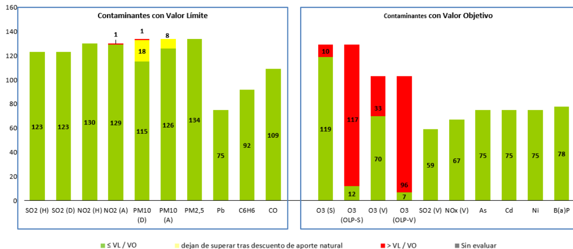
Figura 1. Resumen de la evaluación de la calidad del aire en 2022 por contaminante
