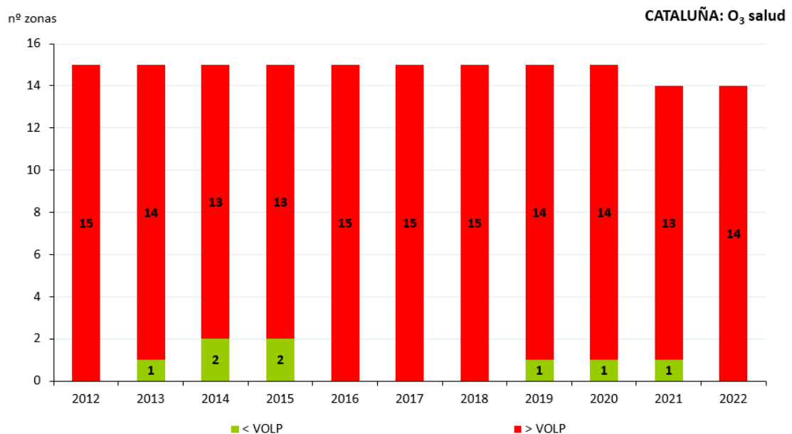
Figura 149. Evolución de las zonas respecto al OLP de ozono para protección de la salud (2012-2022)
