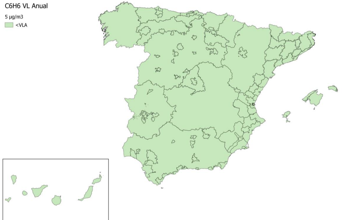
Figura 34. Situación de la calidad del aire de 2022 respecto del VL de C 6 H 6
