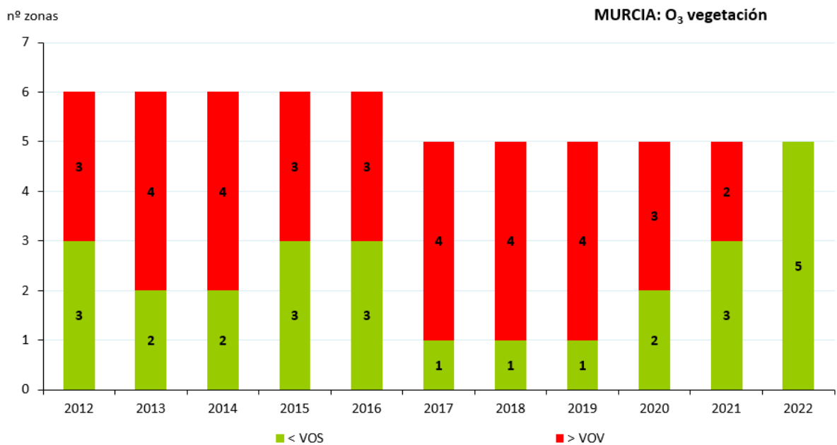
Figura 221. Evolución de las zonas de calidad del aire respecto al VO-Vegetación de O 3 (2012-2022)
