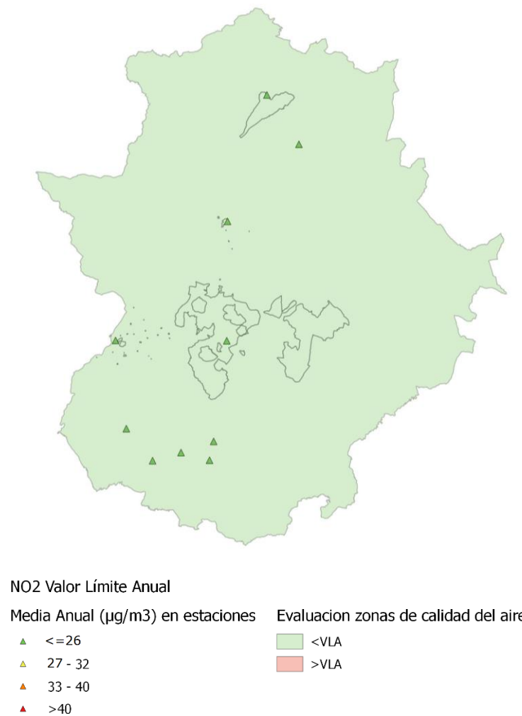
Figura 166. Media anual en estaciones y evaluación por zonas del VLA de NO 2
