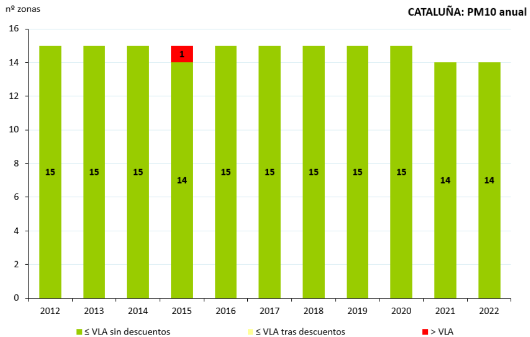
Figura 146. Evolución de las zonas de calidad del aire respecto al VLA de PM10 (2012-2022)
