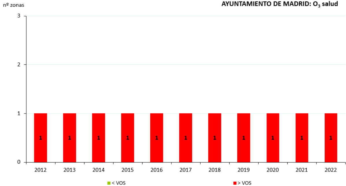
Figura 209. Evolución de las zonas de calidad del aire respecto al VO-Salud de O 3 (2012-2022)
