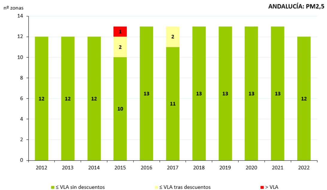
Figura 52. Evolución de las zonas de calidad del aire respecto al VLA de PM2,5 (2012-2022)
