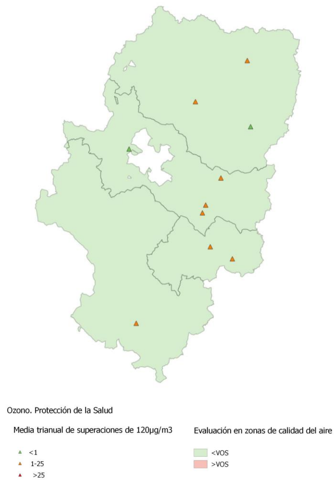
Figura 61. Número de superaciones en estaciones y evaluación por zonas del VO de O 3 para la protección de la salud
