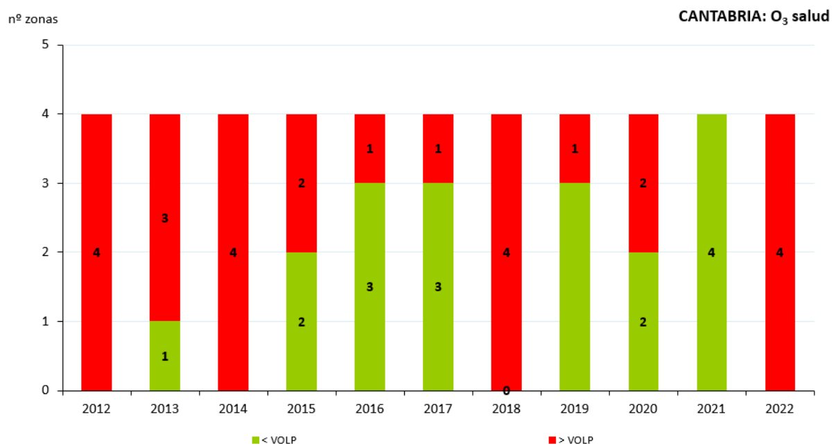
Figura 114. Evolución de las zonas respecto al OLP de ozono para protección de la salud (2012-2022)
