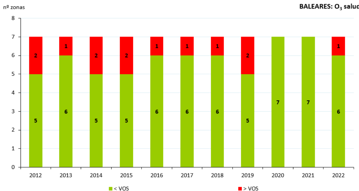
Figura 94. Evolución de las zonas de calidad del aire respecto al VO-Salud de O 3 (2012-2022)
