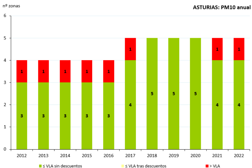
Figura 83. Evolución de las zonas respecto al VLA de PM10 (2012-2022)
