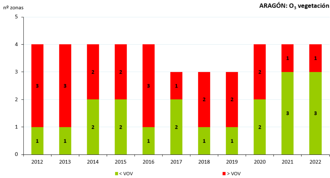
Figura 66. Evolución de las zonas de calidad del aire respecto al VO-Vegetación de O 3 (2012-2022)
