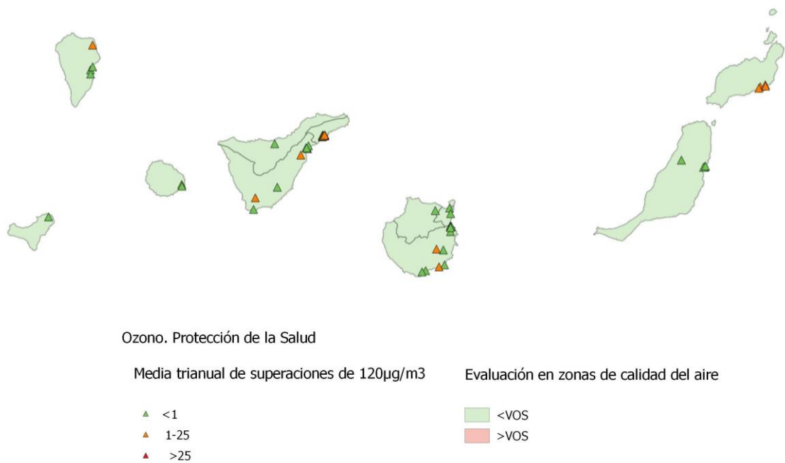
Figura 100. Número de superaciones en estaciones y evaluación por zonas del VO de O 3 para la protección de la salud
