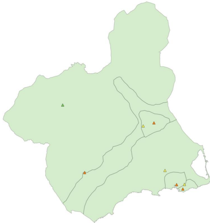
Figura 213. Percentil 90,4 en estaciones y evaluación por zonas del VLD de PM10 no se supera ni siquiera
