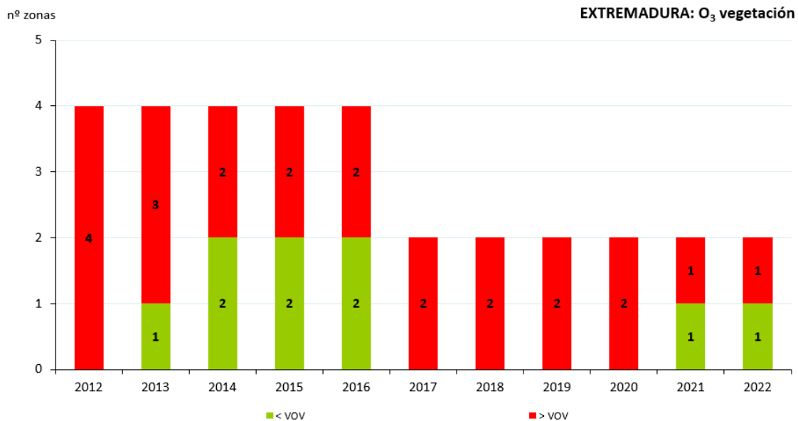
Figura 174. Evolución de las zonas de calidad del aire respecto al VO-Vegetación de O 3 (2012-2022)
