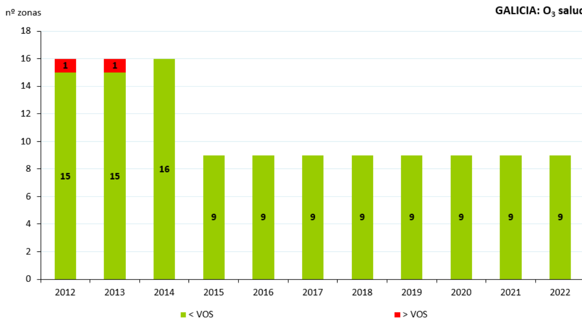
Figura 184. Evolución de las zonas de calidad del aire respecto al VO-Salud de O 3 (2012-2022)
