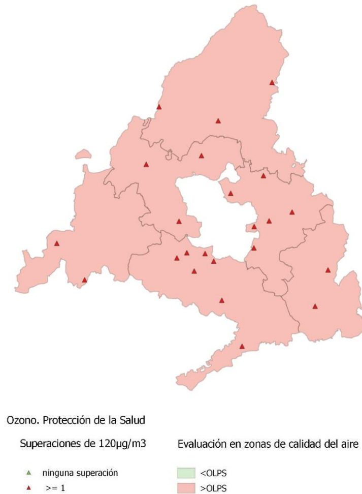
Figura 192. Número de superaciones en estaciones y evaluación por zonas del OLP de O 3 para la protección de la salud
