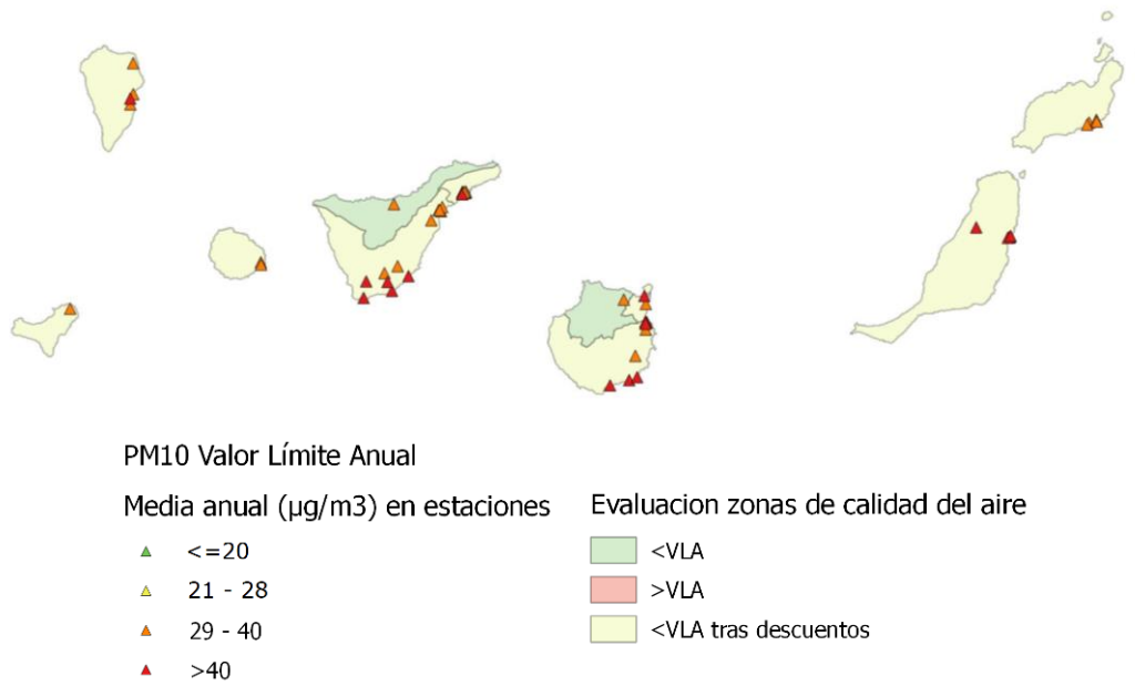
Figura 99. Media anual en estaciones y evaluación por zonas del VLA de PM10
