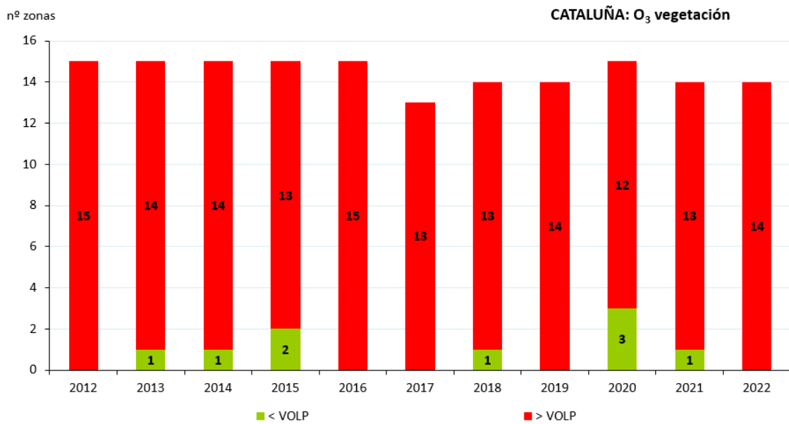
Figura 150. Evolución de las zonas respecto al OLP de ozono para protección de la vegetación (2012-2022)
