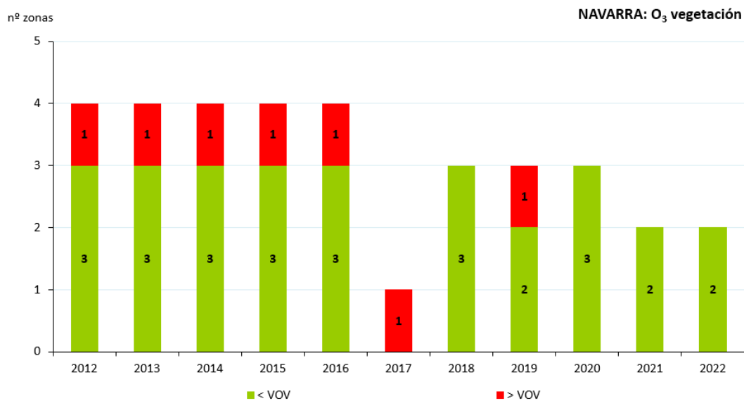
Figura 233. Evolución de las zonas de calidad del aire respecto al VO-Vegetación de O 3 (2012-2022)
