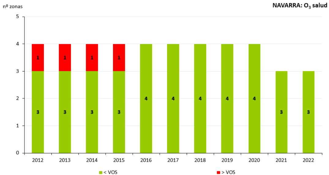
Figura 232. Evolución de las zonas de calidad del aire respecto al VO-Salud de O 3 (2012-2022)
