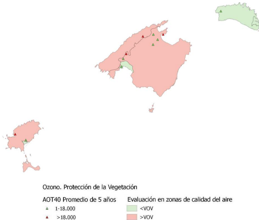
Figura 92. Número de superaciones en estaciones y evaluación por zonas del VO de O 3 para la protección de la vegetación
