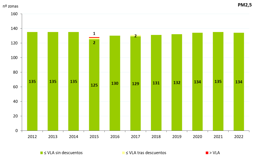
Figura 14. Evolución de las zonas de calidad del aire respecto al VLA de PM 2,5 (2012-2022)
