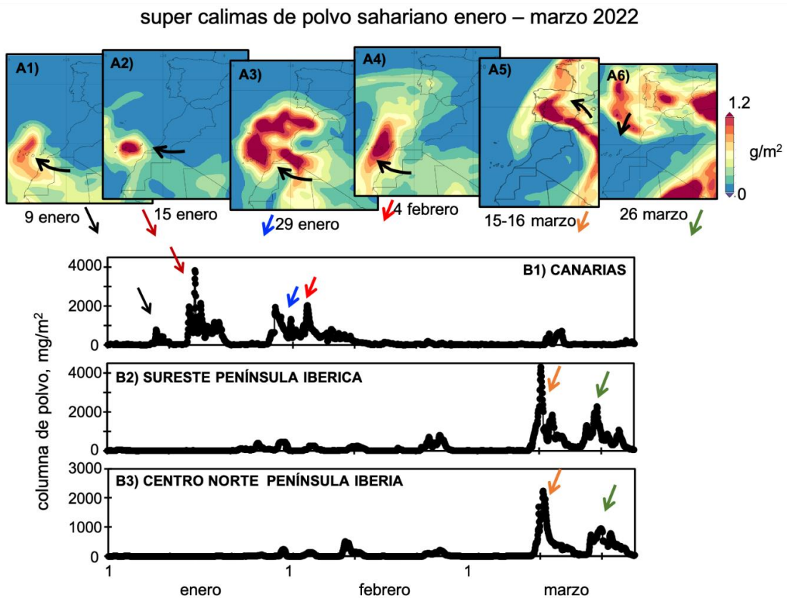
Figura 274. Super calimas de polvo sahariano de enero y marzo 2022. A1-A6) Carga de polvo en la columna atmosférica (miligramos de polvo / m 2 de superficie terrestre), donde el valor máximo corresponde a 7.0, 3.0, 2.0, 1.5, 3.0 y 1.5 g/m 2 , en A1, A2, A3, A4, A5, y A6, respectivamente. B1-B3) serie temporal de carga de polvo en Canarias (B1), el sureste península ibérica (B2: Granada, Almería y Murcia) y el centro norte peninsular (B3: Castilla y León). Datos obtenidos mediante re-análisis con el modelo MERRA-2 57
