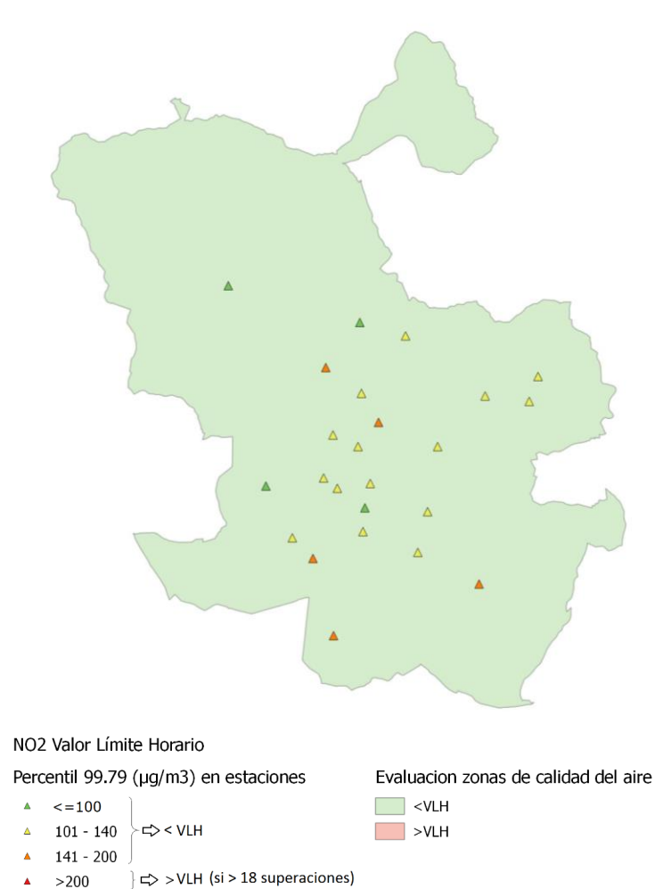
Figura 199. Percentil 99,79 en estaciones y evaluación por zonas del VLH de \text{NO}_2
