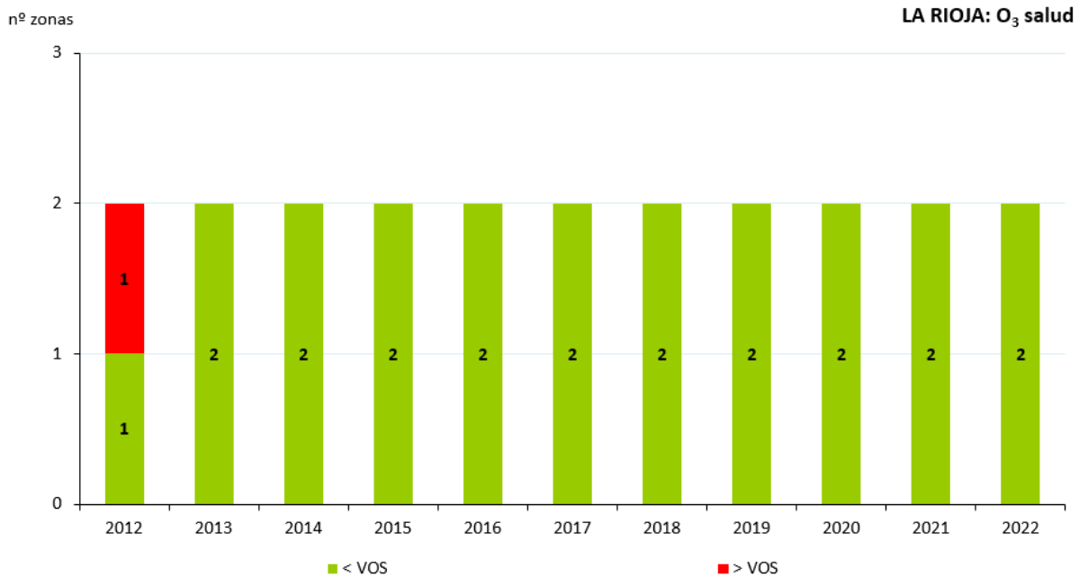
Figura 258. Evolución de las zonas de calidad del aire respecto al VO-Salud de O 3 (2012-2022)
