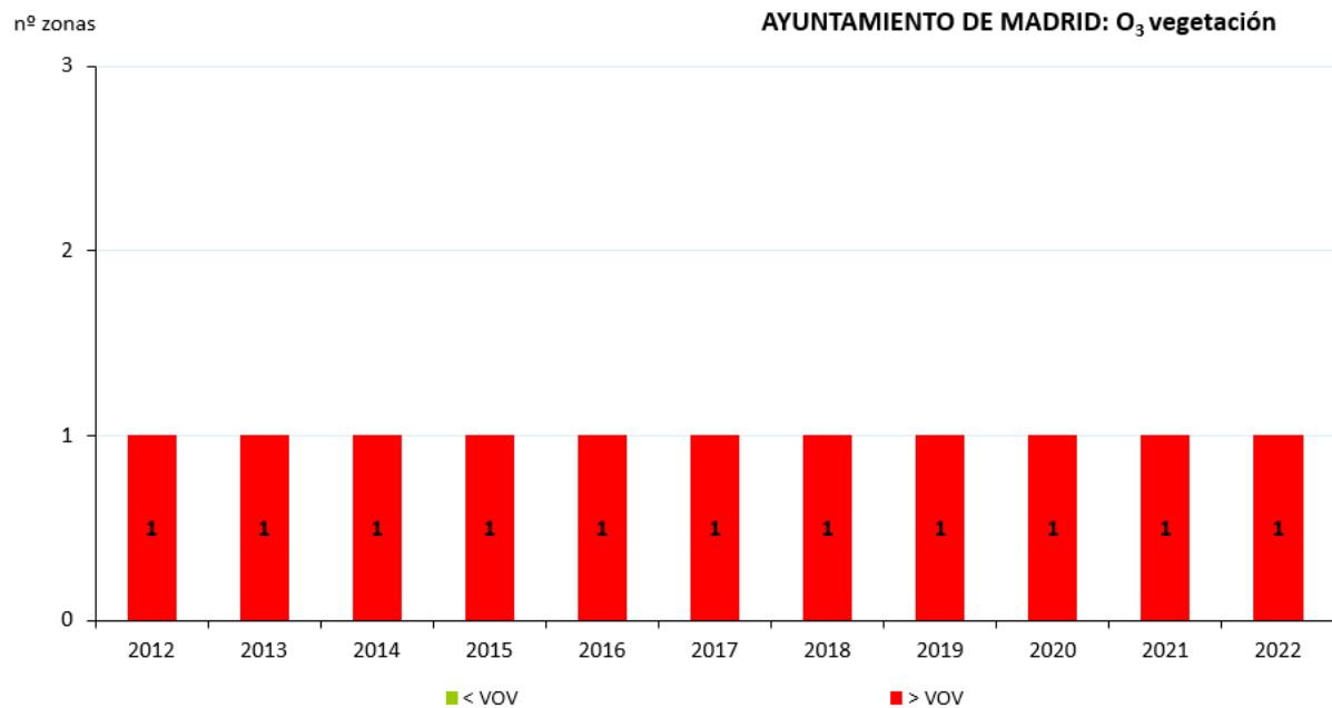
Figura 210. Evolución de las zonas de calidad del aire respecto al VO-Vegetación de O 3 (2012-2022)
