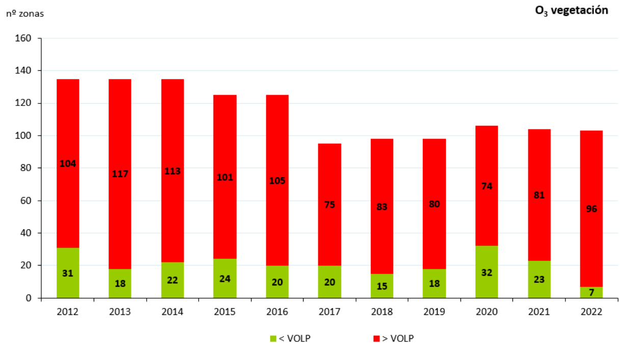
Figura 23. Evolución de las zonas respecto al OLP-vegetación de O 3 (2012-2022)
