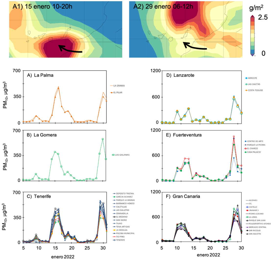
Figura 276. Carga de polvo (A1-A2) sobre Canarias (modelo MERRA-2) y series temporales de promedios diario (24h) de concentraciones de PM 10 evaluadas y reconstruidas mediante duxt-r 57
