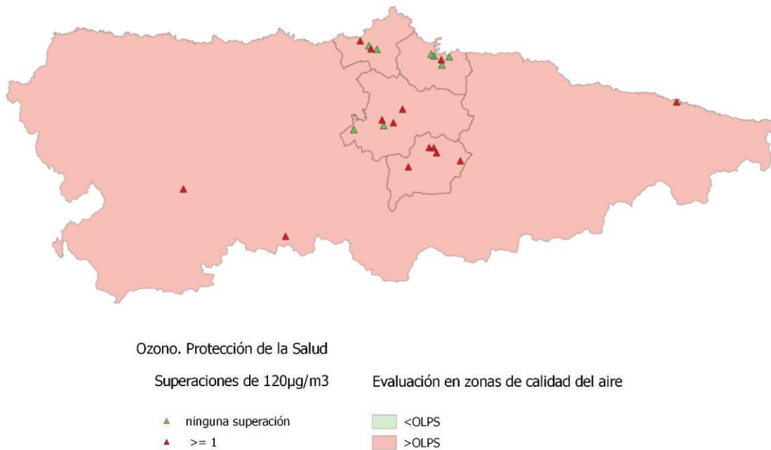
Figura 79. Número de superaciones en estaciones y evaluación por zonas del OLP de O 3 para la protección de la salud
