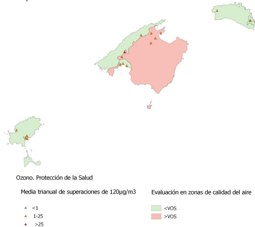
Figura 90. Número de superaciones en estaciones y evaluación por zonas del VO de O 3 para la protección de la salud
