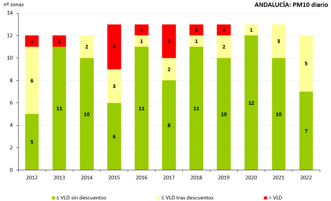
Figura 51. Evolución de las zonas de calidad del aire respecto al VLD de PM10 (2012-2022)
