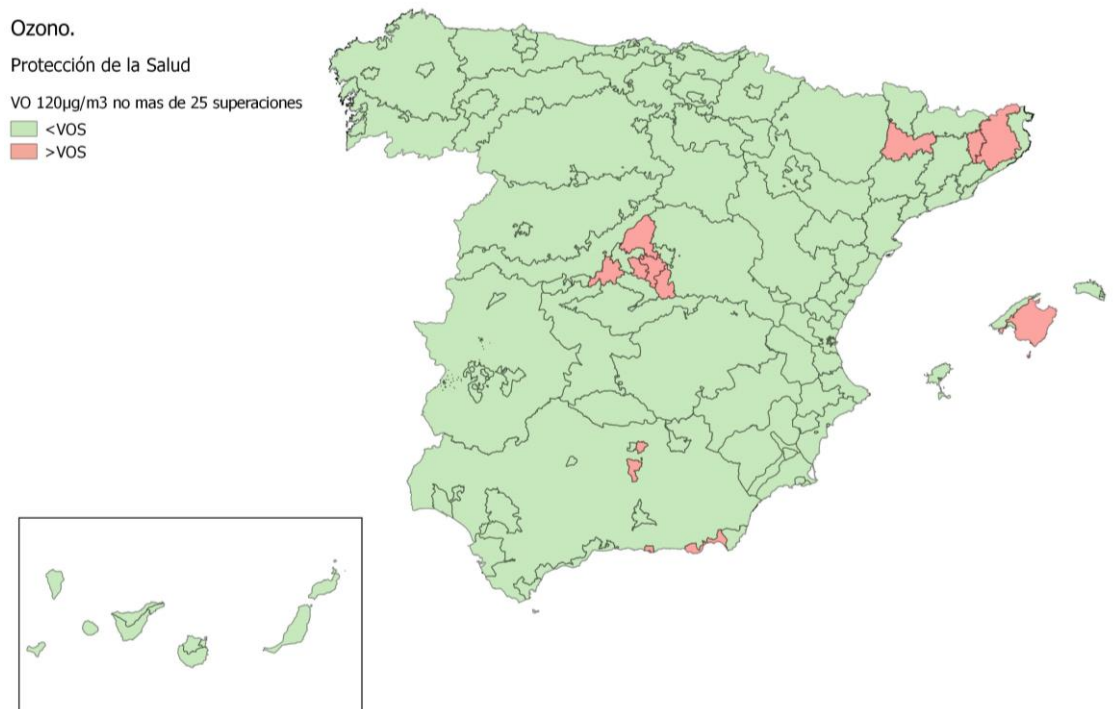
Figura 16. Situación de la calidad del aire de 2022 respecto al VO de O 3 para la protección de la salud
