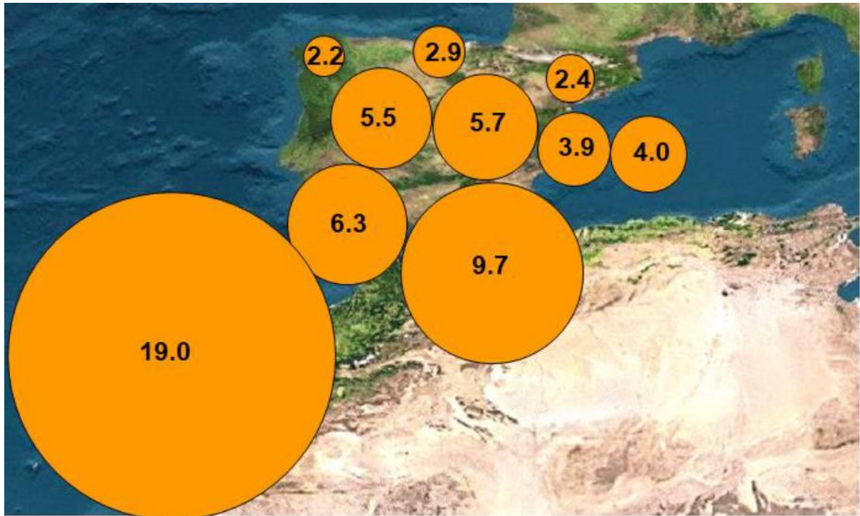
Figura 4. Contribución de polvo africano a PM10 en 2022 (fuente: CSIC)
