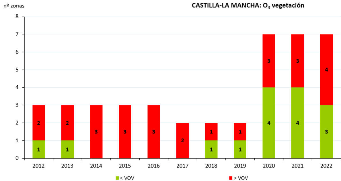
Figura 125. Evolución de las zonas de calidad del aire respecto al VO-Vegetación de O 3 (2012-2022)
