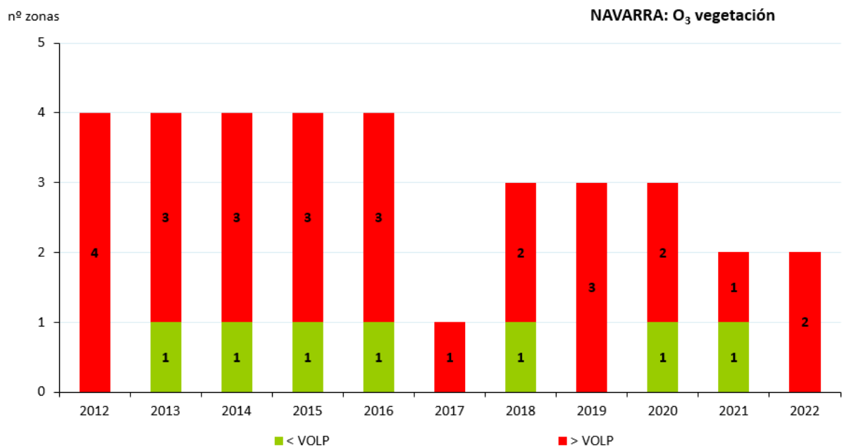
Figura 235. Evolución de las zonas respecto al OLP de ozono para protección de la vegetación (2012-2022)
