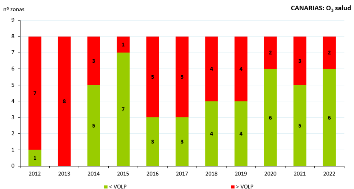
Figura 104. Evolución de las zonas respecto al OLP de ozono para protección de la salud (2012-2022)
