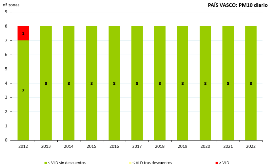
Figura 245. Evolución de las zonas de calidad del aire respecto al VLD de PM10 (2012-2022)
