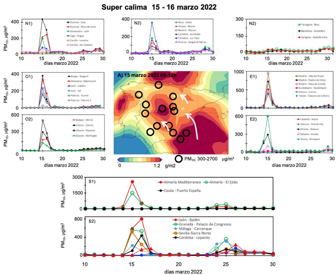
Figura 278. Polvo en columna el 15 de marzo 2022 (promedio 08-12 GTM) mostrando con círculo negro las ubicaciones donde se superaron los 300 \mu\text{g}/\text{m}^3 de \text{PM}_{10} como media diaria. Serie de concentración media diaria de \text{PM}_{10} entre el 10 y 30 de marzo 2022 en la península, en base a datos evaluados y reconstruidos mediante el método duxt-r.
