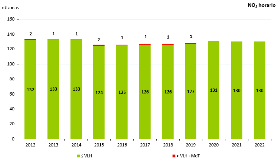
Figura 6. Evolución de las zonas de calidad del aire respecto al VLH de NO 2 (2012-2022)
