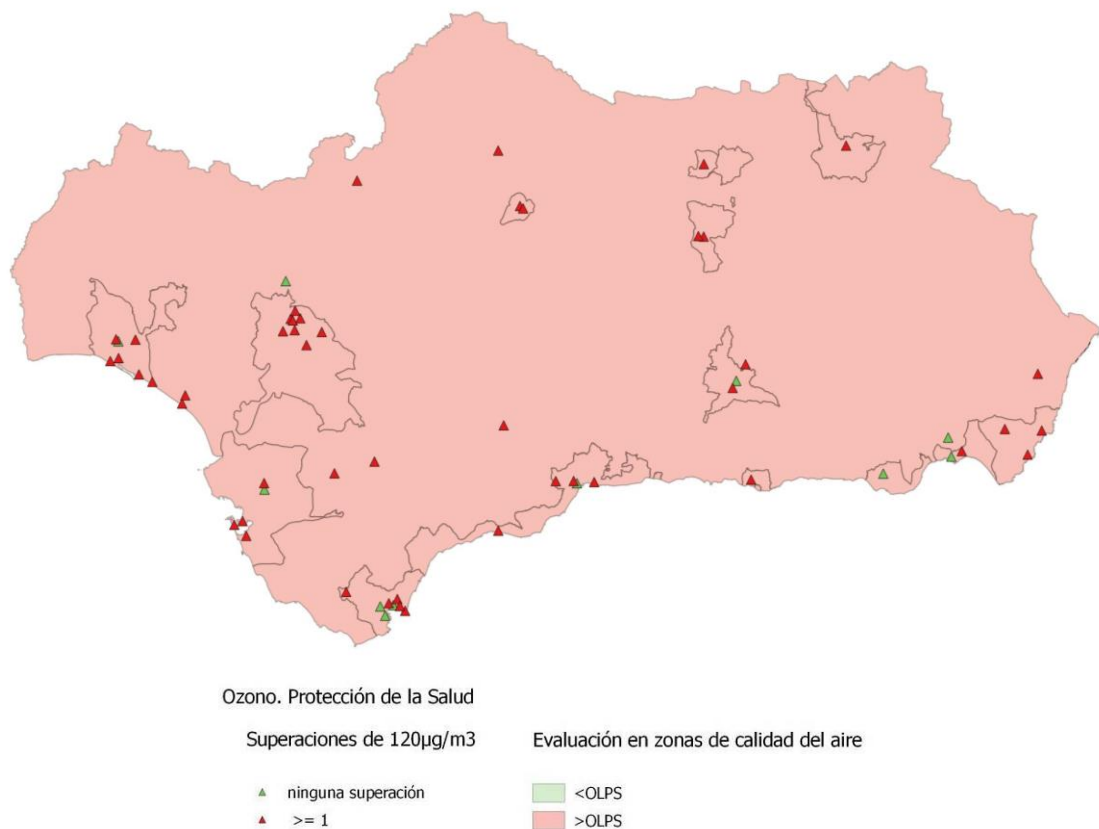
Figura 47. Número de superaciones en estaciones y evaluación por zonas del OLP de \text{O}_3 para la protección de la salud
