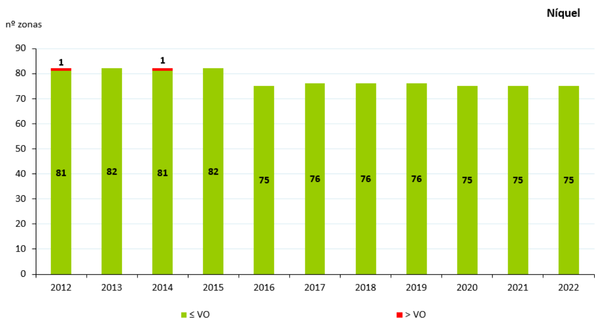
Figura 41. Evolución de las zonas de calidad del aire respecto al VO de Ni (2012-2022)
