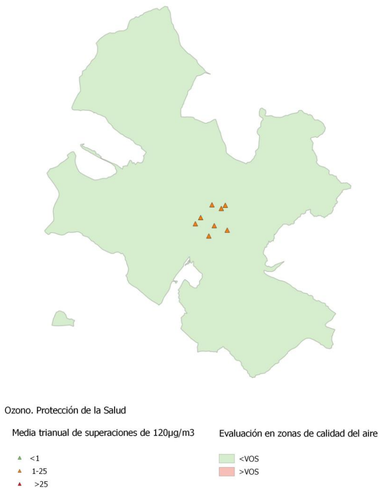
Figura 71. Número de superaciones en estaciones y evaluación por zonas del VO de O 3 para la protección de la salud
