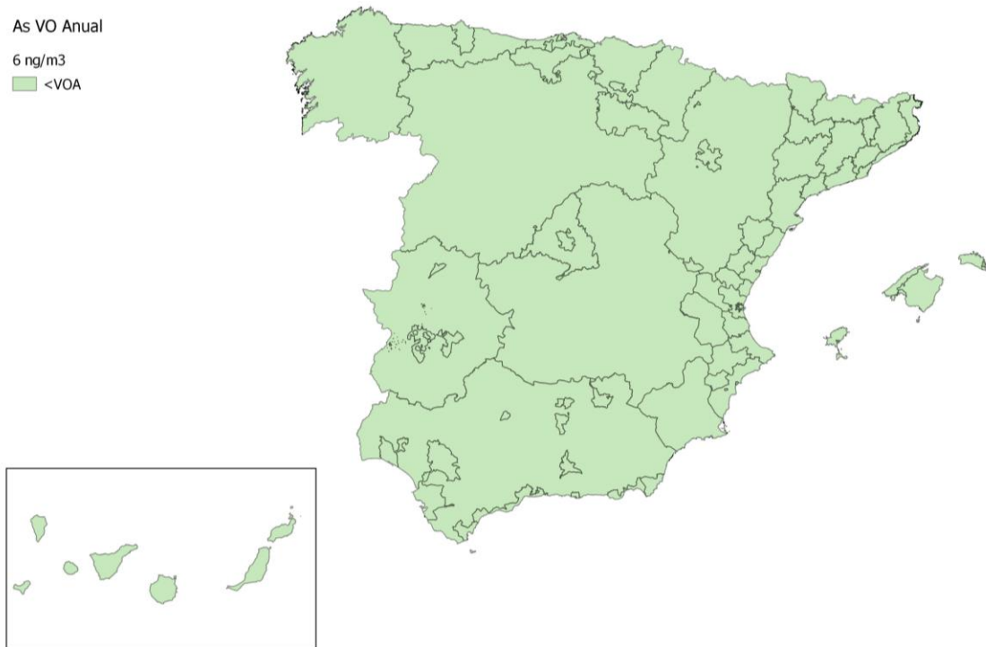
Figura 36. Situación de la calidad del aire de 2022 respecto del VO de As
