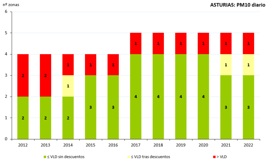
Figura 82. Evolución de las zonas respecto al VLD de PM10 (2012-2022)
