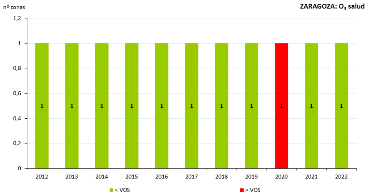
Figura 73. Evolución de las zonas de calidad del aire respecto al VO-Salud de O 3 (2012-2022)
