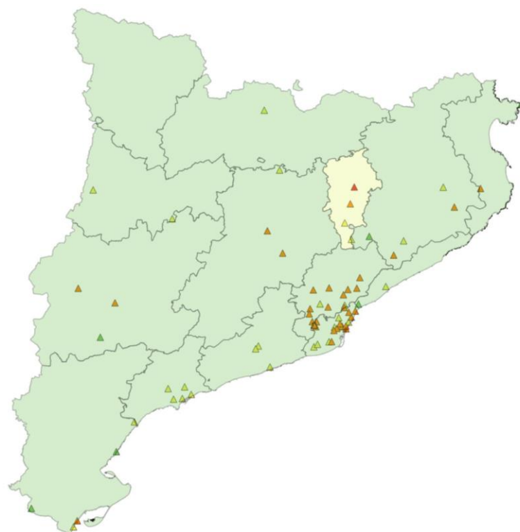
PM10 Valor Límite Diario
