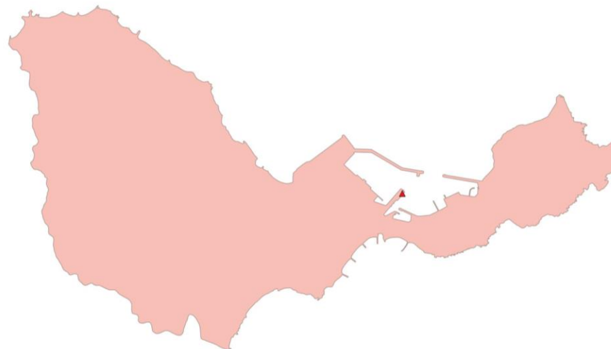
Figura 265. Número de superaciones en estaciones y evaluación por zonas del VO de O 3 para la protección de la salud
