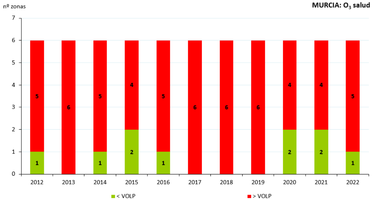
Figura 222. Evolución de las zonas respecto al OLP de ozono para protección de la salud (2012-2022)
