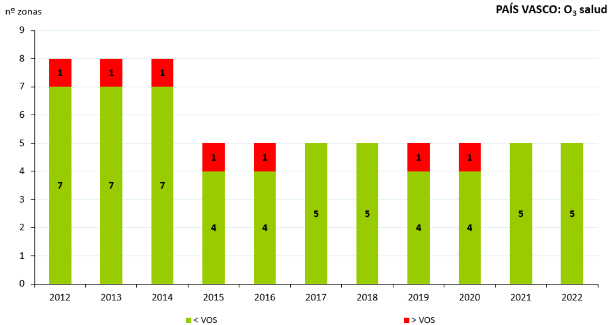
Figura 246. Evolución de las zonas de calidad del aire respecto al VO-Salud de O 3 (2012-2022)
