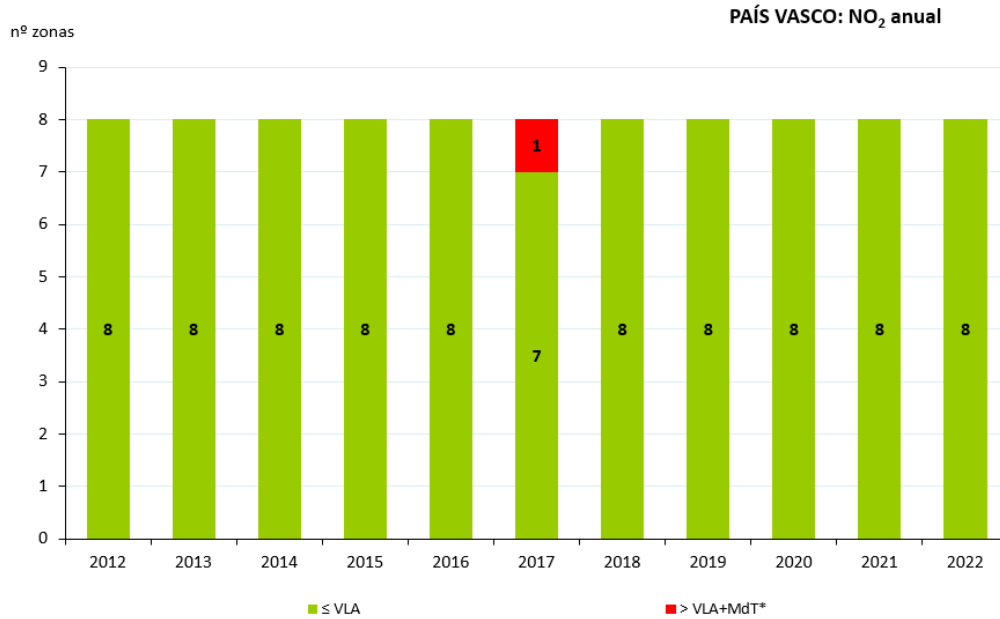
Figura 244. Evolución de las zonas de calidad del aire respecto al VLA de NO 2 (2012-2022)
