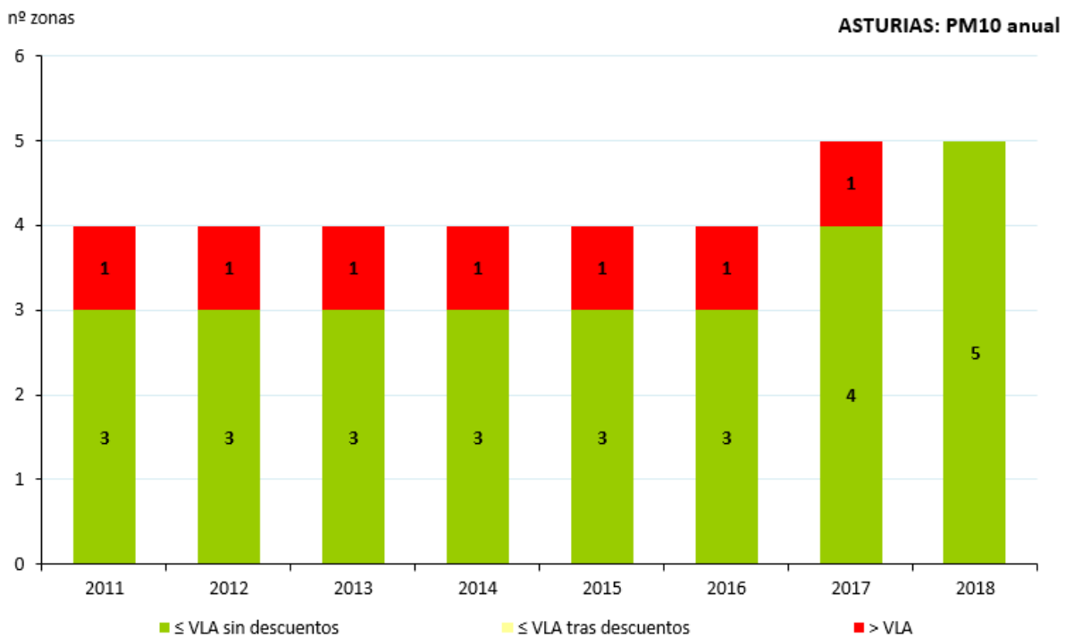
Figura 68. Evolución de las zonas respecto al VLA de PM10 (2011-2018)
