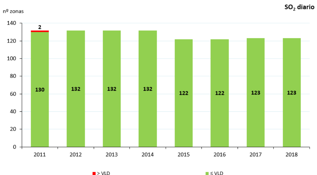
Figura 20. Situación respecto al VLD de SO 2 (2011-2018)
