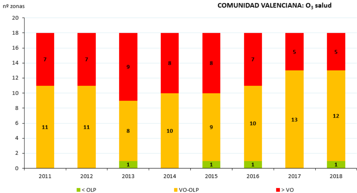
Figura 123. Situación respecto al VO-Salud de O 3 (2011-2018)
