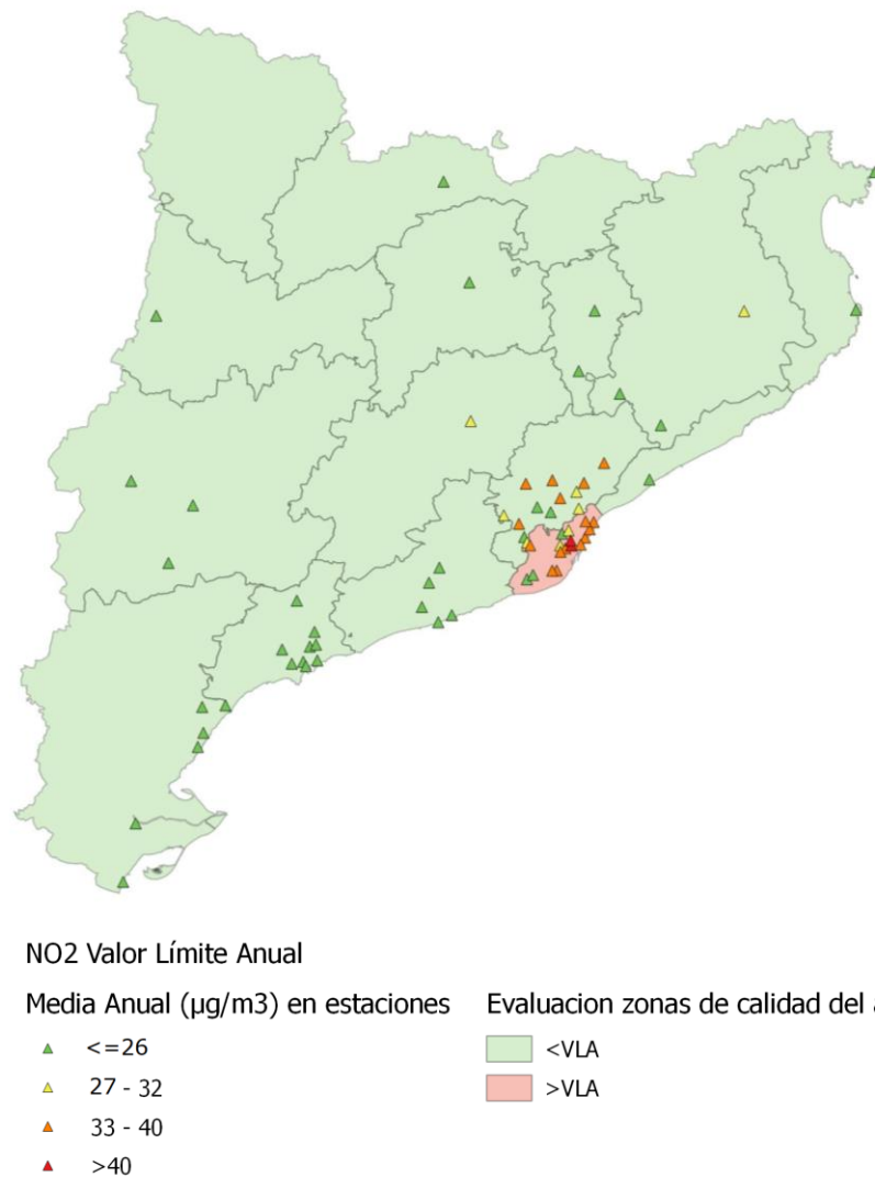
Figura 105. Media anual en estaciones y evaluación por zonas del VLA de NO 2
