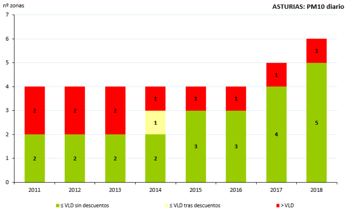
Figura 67. Evolución de las zonas respecto al VLD de PM10 (2011-2018)
