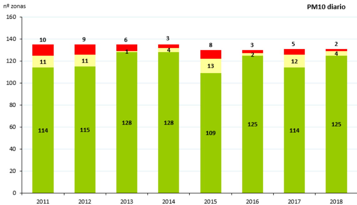
Figura 7. Situación respecto al VLD de PM10 (2011-2018)
