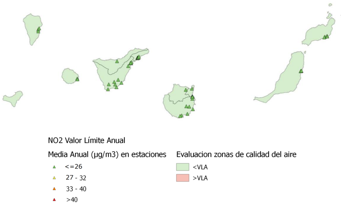
Figura 79. Media anual en estaciones y evaluación por zonas del VLA de NO 2
