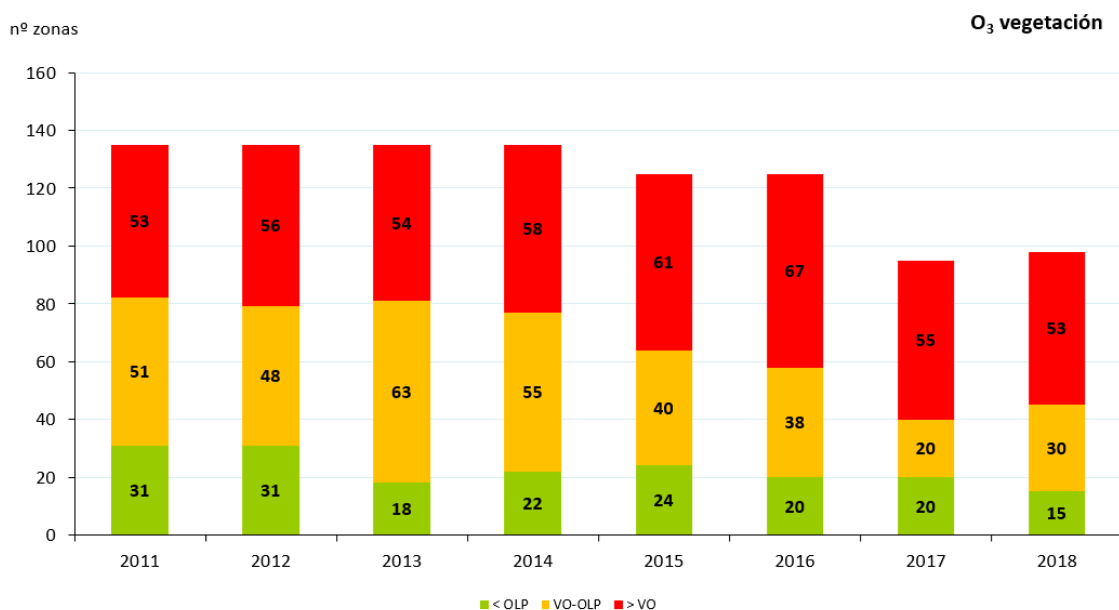
Figura 16. Evolución de las zonas respecto al VO-vegetación de O 3 (2011-2018)
