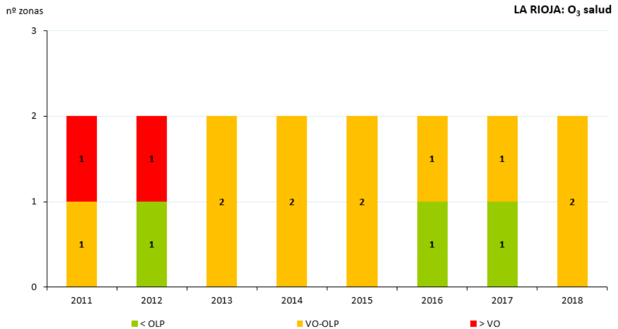
Figura 189. Situación respecto al VO-Salud de O 3 (2011-2018)
