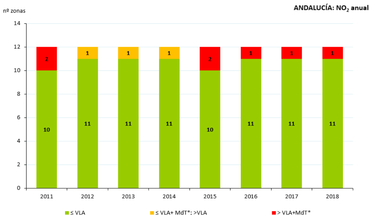
Figura 41. Situación respecto al VLA de NO 2 (2011-2018)
