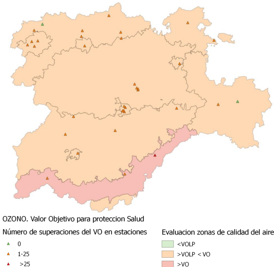
Figura 102. Número de superaciones en estaciones y evaluación por zonas del VO de \text{O}_3 para la protección de la salud
