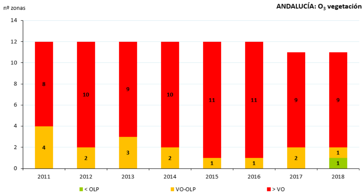
Figura 45. Situación respecto al VO-Vegetación de O 3 (2011-2018)
