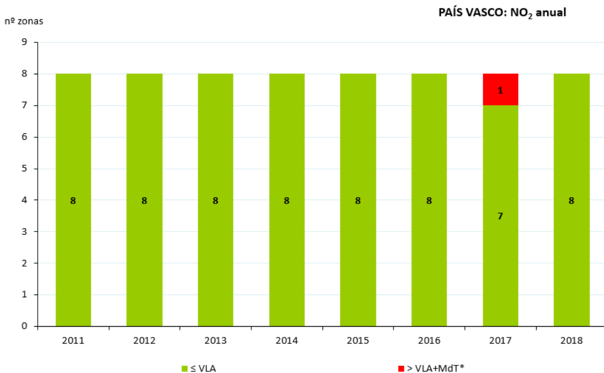
Figura 180. Situación respecto al VLA de NO 2 (2011-2018)
