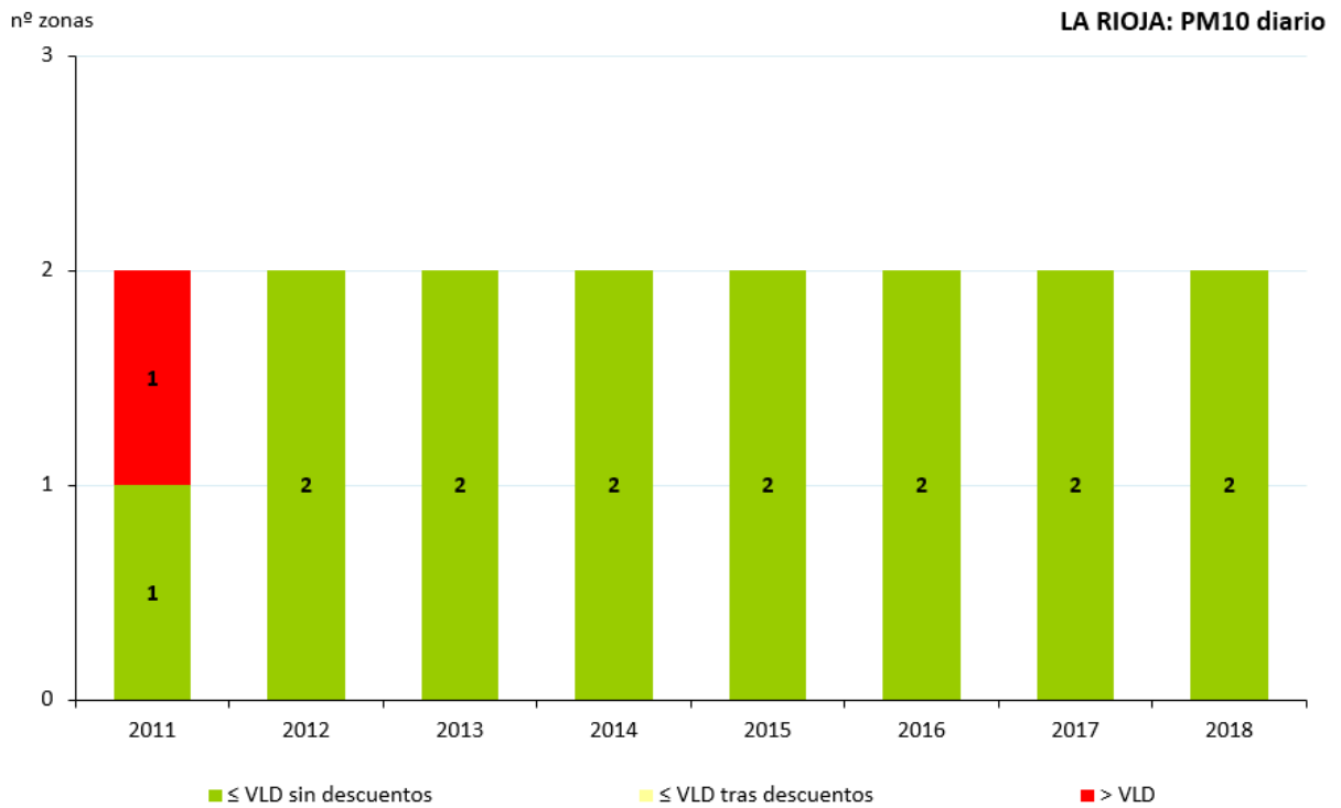
Figura 188. Situación respecto al VLD de PM10 (2011-2018)
