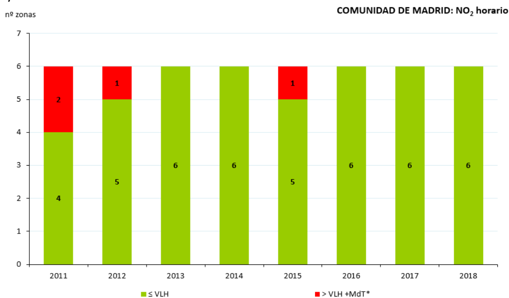
Figura 146. Situación respecto al VLH de NO 2 (2011-2018)
