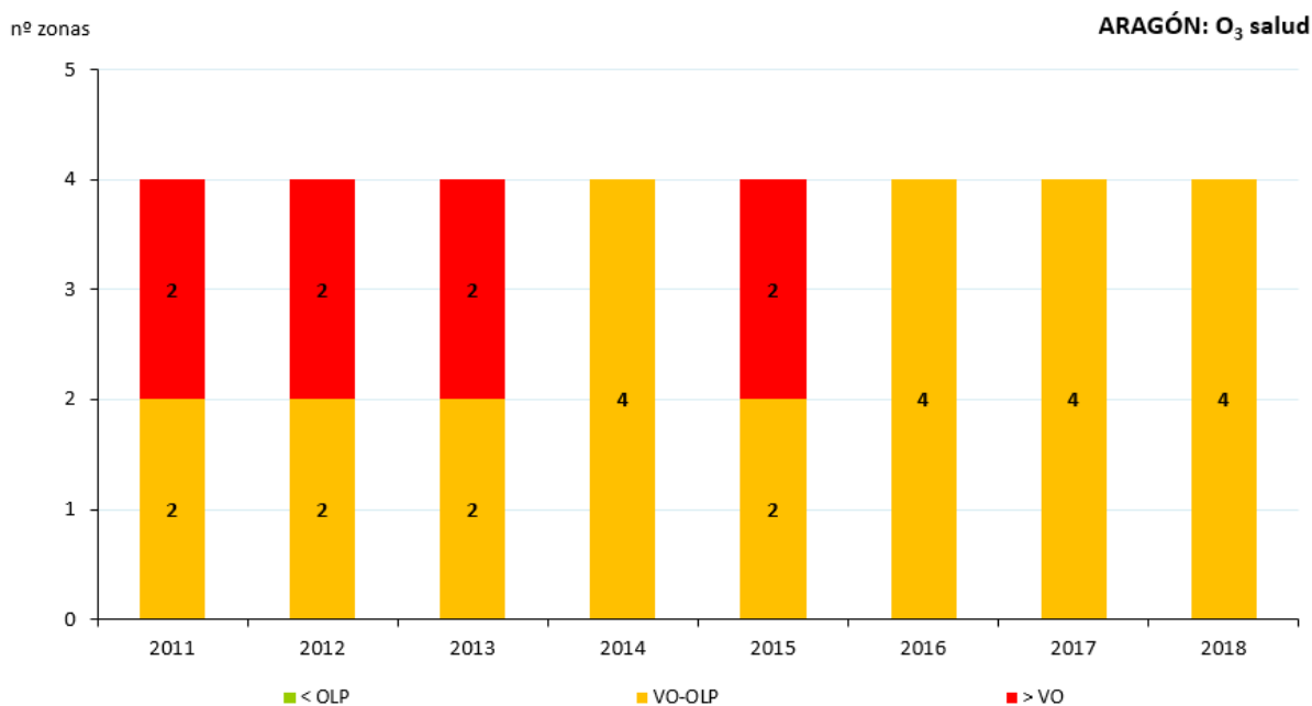
Figura 55. Situación respecto al VO-Salud de O 3 (2011-2018)
