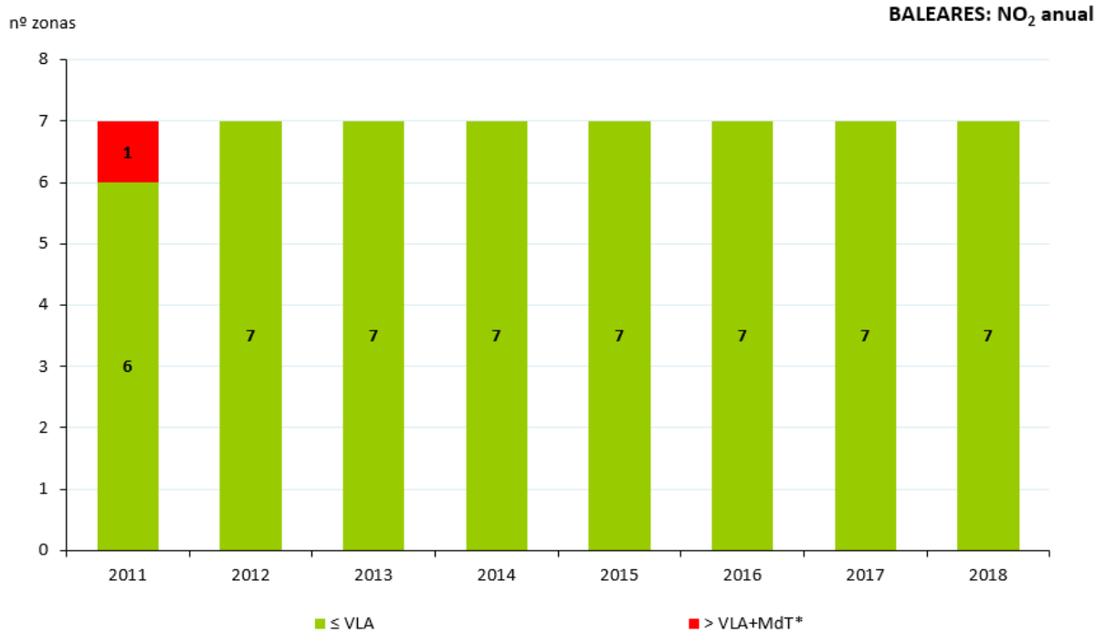
Figura 75. Situación respecto al VLA de NO 2 (2011-2018)
