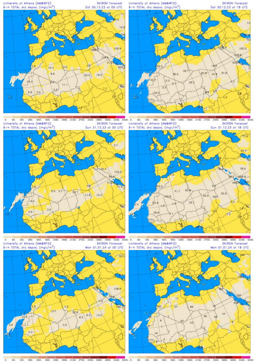
Depósito seco de polvo ( \text{mg}/\text{m}^2 ) predicho por el modelo SKIRON para los días 30 y 31 de diciembre de 2023 y 1 de enero de 2024 a las 00 y 18 UTC © Universidad de Atenas.
