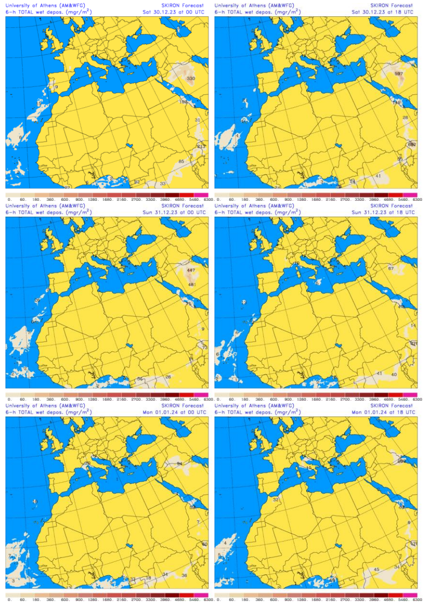
Depósito húmedo de polvo (mg/m 2 ) predicho por el modelo SKIRON para los días 30 y 31 de diciembre de 2023 y 1 de enero de 2024 a las 00 y 18 UTC © Universidad de Atenas.
