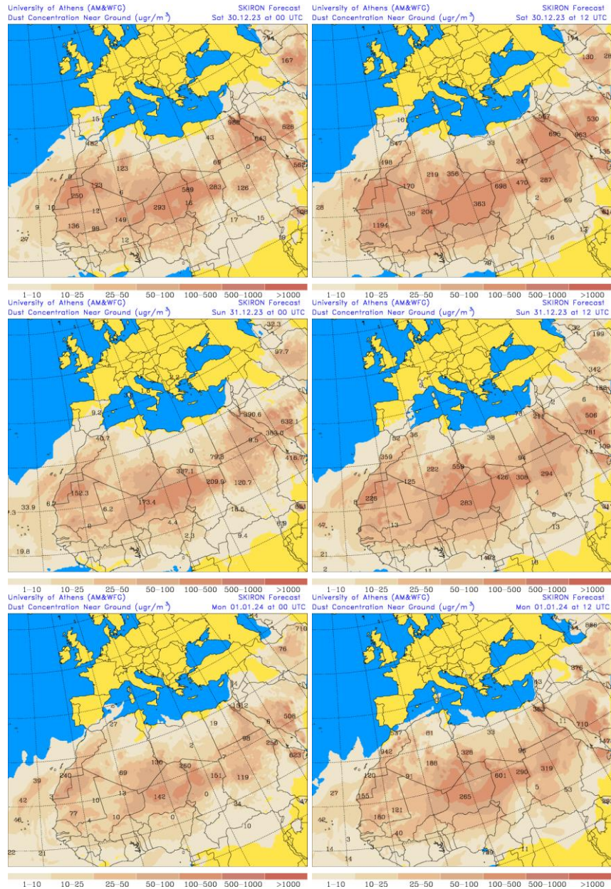
Concentración de polvo ( \mu\text{g}/\text{m}^3 ) predicha por el modelo SKIRON para los días 30 y 31 de diciembre de 2023 y 1 de enero de 2024 a las 00 y 12 UTC © Universidad de Atenas.
