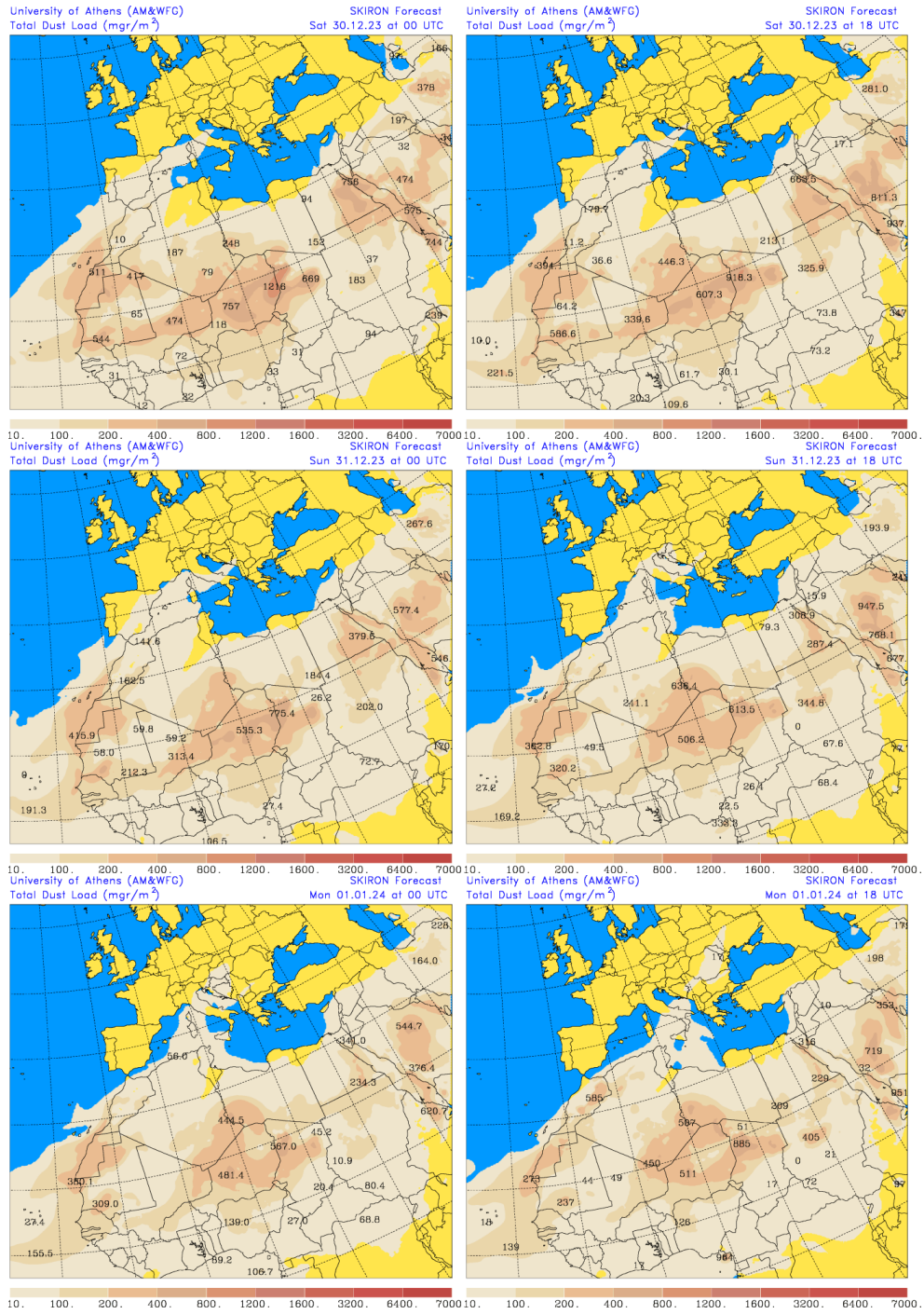
Carga total de polvo (mg/m 2 ) predicha por el modelo SKIRON para los días 30 y 31 de diciembre de 2023 y 1 de enero de 2024 a las 00 y 18 UTC © Universidad de Atenas.
