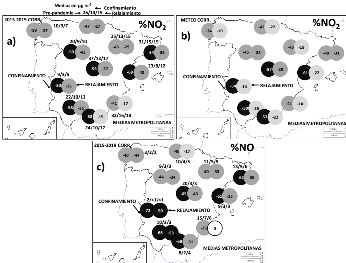
Figura 6. a) En círculos: cambio porcentual promedio de \text{NO}_2 en comparación con las medias de 2015-2019; por encima o por debajo de los círculos: concentraciones promedio (en \mu\text{g m}^{-3} ) durante los períodos de pre-pandemia / confinamiento / relajamiento. b) Ídem, pero los círculos indican reducciones corregidas por meteorología (reducciones respecto a BaU). c) Ídem para concentraciones de \text{NO} y cambio porcentual promedio de \text{NO} en comparación con las medias de 2015-2019. Modificado de Querol et al. (2021).
