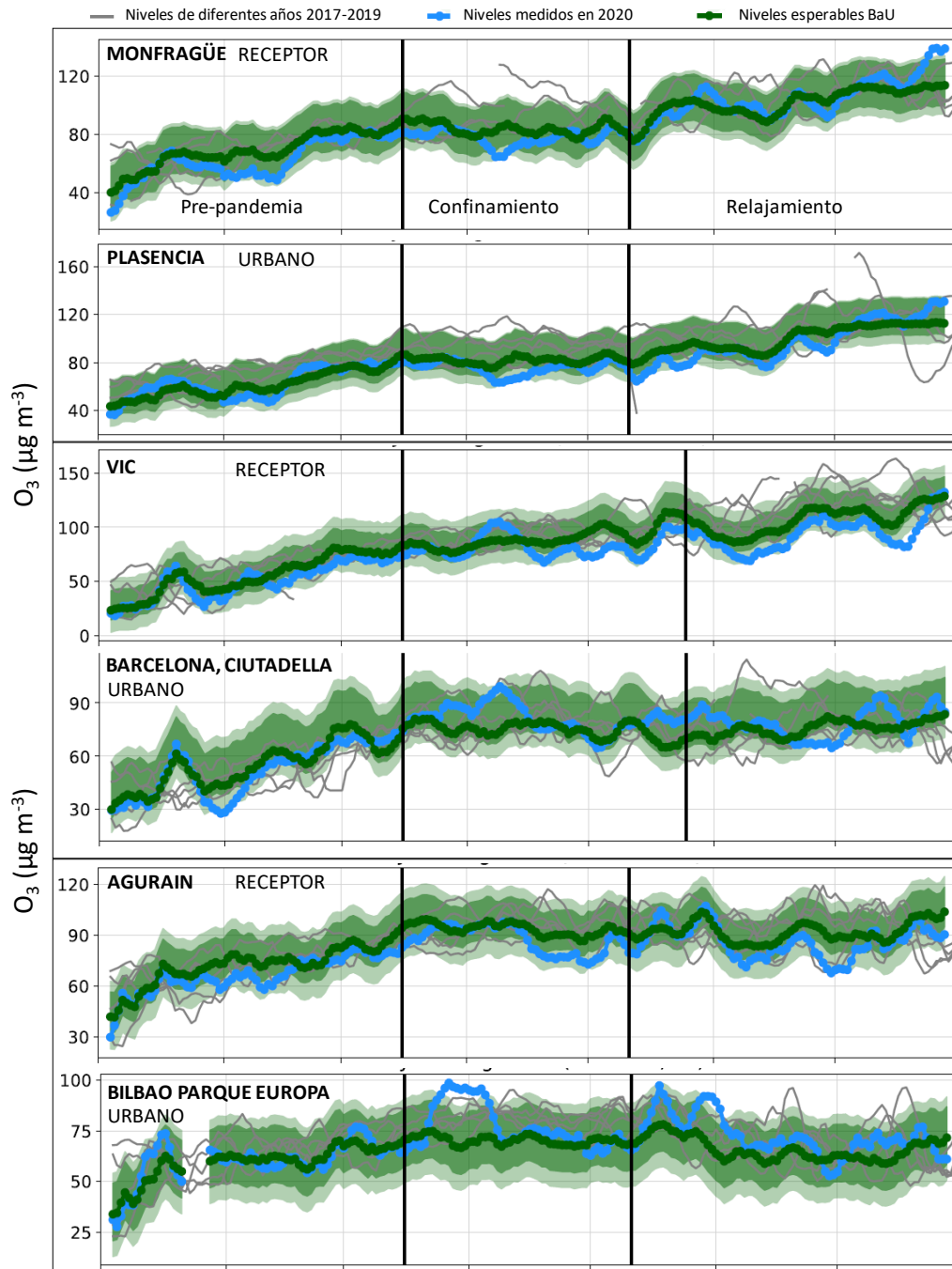
Figuras 10. Ejemplos de resultados de la normalización de series temporales de niveles de O 3 MD8h para estaciones de Extremadura, Barcelona y Bilbao (con ejemplos de zona receptora y urbana en cada caso), mostrando las diferencias entre los niveles de O 3 medidos respecto a los BaU durante las fases pre-pandémica, confinamiento y relajamiento.
