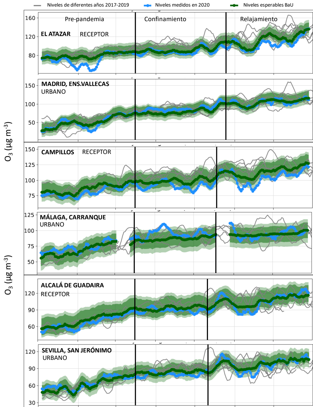
Figuras 11. Ejemplos de resultados de la normalización de series temporales de niveles de O 3 MD8h para estaciones de Madrid, Málaga y Sevilla (con ejemplos de zona receptora y urbana en cada caso), mostrando las diferencias entre los niveles de O 3 medidos respecto a los BaU durante las fases pre-pandémica, confinamiento y relajamiento.
