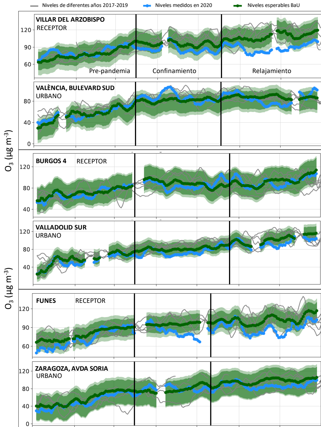
Figuras 12. Ejemplos de resultados de la normalización de series temporales de niveles de O 3 MD8h para estaciones de Valencia, Valladolid y Zaragoza (con ejemplos de zona receptora y urbana en cada caso), mostrando las diferencias entre los niveles de O 3 medidos respecto a los BaU durante las fases pre-pandémica, confinamiento y relajamiento.
