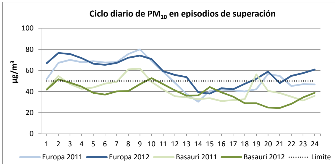
Figura 12. Ciclos diarios en Parque Europa y Basauri .
