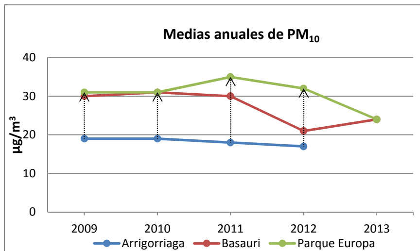
Figura 11. Comparativa de niveles de PM_{10} entre estaciones del Bajo Nervión.
