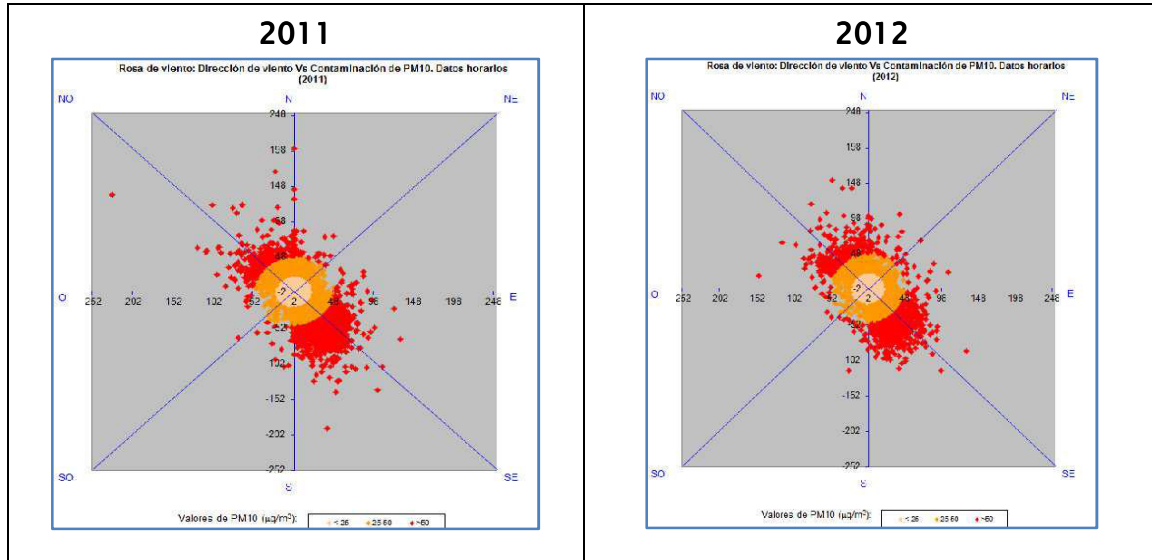
Figura 10. Rosas de viento con contaminación de PM 10 registrada en Parque Europa.
