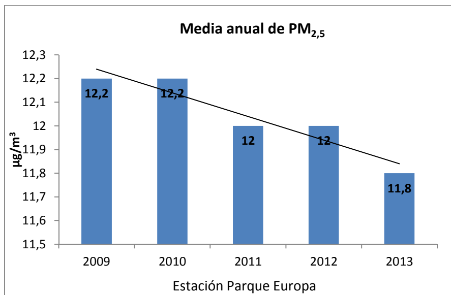
Figura 7. Serie de datos de Pm_{2,5} registrados en los últimos años en Parque Europa.
