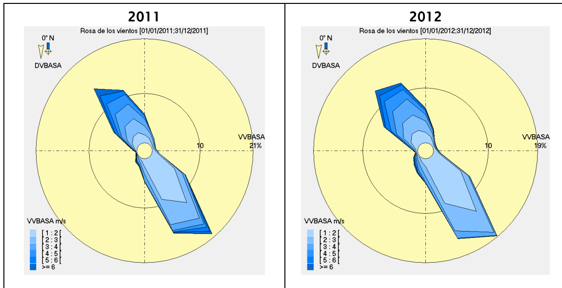
Figura 4. Rosas de vientos de la estación de Basauri en años de superación.
