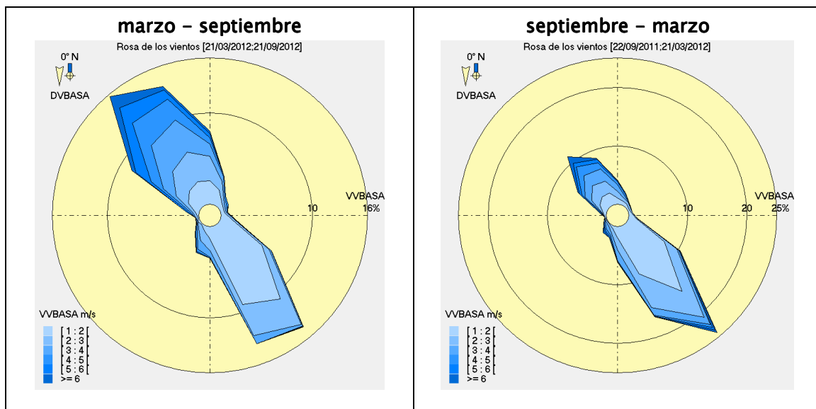
Figura 5. Rosas de vientos por periodos de distribución anual.
