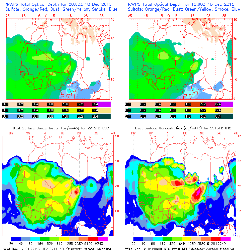
Espesor óptico de aerosoles a 550 nm (arriba) y concentración de polvo a nivel de superficie (abajo) previstos por el modelo NAAPS para el día 10 de diciembre de 2015 a las 00:00 UTC. ©Naval Research Laboratory (NRL), Monterey, CA.
