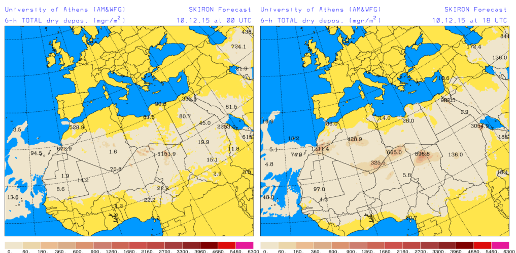
Depósito seco de polvo ( \text{mg}/\text{m}^2 ) predicho por el modelo SKIRON para el día 10 de diciembre de 2015 a las 00 UTC (izquierda) y a las 18 UTC (derecha). © Universidad de Atenas.
