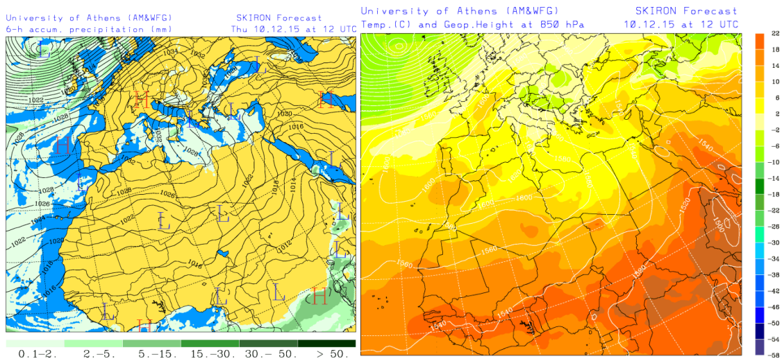
Precipitación acumulada (mm) y presión a nivel del mar (hPa) (izquierda) y campo de temperaturas (°C) y de altura geopotencial a 850 hPa (derecha) previsto por el modelo SKIRON para el día 10 de diciembre de 2015 a las 12 UTC. © Universidad de Atenas.
