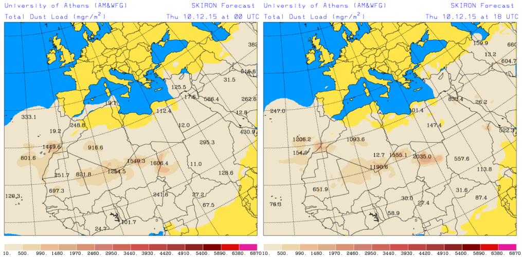
Carga total de polvo (mg/m 2 ) predicha por el modelo SKIRON para los días el día 10 de 2015 a las 00 UTC (izquierda) y a las 18 UTC (derecha). © Universidad de Atenas.
