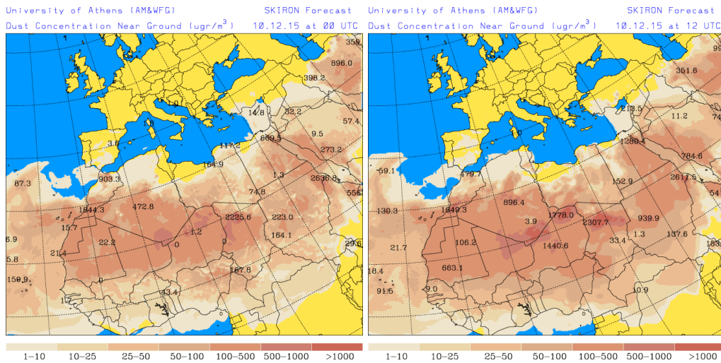
Concentración de polvo ( \mu\text{g}/\text{m}^3 ) predicha por el modelo SKIRON para el día 10 de diciembre de 2015 a las 00 UTC (izquierda) y a las 12 UTC (derecha). © Universidad de Atenas.
