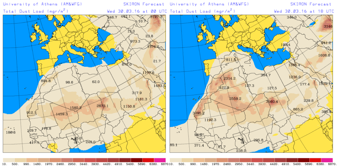
Carga total de polvo (mg/m 2 ) predicha por el modelo SKIRON para el día 30 de marzo de 2016 a las 00 UTC (izquierda) y a las 18 UTC (derecha). © Universidad de Atenas.
