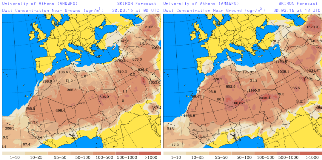
Concentración de polvo ( \mu\text{g}/\text{m}^3 ) predicha por el modelo SKIRON para el día 30 de marzo de 2016 a las 00 UTC (izquierda) y a las 12 UTC (derecha). © Universidad de Atenas.
