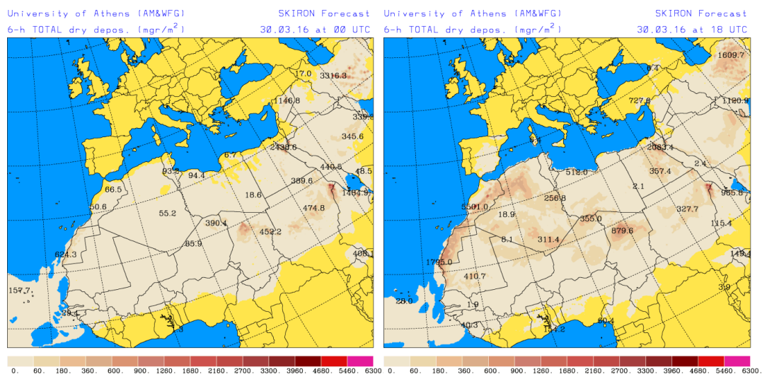
Depósito seco de polvo (mg/m 2 ) predicho por el modelo SKIRON para el día 30 de marzo de 2016 a las 00 UTC (izquierda) y a las 18 UTC (derecha). © Universidad de Atenas.
