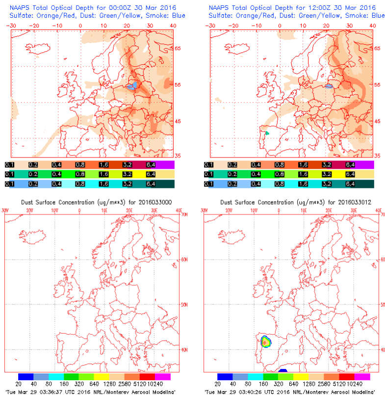
Espesor óptico de aerosoles a 550 nm (arriba) y concentración de polvo a nivel de superficie (abajo) previstos por el modelo NAAPS para el día 30 de marzo de 2016 a las 00:00 UTC. ©Naval Research Laboratory (NRL), Monterey, CA.
