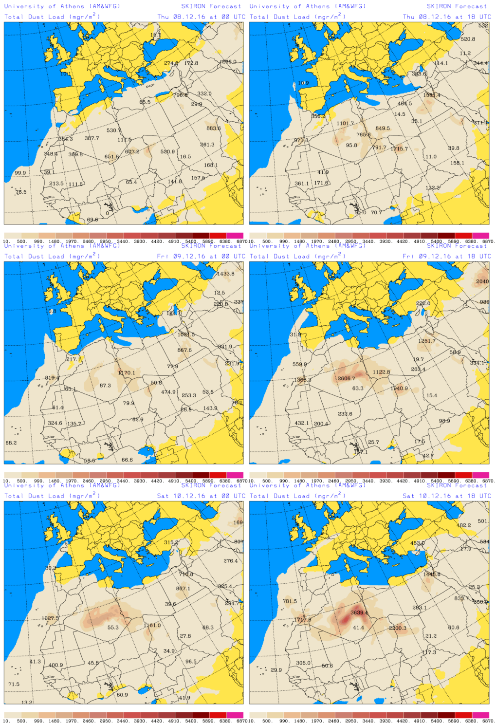
Carga total de polvo (mg/m 2 ) predicha por el modelo SKIRON para los días 8, 9 y 10 de diciembre de 2016 a las 00 UTC (izquierda) y a las 18 UTC (derecha). © Universidad de Atenas.
