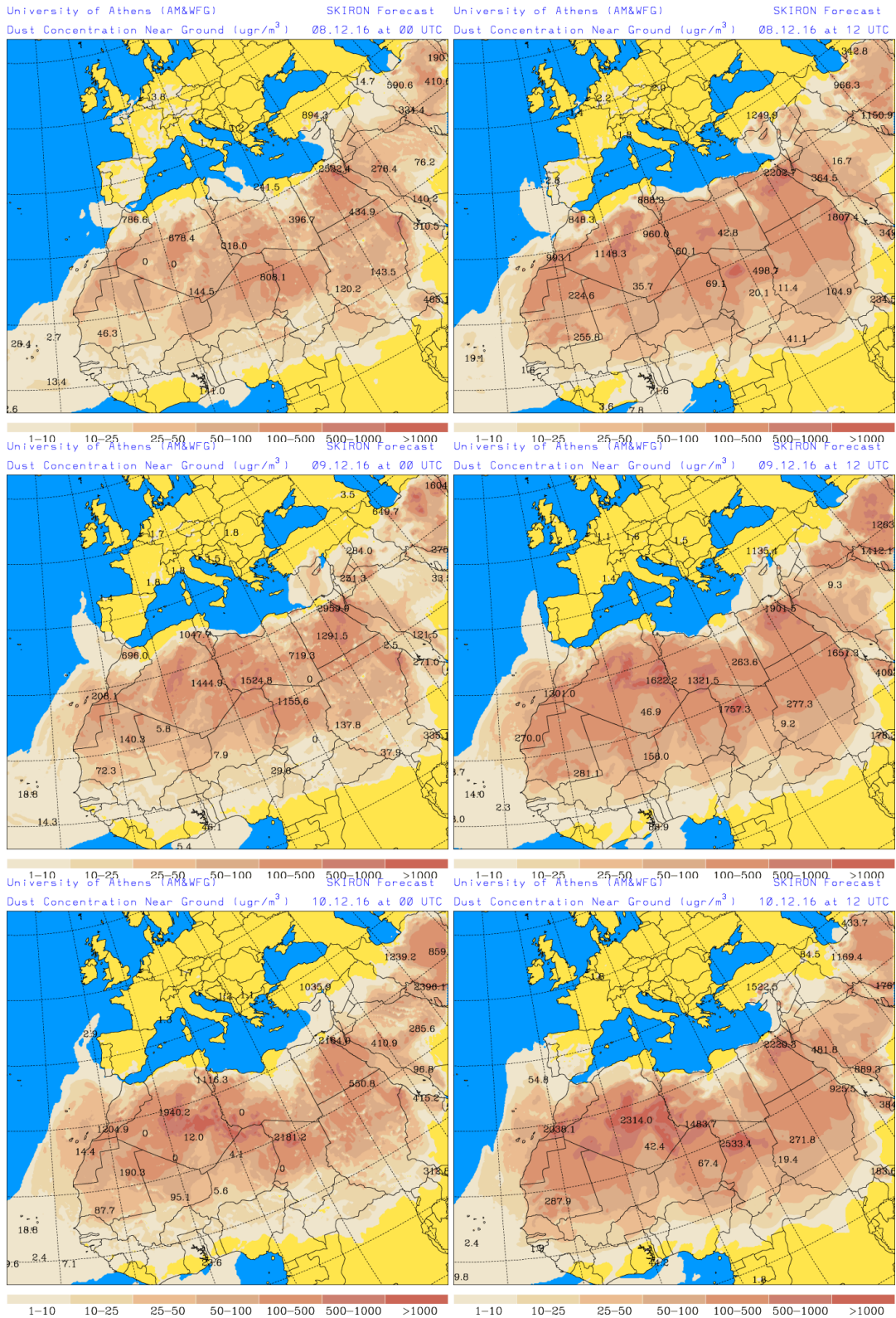
Concentración de polvo ( \mu\text{g}/\text{m}^3 ) predicha por el modelo SKIRON para los días 8, 9 y 10 de diciembre de 2016 a las 00 UTC (izquierda) y a las 12 UTC (derecha). © Universidad de Atenas.
