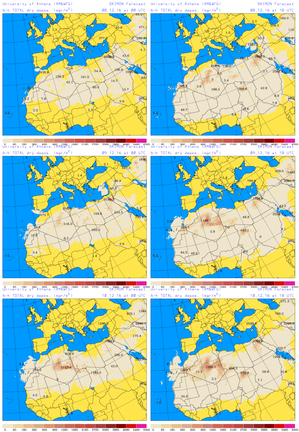
Dépósito húmedo de polvo (mg/m 2 ) predicho por el modelo SKIRON para los días 8, 9 y 10 de diciembre de 2016 a las 00 UTC (izquierda) y a las 18 UTC (derecha). © Universidad de Atenas.
