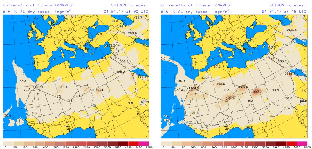
Depósito seco de polvo ( \text{mg}/\text{m}^2 ) predicho por el modelo Skiron para el día 01 de enero de 2017 a las 00 (izquierda) y a las 18 UTC (derecha). © Universidad de Atenas.
