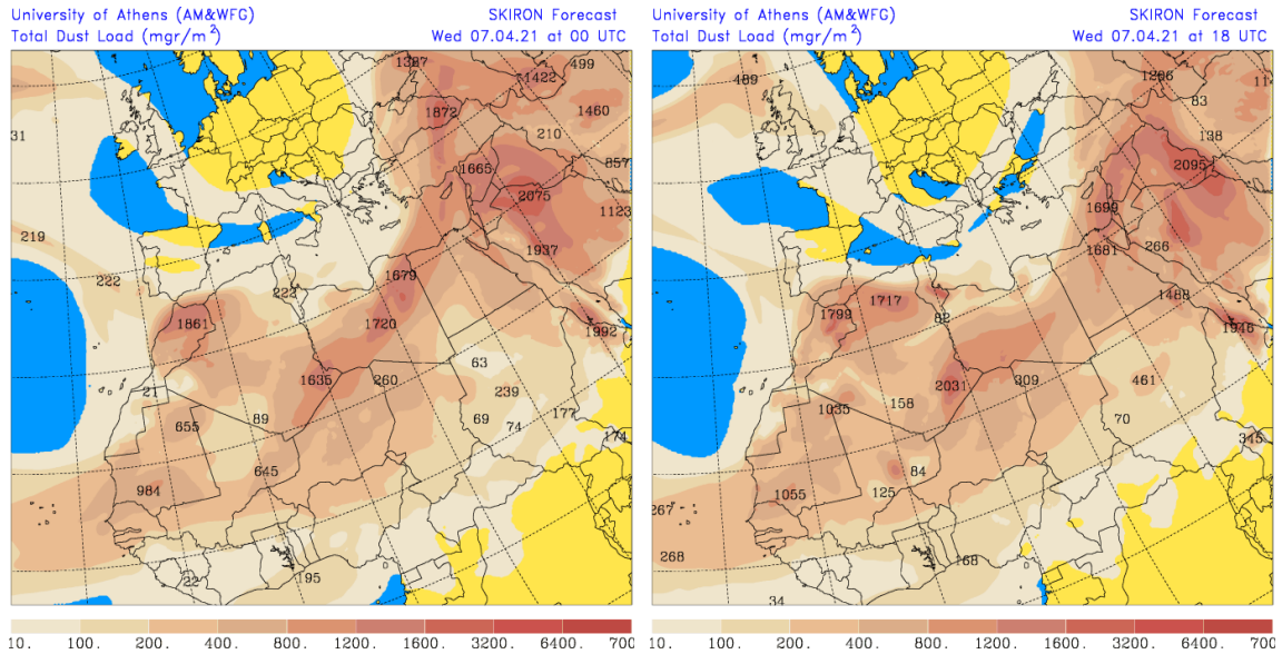
Carga total de polvo (mg/m 2 ) predicha por el modelo SKIRON para el día 7 de abril de 2021 a las 00 y 18 UTC © Universidad de Atenas.
