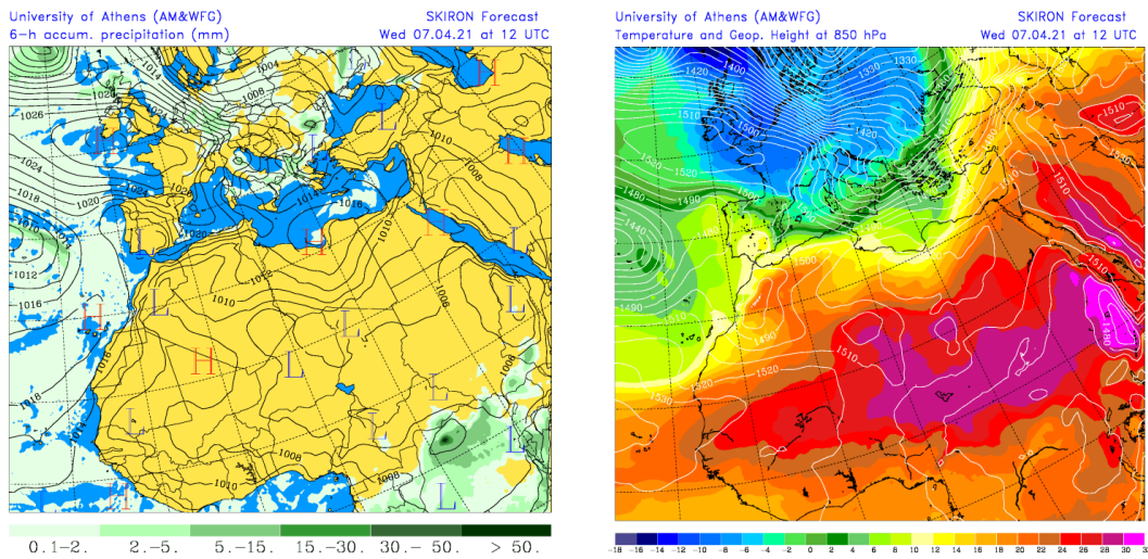
Precipitación acumulada (mm) y presión a nivel del mar (hPa) (izquierda) y campo de temperaturas (°C) y de altura geopotencial a 850 hPa (derecha) previsto por el modelo SKIRON para el día 7 de abril de 2021 a las 12 UTC © Universidad de Atenas.
