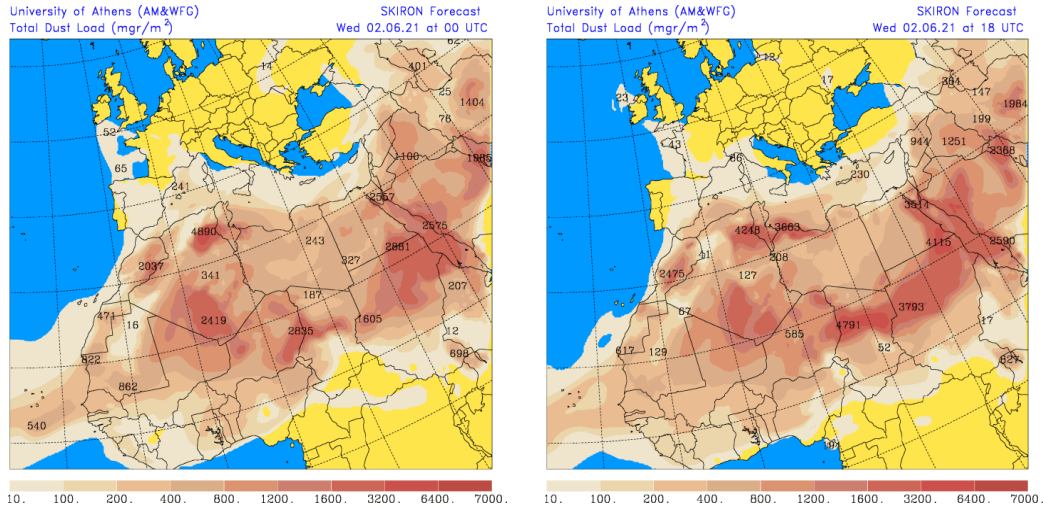
Carga total de polvo ( \text{mg}/\text{m}^2 ) predicha por el modelo SKIRON para el día 2 de junio de 2021 a las 00 y 18 UTC © Universidad de Atenas.
