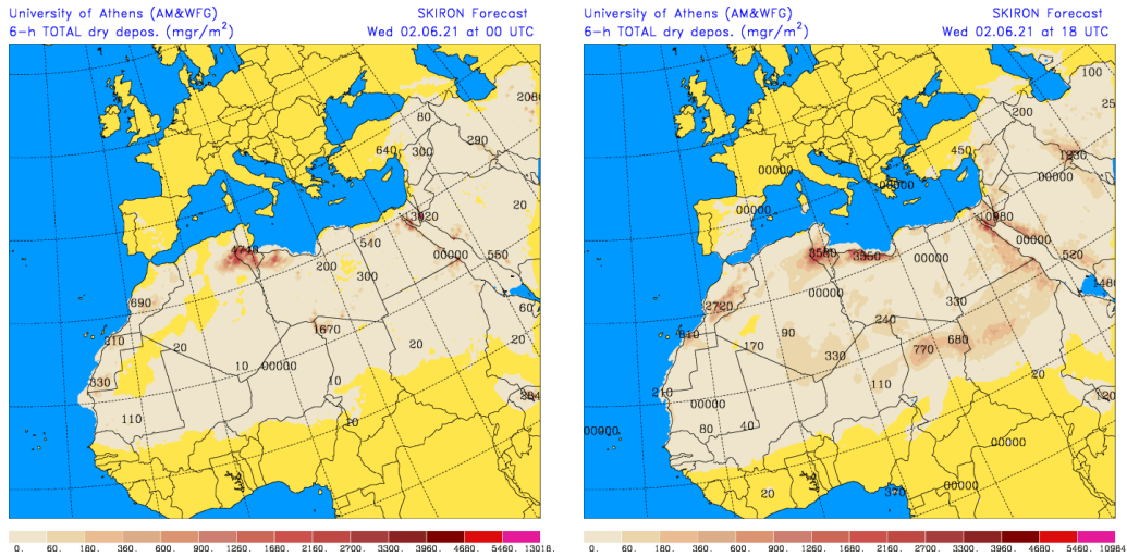
Depósito seco de polvo (mg/m 2 ) predicho por el modelo SKIRON para el día 2 de junio de 2021 a las 00 y 18 UTC © Universidad de Atenas.
