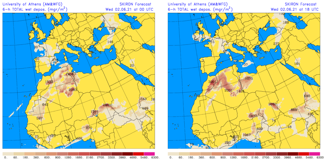
Depósito húmedo de polvo (mg/m 2 ) predicho por el modelo SKIRON para el día 2 de junio de 2021 a las 00 y 18 UTC © Universidad de Atenas.
