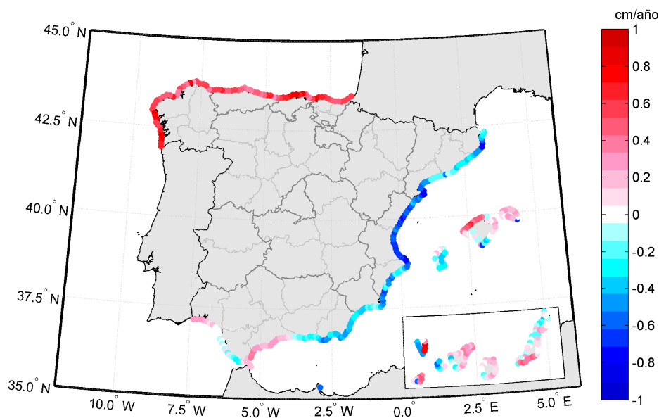
Figura 18. Tendencia de cambio observada en los últimos 60 años en la altura de ola sólo excedida 12 horas al año, H_{s12} . Fuente: IH Cantabria.
