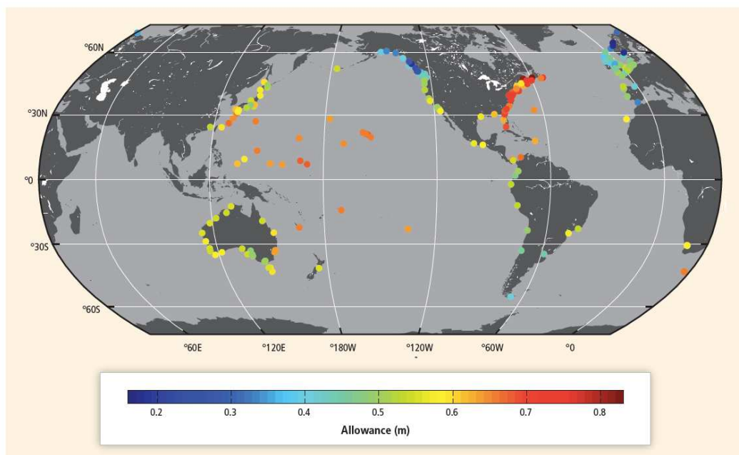
Figura 9. Incremento en la altura de las defensas de protección frente a inundación costera que sería necesario en el periodo 2081-2100 para preservar la misma frecuencia de excedencias experimentada en el periodo 1986-2005. El resultado se muestra para la localización de 182 mareógrafos y considerando las proyecciones regionales de aumento del mar relativo correspondientes al RCP4.5. (Fuente: Wong et al. IPCC-AR5).
