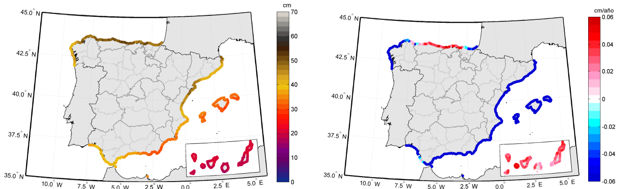
Figura 13. Marea meteorológica asociada a 50 años de período de retorno (izquierda) y tasa de cambio observada en los últimos 60 años en la marea meteorológica (derecha). Fuente: IH Cantabria.
