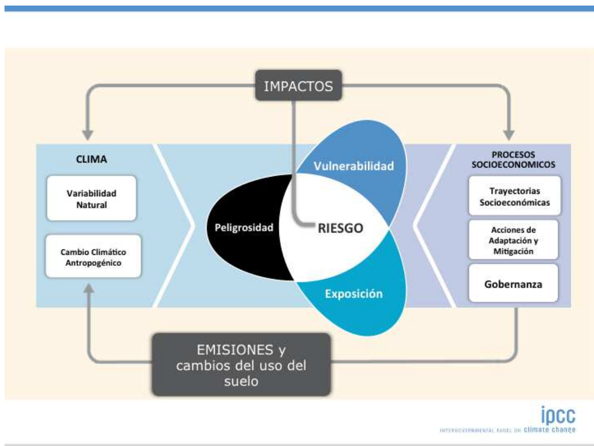
Figura 6. Esquema conceptual de la evaluación del riesgo derivado de impactos relacionados con el clima Fuente: Modificada de IPCC-AR5, 2014.
