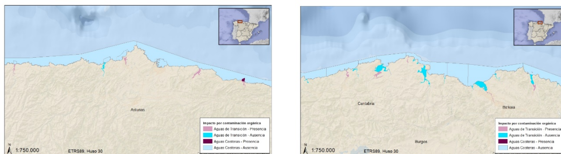
Figura 37. Masas de agua costeras y de transición impactadas por materia orgánica en la demarcación
