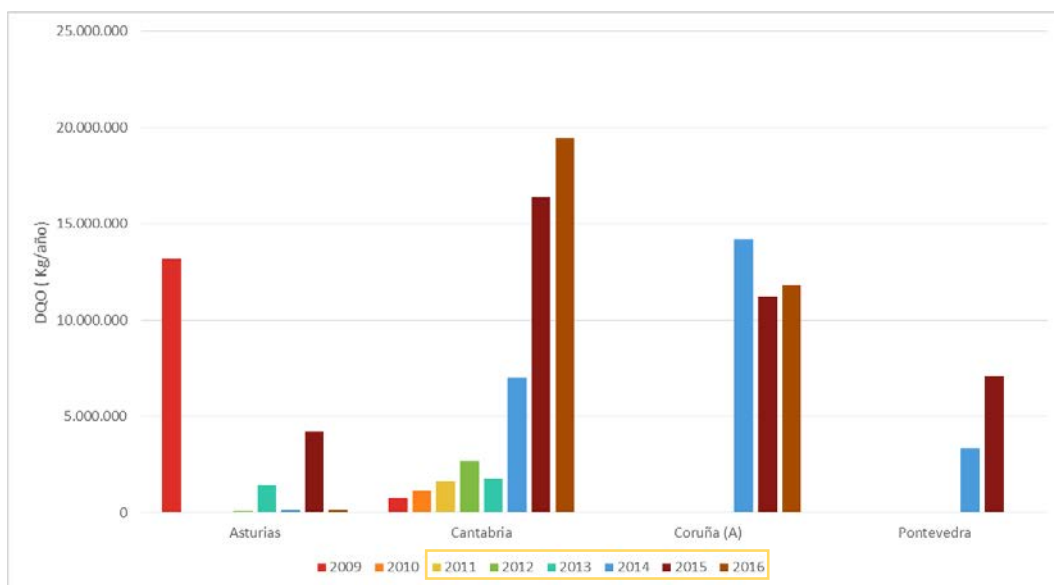
Figura 33. DQO aportada a la demarcación por instalaciones que notifican al Registro PRTR
