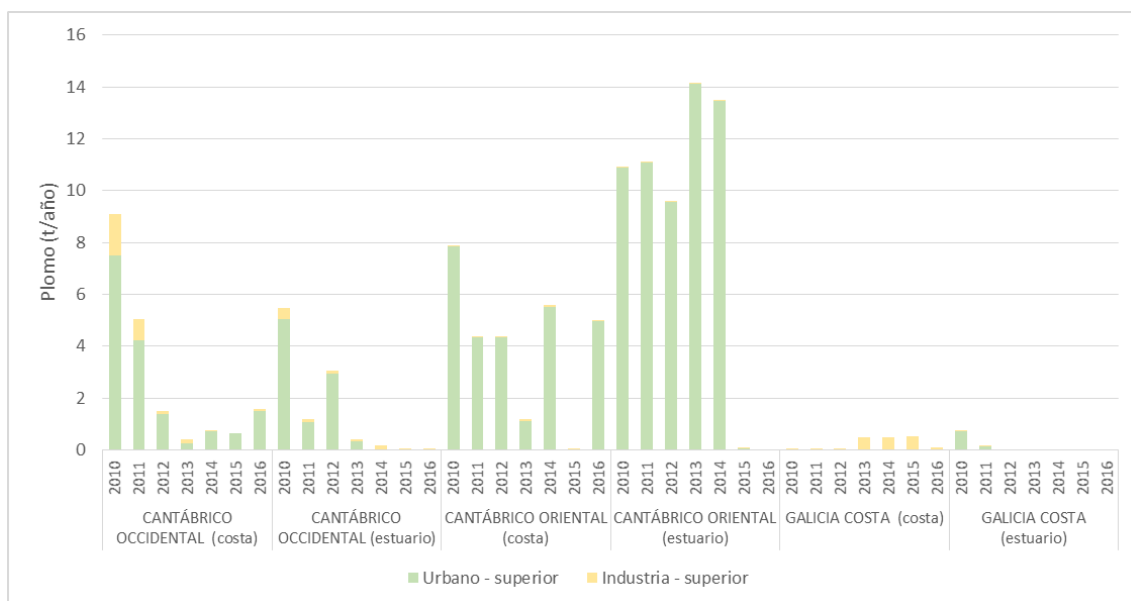
Figura 43. Aportes de plomo por vertidos directos
