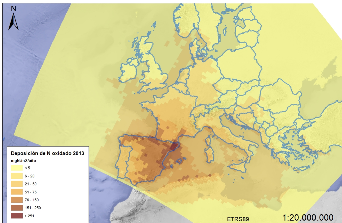
Figura 30. Deposición de nitrógeno oxidado procedente únicamente de emisiones españolas
