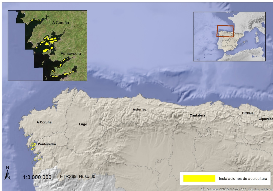
Figura 3. Instalaciones de acuicultura de la Demarcación noratlántica en 2016
