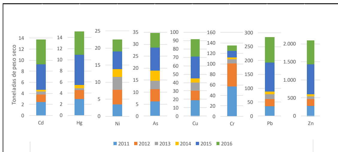
Figura 69. Aportes de metales pesados (t/año) contenidos en los sedimentos vertidos al mar procedentes de los dragados portuarios
