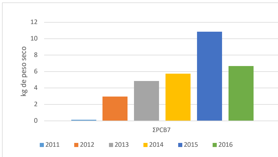
Figura 70. Aportes de PCB's \Sigma 7 congéneres IUPAC (Kg/año) contenidos en los vertidos al mar procedentes de los dragados portuarios
