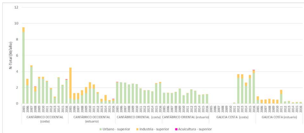
Figura 8. Aportes de nitrógeno total por vertidos directos
