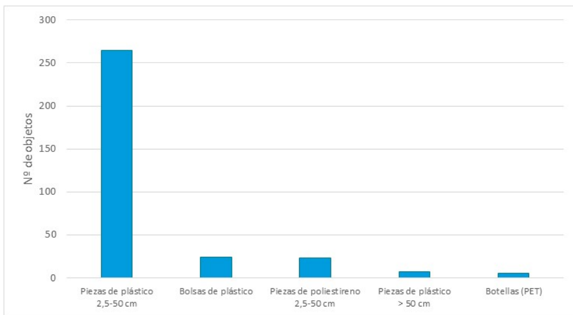
Figura 88. Objetos encontrados en el río Nervión durante 2016
