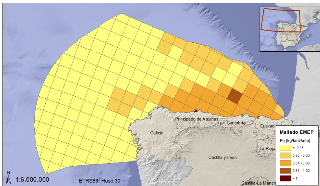
Figura 78. Masa de plomo depositado desde la atmósfera por unidad de superficie durante el año 2014
