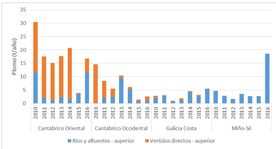
Figura 42. Aportes de plomo desde ríos y vertidos directos
