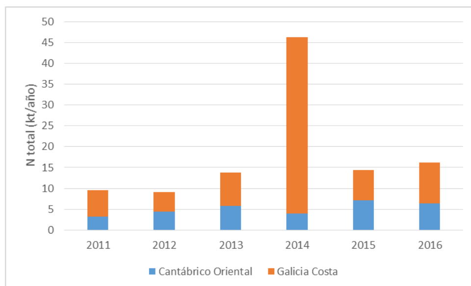
Figura 18. Aporte medio anual de nitrógeno total desde ríos para aquellos que tienen datos todos los años del periodo 2011-2016
