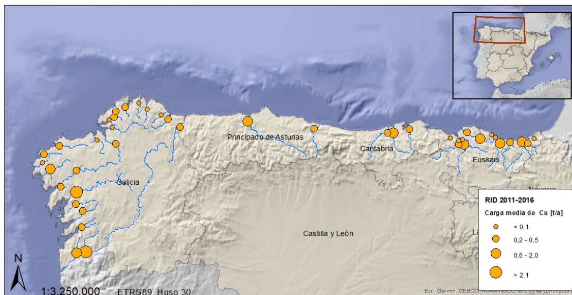
Figura 64. Aporte medio anual de cobre por ríos en el periodo 2011-2016
