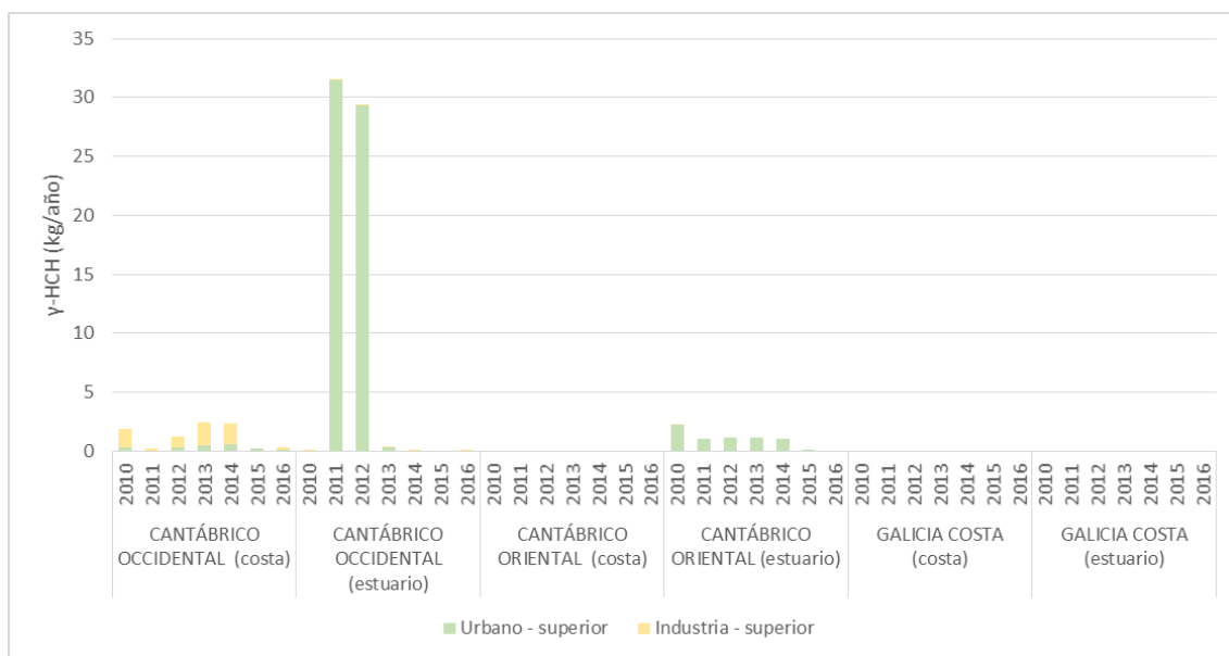
Figura 49. Aportes de \gamma -hexaclorociclohexano por vertidos directos (Fuente: Figura elaborada por el CEDEX a partir de datos del Programa RID del Convenio OSPAR)
