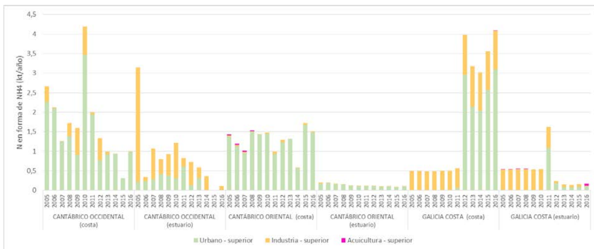
Figura 6. Aportes de nitrógeno en forma de amonio por vertidos directos
