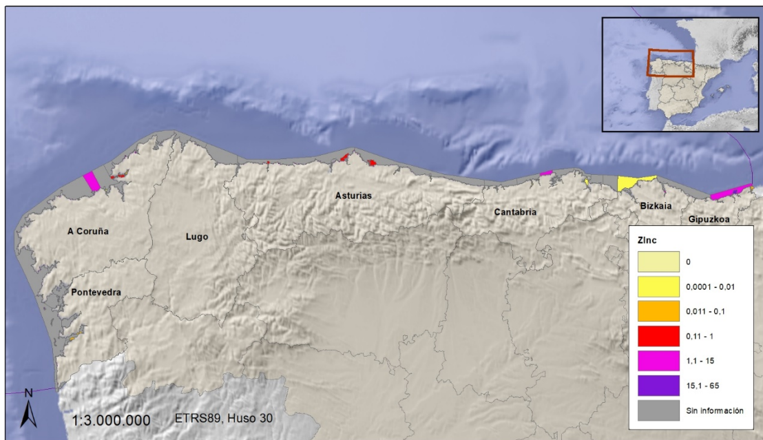
Figura 56. Aportes de zinc por vertidos directos (t/año) por masa de agua costera o de transición
