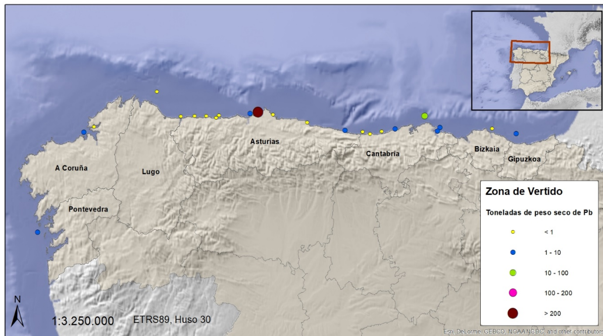
Figura 74. Aportes de Pb contenidos en los sedimentos vertidos al mar procedentes de los dragados portuarios
