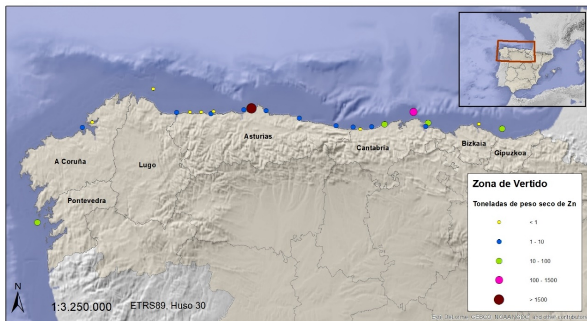
Figura 75. Aportes de Zn contenidos en los sedimentos vertidos al mar procedentes de los dragados portuarios
