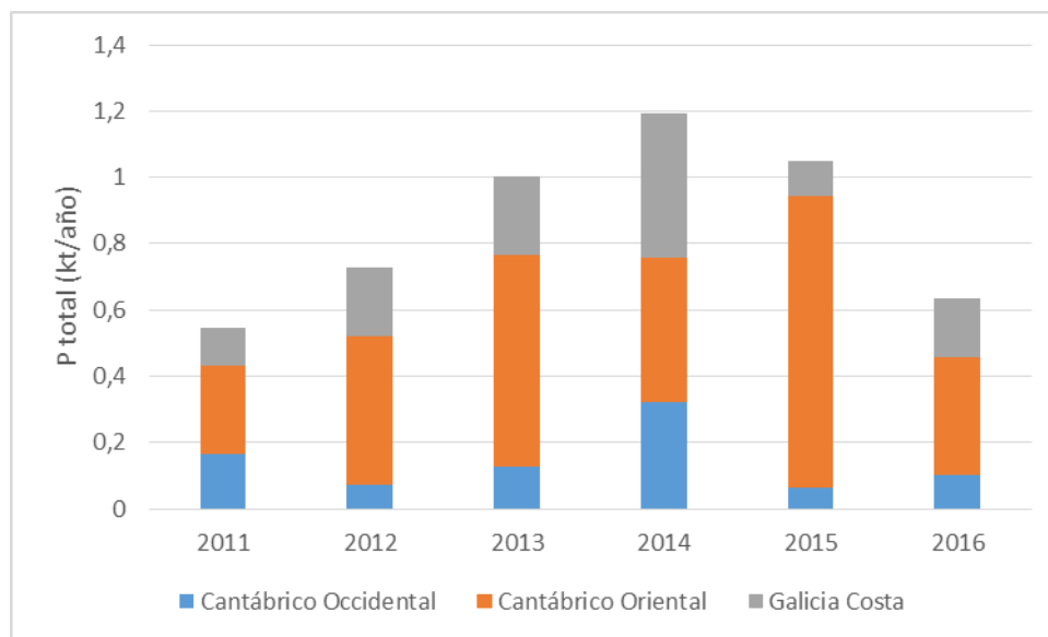
Figura 20. Aporte medio anual de fósforo total desde ríos para aquellos que tienen datos todos los años del periodo 2011-2016
