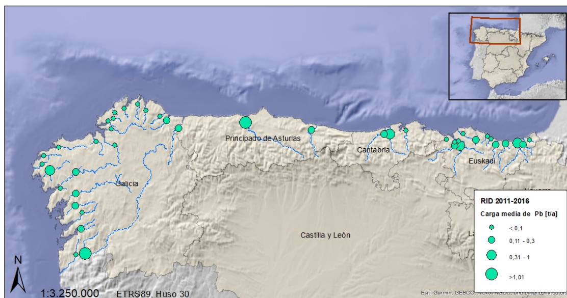
Figura 63. Aporte medio anual de plomo por ríos en el periodo 2011-2016
