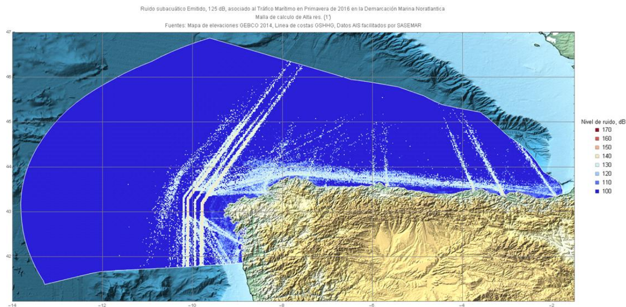
Figura 7. Nivel medio de emisión sonora por navegación a 125 Hz en primavera de 2016
