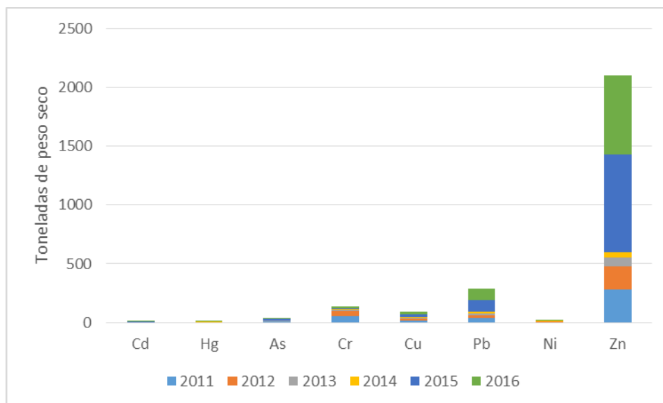
Figura 68. Aportes de metales pesados (t/año) contenidos en los sedimentos vertidos al mar procedentes de los dragados portuarios
