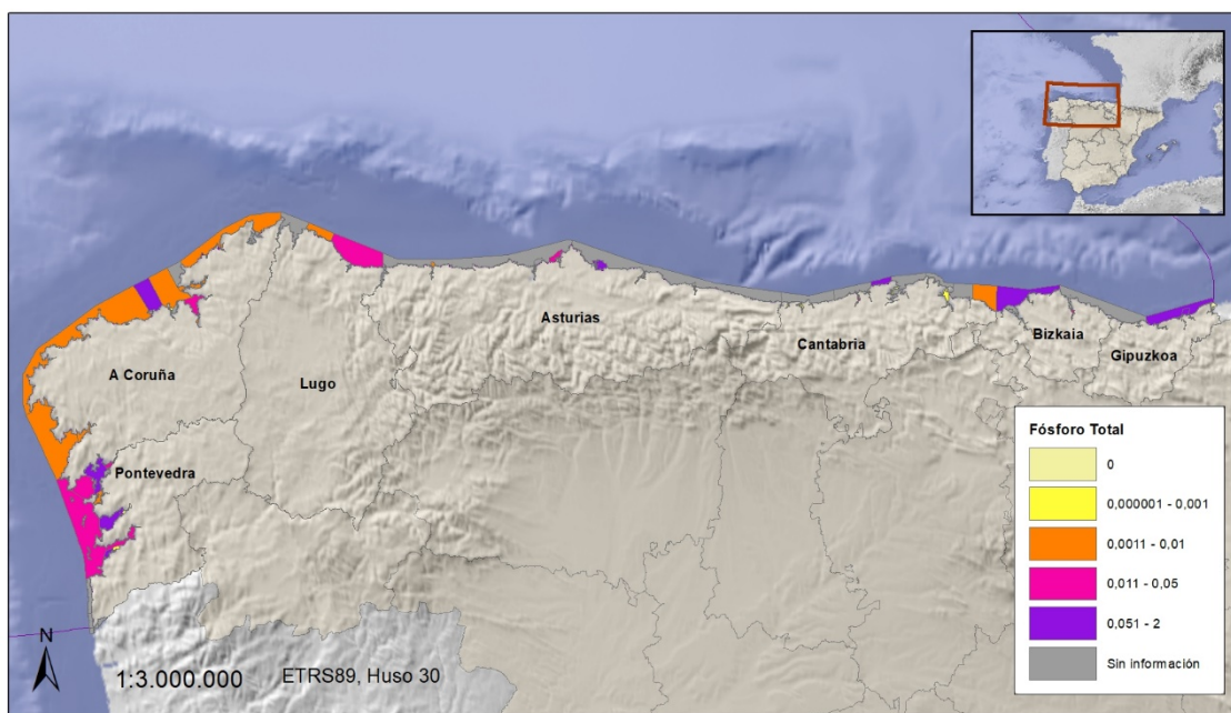
Figura 15. Aportes directos de fósforo total por masa de agua costera (kt/año)
