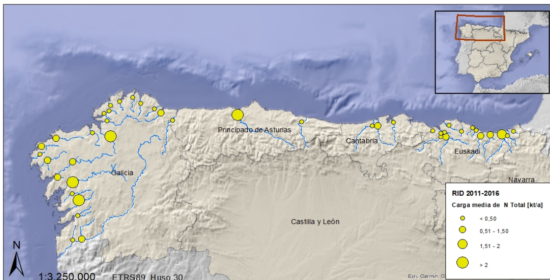
Figura 23. Aporte medio anual de nitrógeno total aportada por ríos
