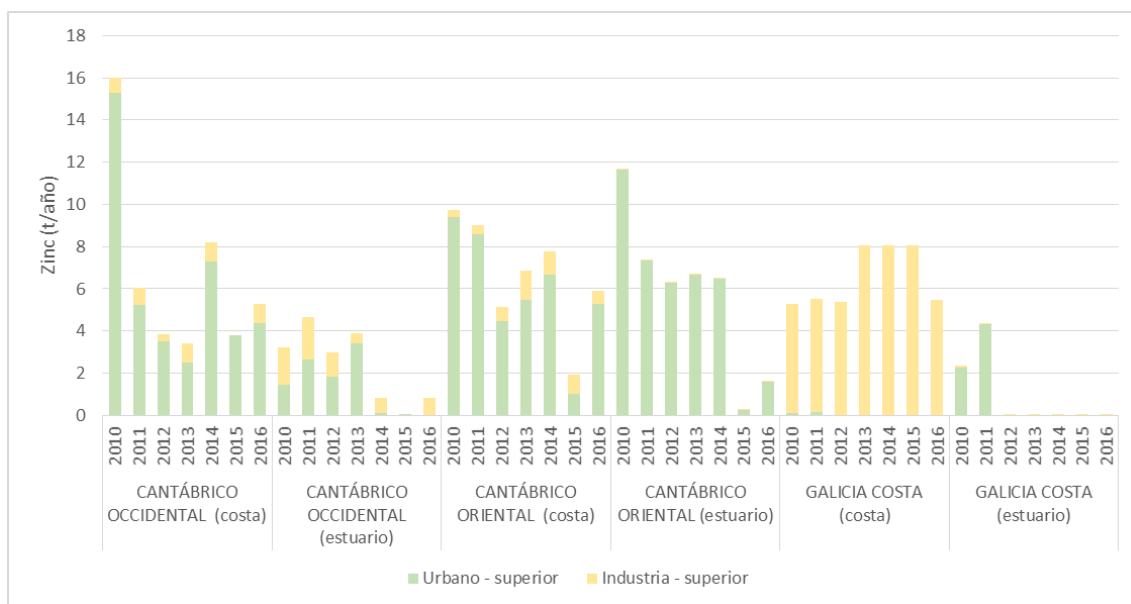
Figura 47. Aportes de zinc por vertidos directos
