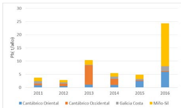
Figura 58. Aporte medio anual de plomo por ríos
