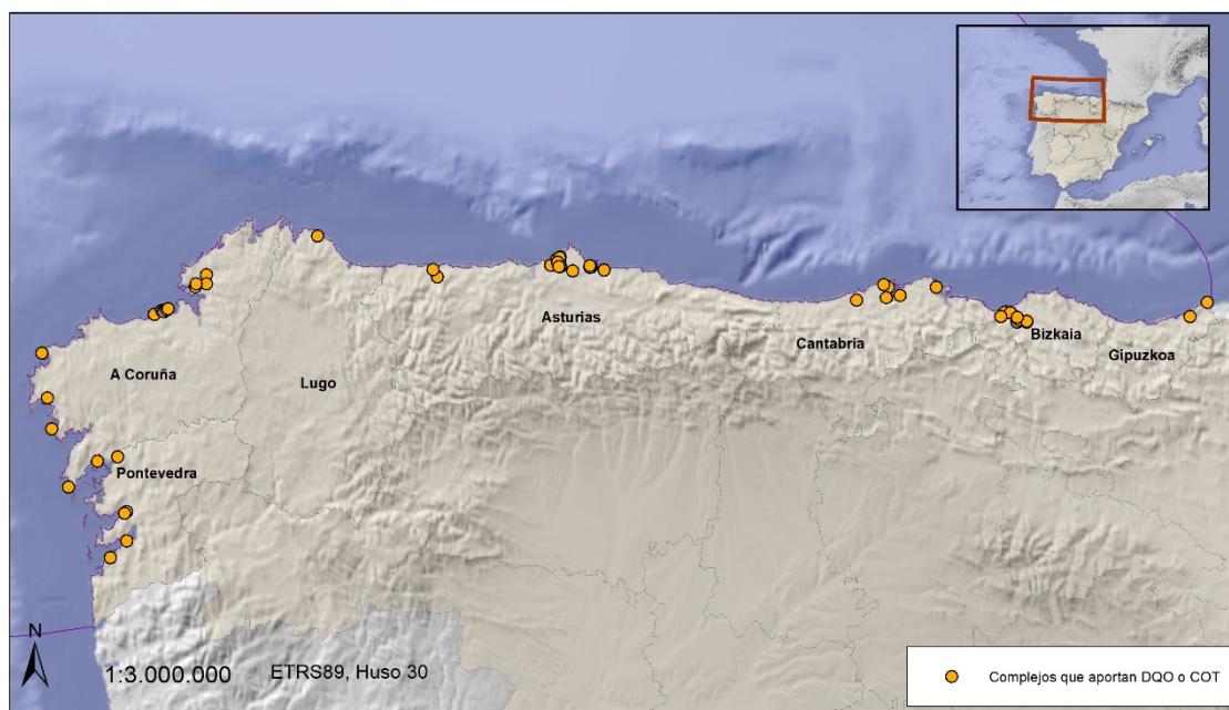
Figura 35. Localización de complejos que notifican al Registro PRTR emisiones de DQO o COT al litoral
