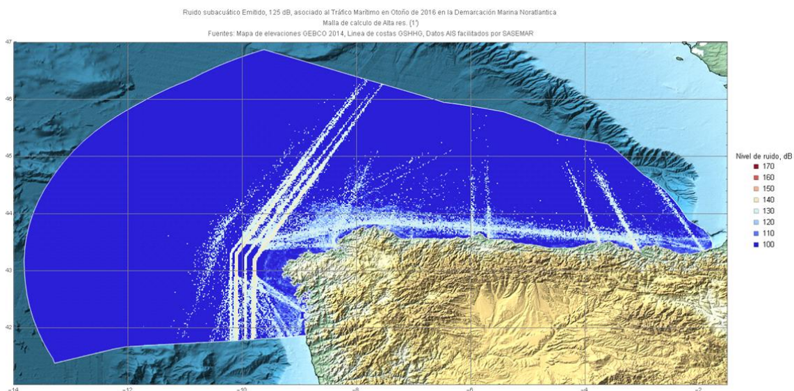
Figura 9. Nivel medio de emisión sonora por navegación a 125 Hz en otoño de 2016
