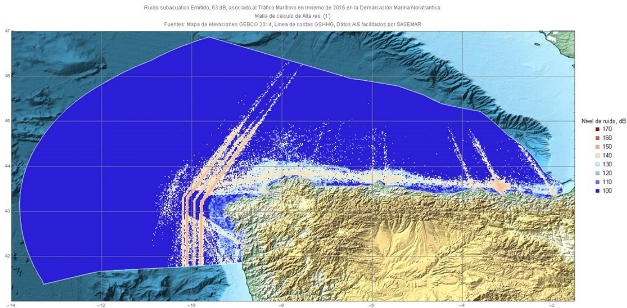
Figura 2. Nivel medio de emisión sonora por navegación a 63 Hz en invierno de 2016
