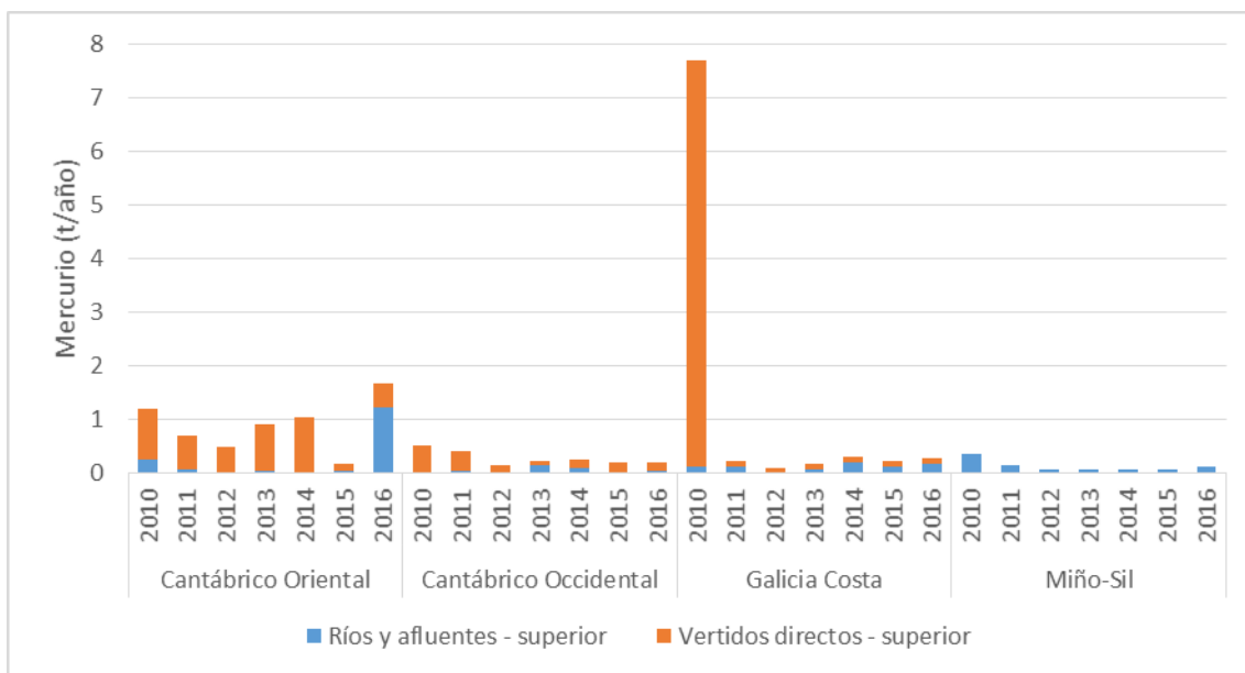
Figura 40. Aportes de mercurio desde ríos y vertidos directos
