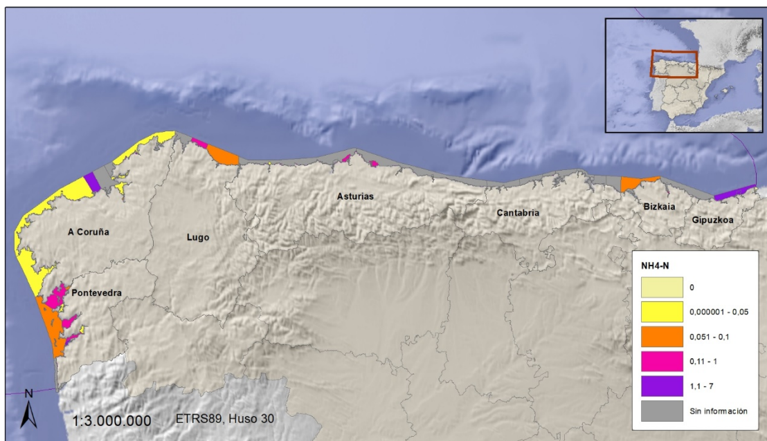
Figura 11. Aportes directos de nitrógeno en forma de amonio por masa de agua costera (kt/año)
