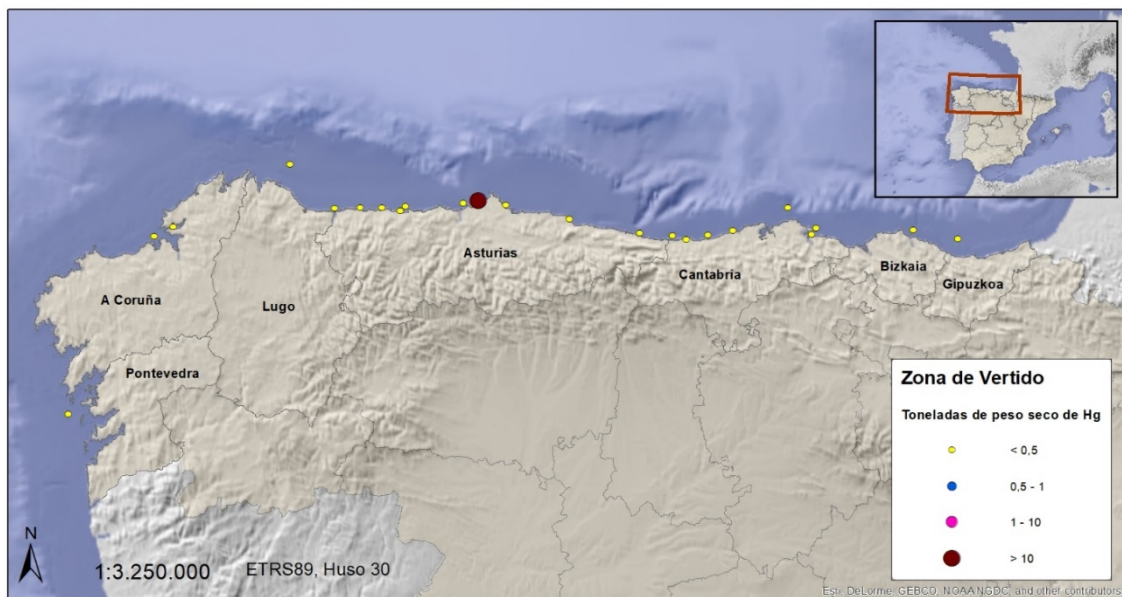
Figura 72. Aportes de Hg contenidos en los sedimentos vertidos al mar procedentes de los dragados portuarios
