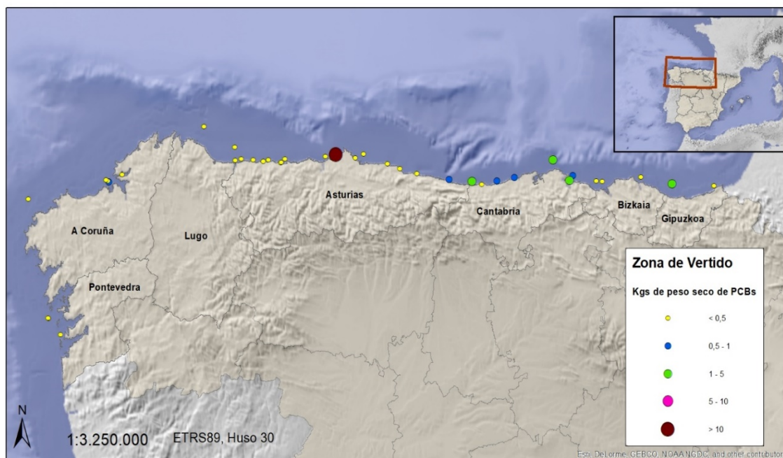
Figura 76. Aportes de PCB's ( \Sigma 7 congéneres IUPAC) contenidos en los sedimentos vertidos al mar procedentes de los dragados portuarios
