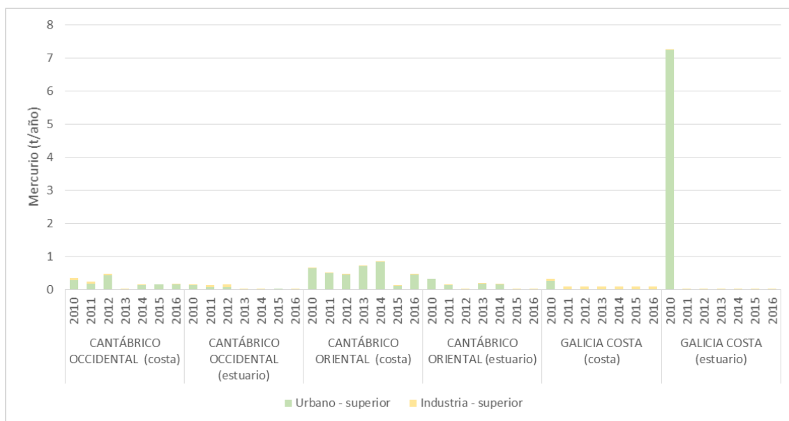
Figura 41. Aportes de mercurio por vertidos directos
