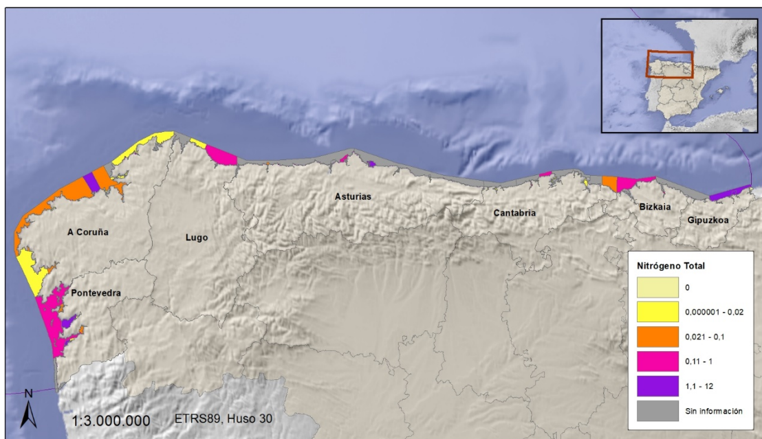
Figura 13. Aportes directos de nitrógeno total por masa de agua costera (kt/año)
