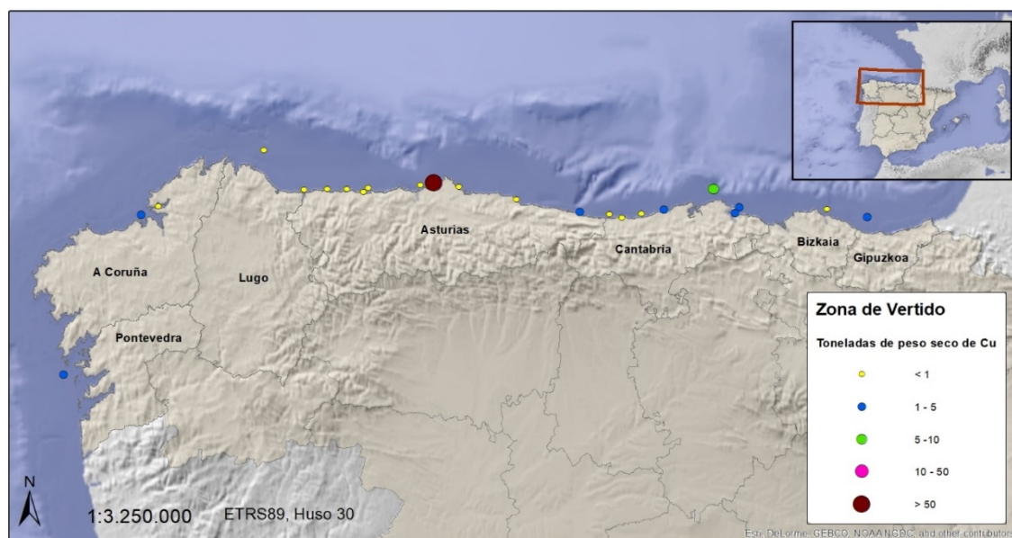
Figura 73. Aportes de Cu contenidos en los sedimentos vertidos al mar procedentes de los dragados portuarios
