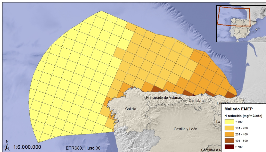
Figura 27. Masa de nitrógeno reducido depositado desde la atmósfera por unidad de superficie durante el año 2014
