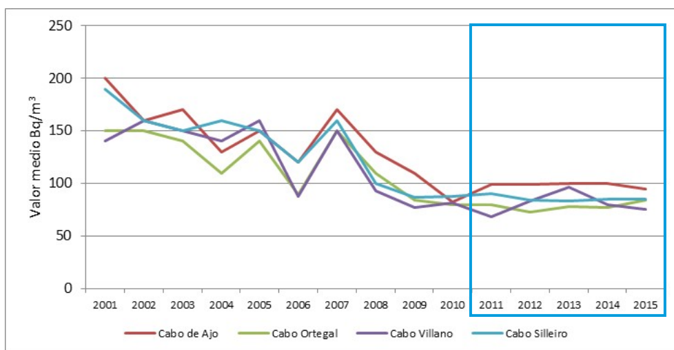
Figura 83. Concentración de actividad de tritio (Bq/m 3 ) en las estaciones de la demarcación (Fuente: Figura elaborada por el CEDEX con datos publicados por el Consejo de Seguridad Nuclear)
