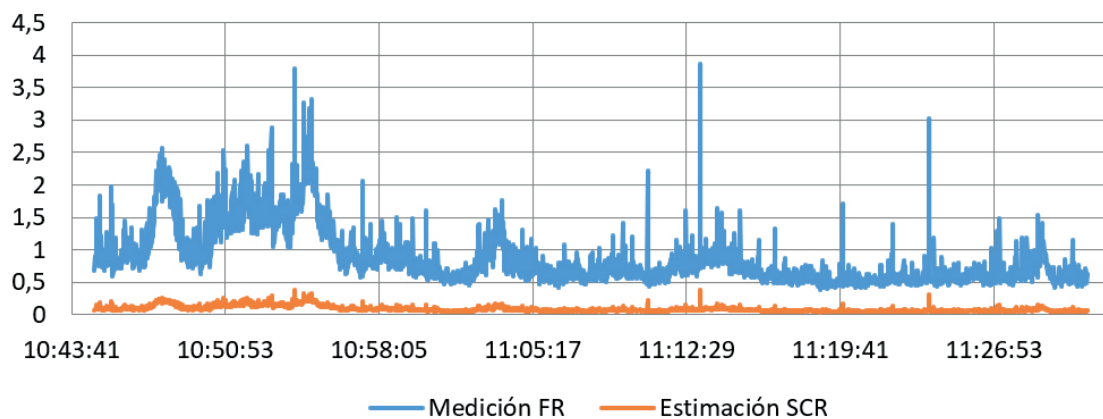
Fig. 3.3. Concentración de fracción respirable de partículas y estimación de SCR. (Fuente: INS)
