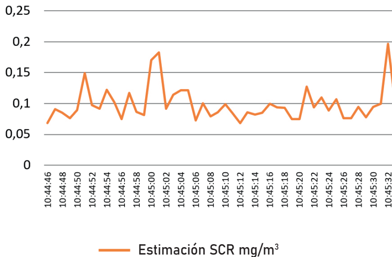
Fig. 3.5. Detalle de la concentración estimada de SCR (Fuente: INS)
