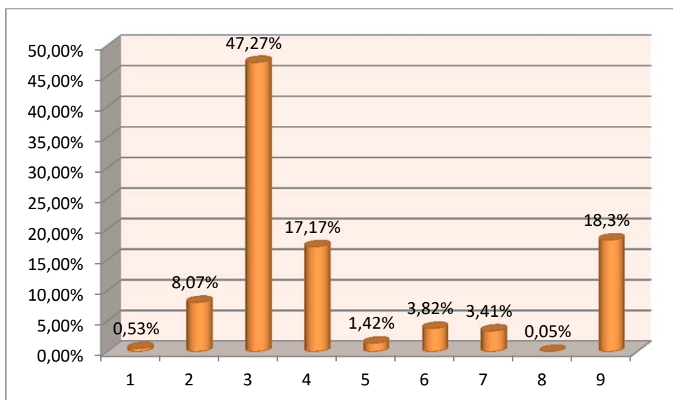
Figura 6.1. Requisitos energéticos de las etapas de producción en la fabricación de paneles fotovoltaicos como porcentajes del requisito de energía bruta (GER).
