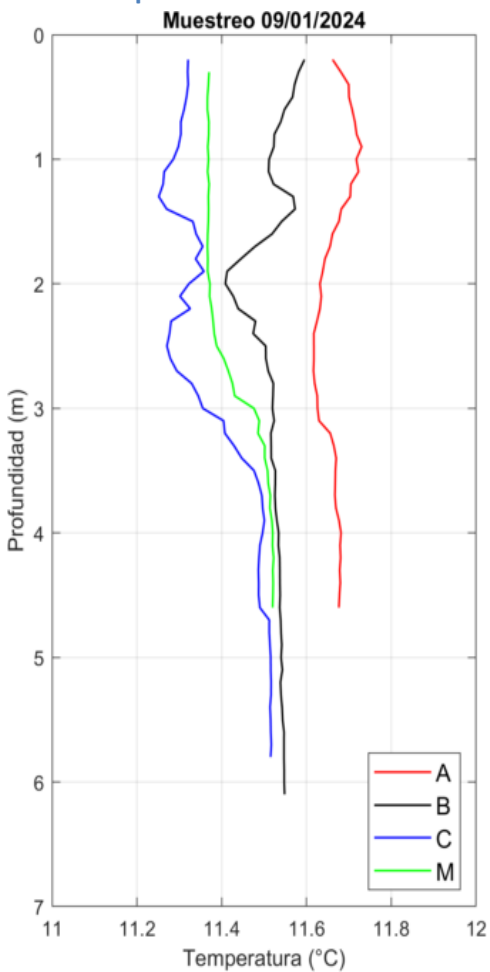
Figura 25. Perfiles de Temperatura obtenidos el día 09/01/24 con el CTD.
