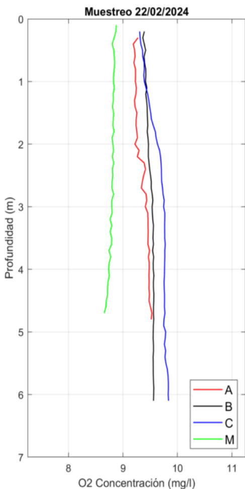
Figura 40. Perfiles de Concentración de O2 obtenidos el día 22/02/24 con el CTD.
