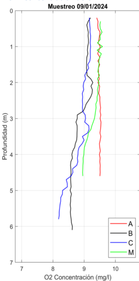
Figura 37. Perfiles de Concentración de O 2 obtenidos el día 09/01/24 con el CTD.
