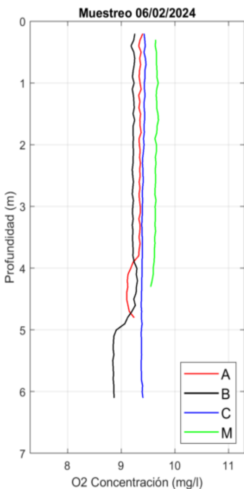
Figura 39. Perfiles de Concentración de O2 obtenidos el día 06/02/24 con el CTD.
