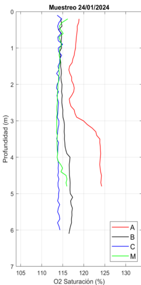
Figura 34. Perfiles de Saturación de O2 obtenidos el día 24/01/24 con el CTD.
