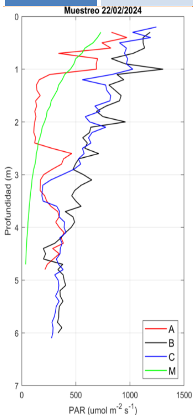
Figura 52. Perfiles de Luz PAR obtenidos el día 22/02/24 con el CTD.
