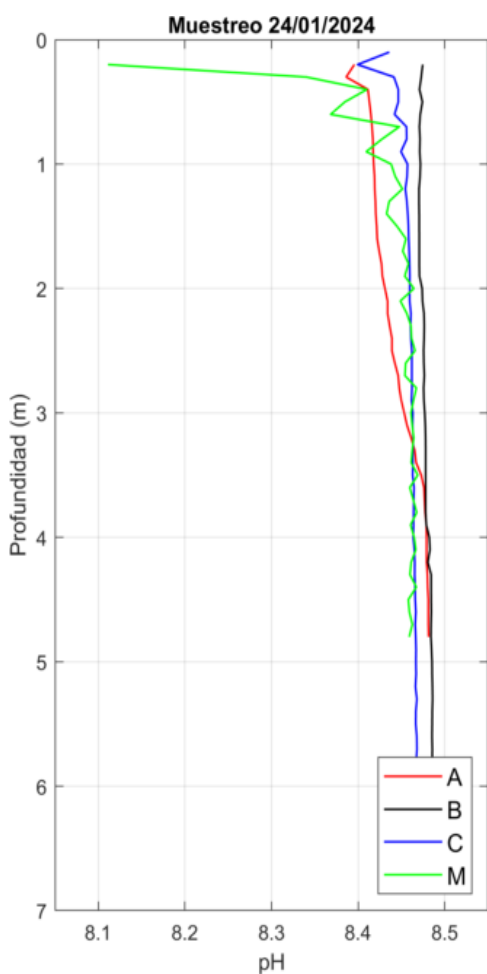
Figura 46. Perfiles de pH obtenidos el día 24/01/24 con el CTD.
