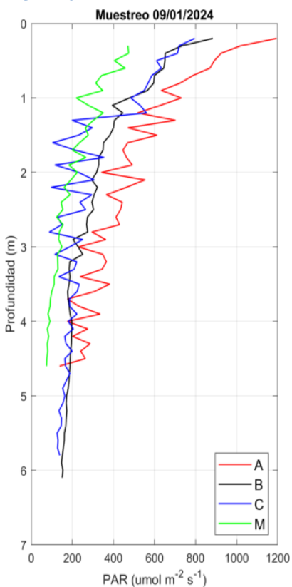
Figura 49. Perfiles de Luz PAR obtenidos el día 09/01/24 con el CTD.
