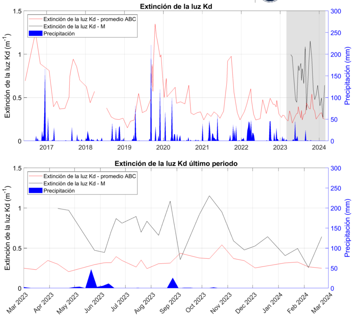
Figura 15: Coeficiente de extinción de la luz a partir de los datos obtenidos en los muestreos del proyecto DMMEM y BELICH en las estaciones de muestreo A, B, C y M, comparado con la precipitación en el aeropuerto de San Javier obtenido a partir de los datos de la AEMET. En la parte superior se muestra la serie desde 2016 y en la parte inferior el último año.
