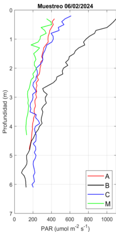
Figura 51. Perfiles de Luz PAR obtenidos el día 06/02/24 con el CTD.
