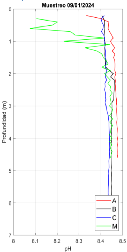
Figura 45. Perfiles de pH obtenidos el día 09/01/24 con el CTD.
