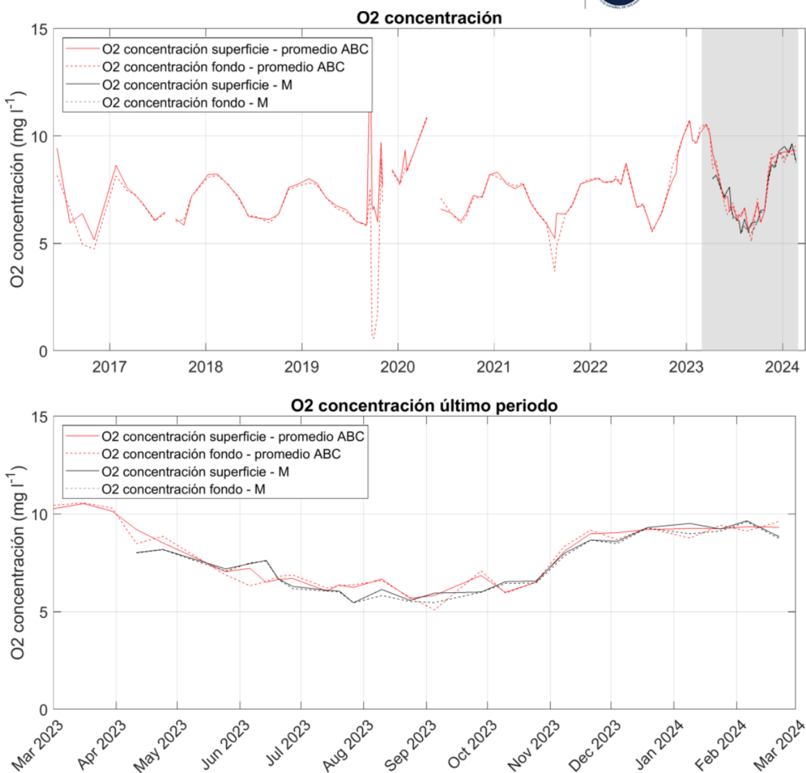
Figura 17: Series temporales promedio de oxígeno disuelto para las capas superficiales (0,5 m; línea continua) y de fondo (entre 4 y 6m dependiendo de la estación, Figura 1; línea discontinua) de los muestreos del proyecto DMMEM y BELICH para las estaciones de muestreo A, B, C y M de la laguna del Mar Menor.
