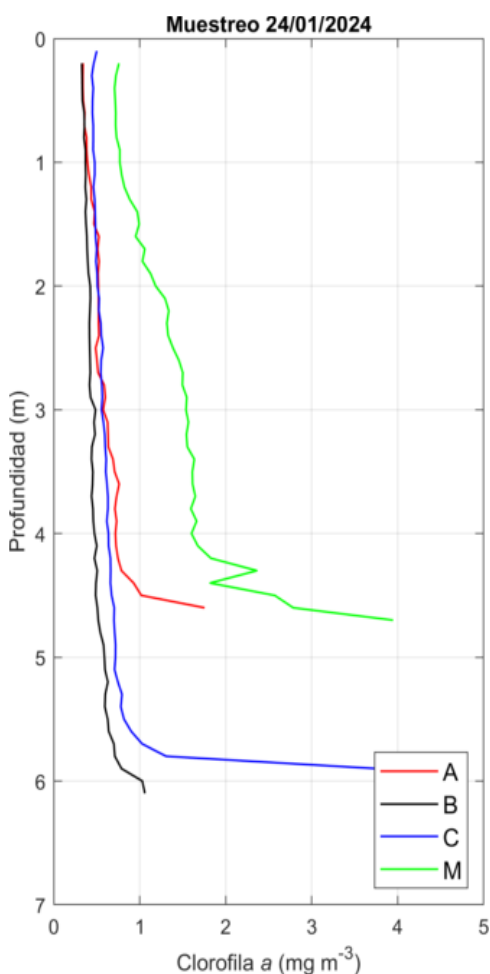
Figura 54. Perfiles de Clorofila obtenidos el día 24/01/24 con el CTD.
