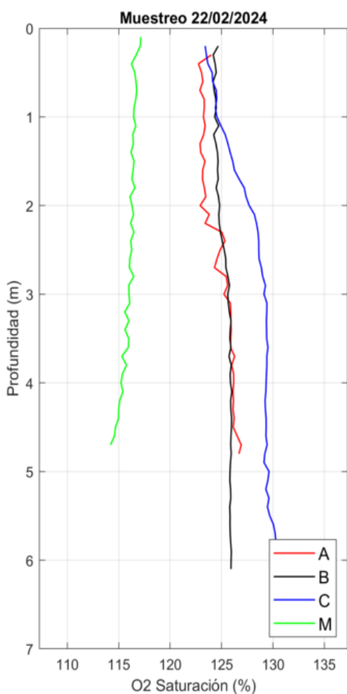
Figura 36. Perfiles de Saturación de O2 obtenidos el día 22/02/24 con el CTD.
