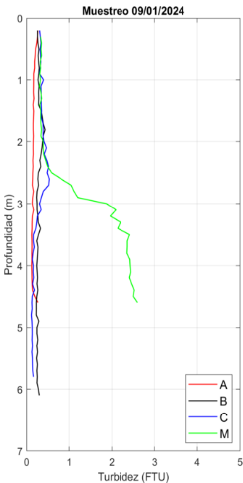
Figura 41. Perfiles de Turbidez obtenidos el día 09/01/24 con el CTD.
