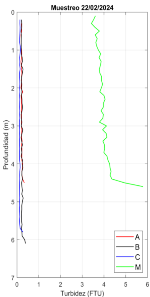
Figura 44. Perfiles de Turbidez obtenidos el día 22/02/24 con el CTD.
