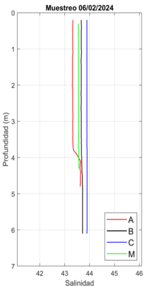
Figura 31. Perfiles de Salinidad obtenidos el día 06/02/24 con el CTD.
