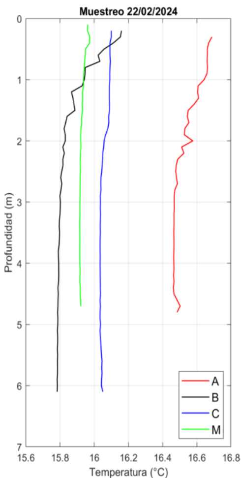
Figura 28. Perfiles de Temperatura obtenidos el día 22/02/24 con el CTD.
