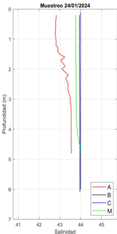
Figura 30. Perfiles de Salinidad obtenidos el día 24/01/24 con el CTD.
