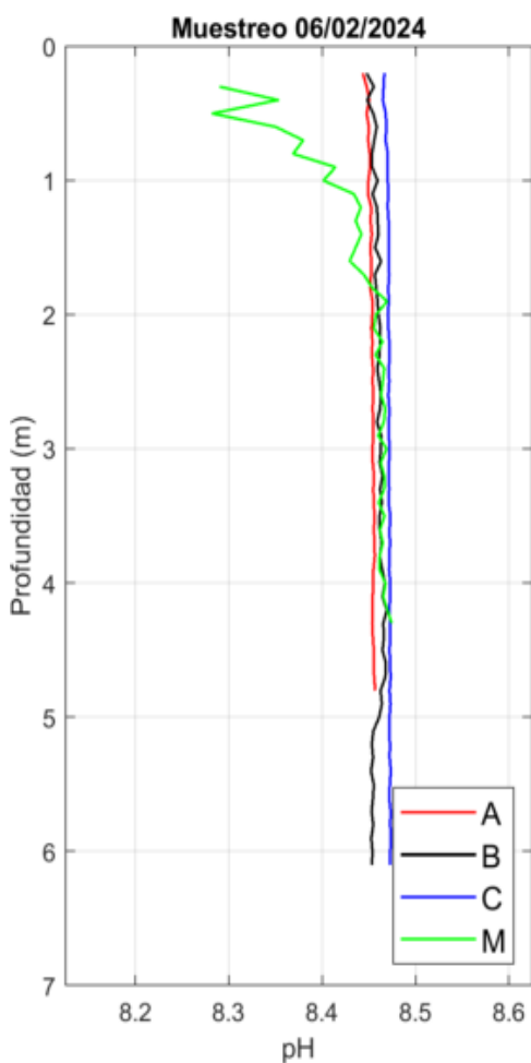
Figura 47. Perfiles de pH obtenidos el día 06/02/24 con el CTD.
