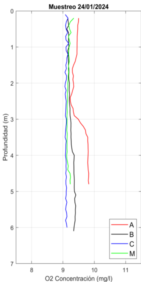
Figura 38. Perfiles de Concentración de O2 obtenidos el día 24/01/24 con el CTD.
