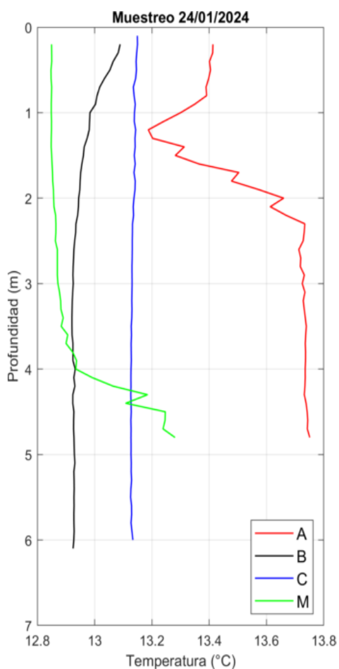
Figura 26. Perfiles de Temperatura obtenidos el día 24/01/24 con el CTD.
