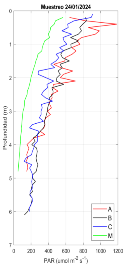
Figura 50. Perfiles de Luz PAR obtenidos el día 24/01/24 con el CTD.
