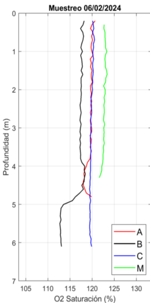
Figura 35. Perfiles de Saturación de O2 obtenidos el día 06/02/24 con el CTD.
