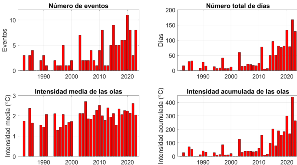
Figura 6: Estadísticas de olas de calor por año desde 1982.
