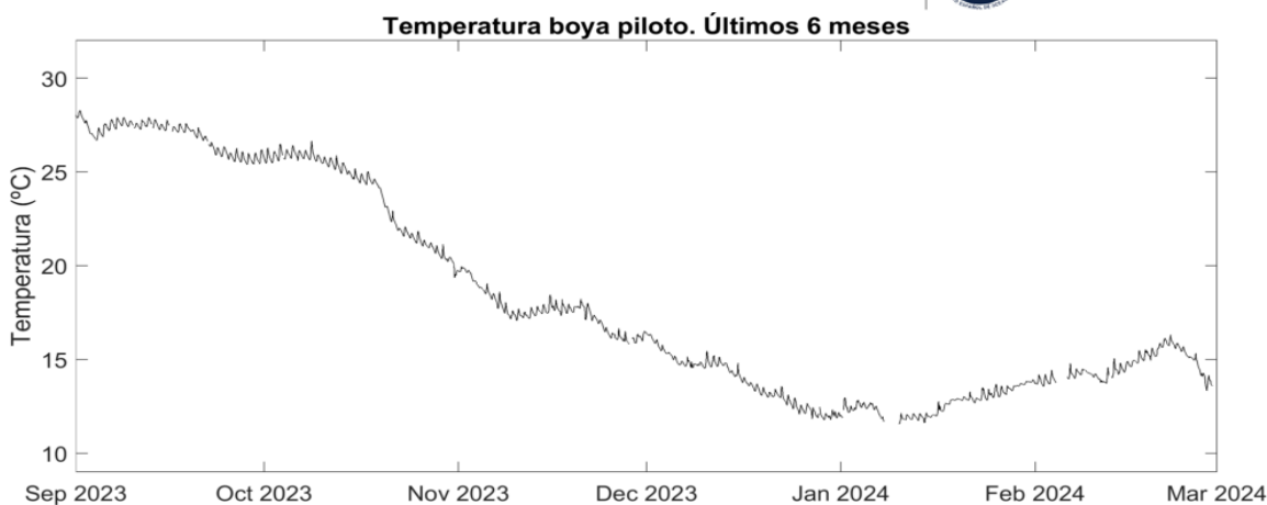
Figura 3: Serie temporal de temperatura media obtenida por los sensores térmicos de la boya piloto SMLG, calibrados con los datos de CTD obtenidos por el IEO-CSIC. En la parte superior se muestra la serie desde octubre de 2022 y en la parte inferior los últimos 6 meses.
