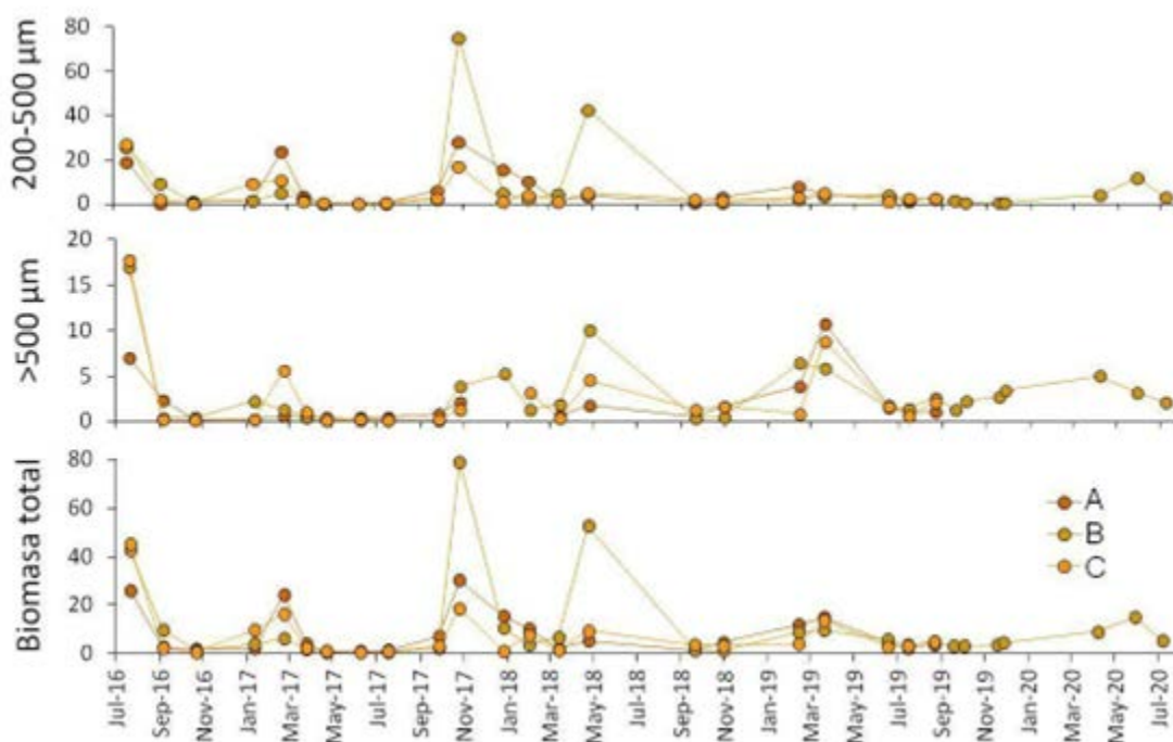
Figura 21: Variabilidad temporal de los valores de biomasa de mesozooplancton ( \text{mg peso seco} \cdot \text{m}^{-3} ) en las estaciones de muestreo A, B y C.
