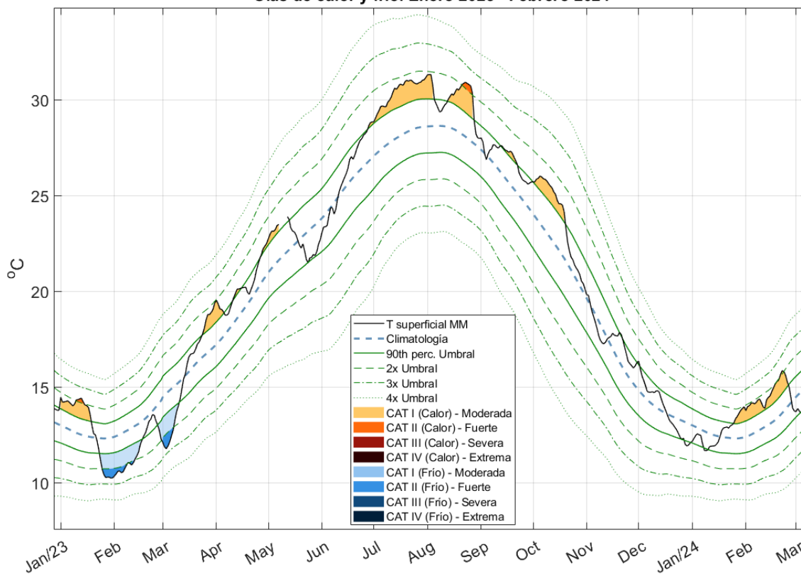
Figura 5: Serie temporal de temperatura desde enero de 2023 comparado con la climatología, mostrando las olas de calor y de frío en las categorías propuestas por Hobday et. al, (2018).
