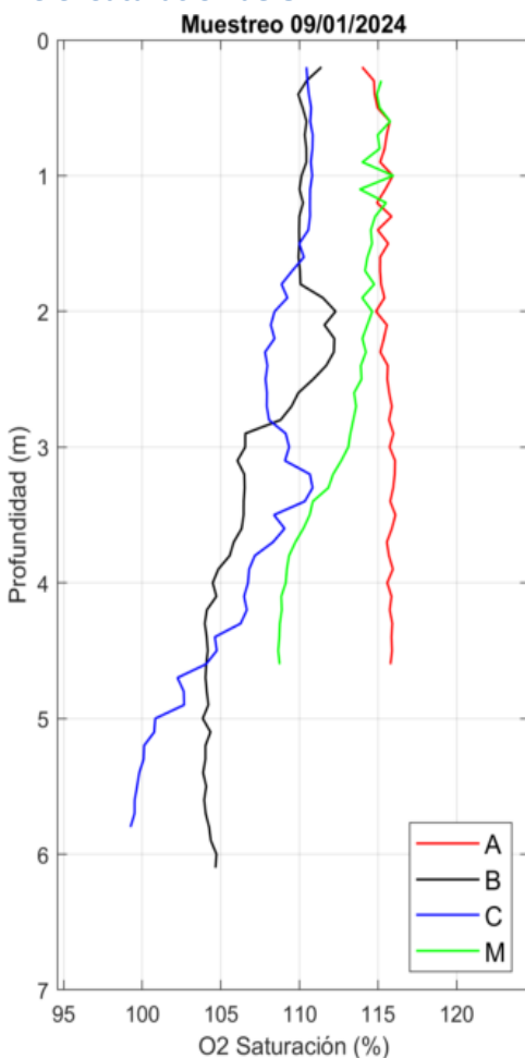
Figura 33. Perfiles de Saturación de O2 obtenidos el día 09/01/24 con el CTD.
