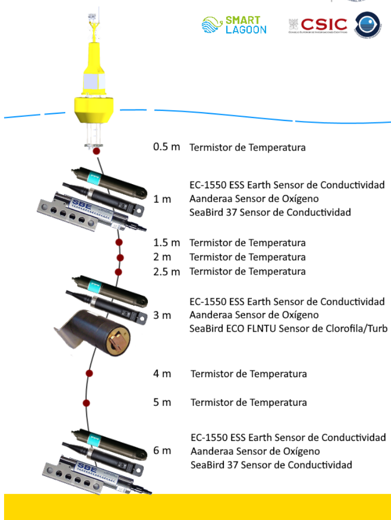
Figura 23: Esquema de los sensores instalados en la boya piloto SMLG con los nuevos sensores de temperatura, conductividad y presión a 1 y 6 metros de profundidad (Seabird-37).
