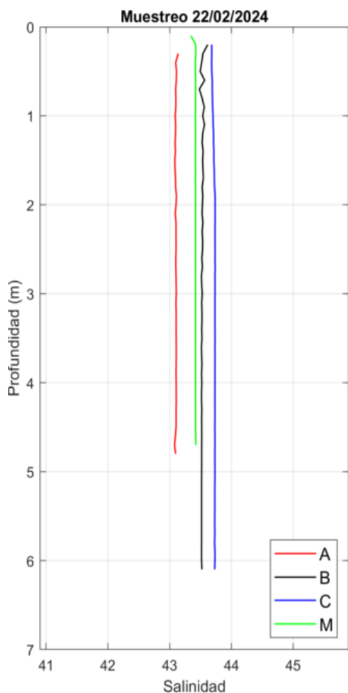
Figura 32. Perfiles de Salinidad obtenidos el día 22/02/24 con el CTD.
