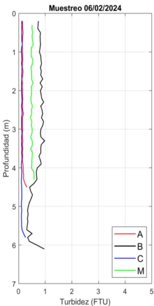
Figura 43. Perfiles de Turbidez obtenidos el día 06/02/24 con el CTD.
