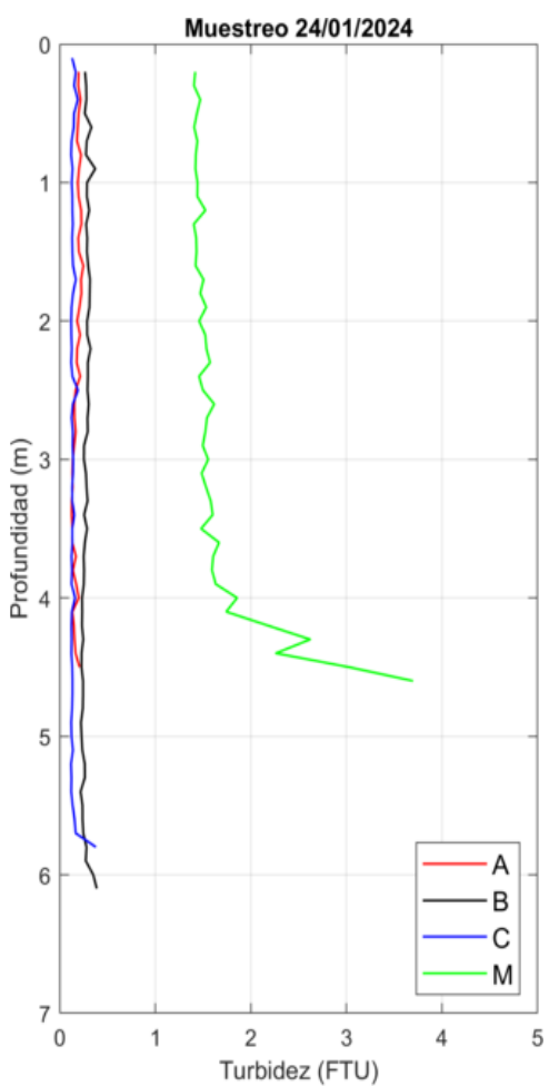
Figura 42. Perfiles de Turbidez obtenidos el día 24/01/24 con el CTD.
