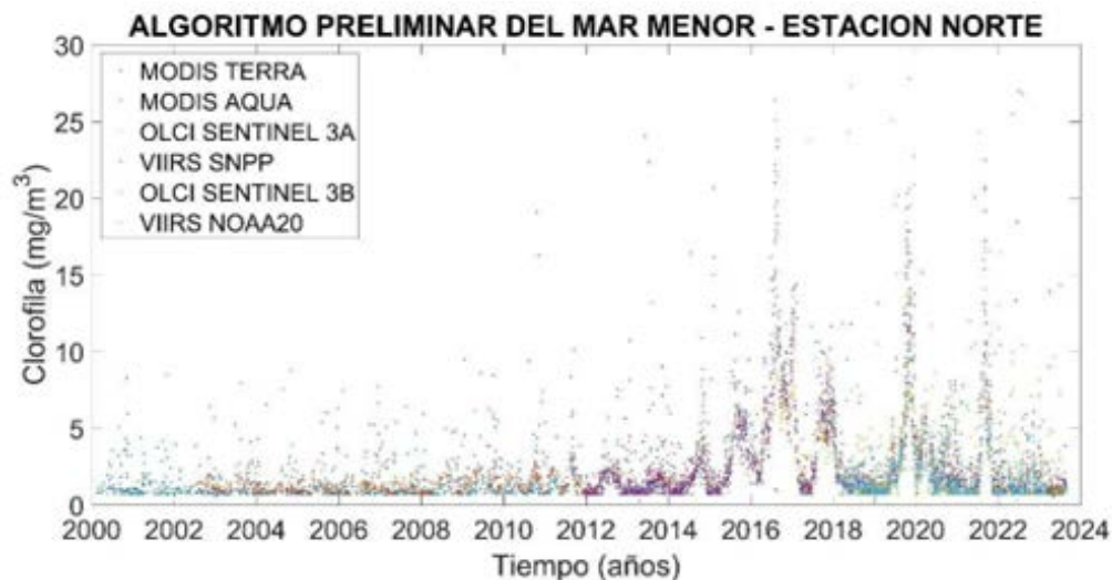
Figura 12: Evolución de la concentración de clorofila-a en una localización significativa de la cubeta norte del Mar Menor aplicando el algoritmo preliminar específico para la laguna para varios sensores satelitales.
