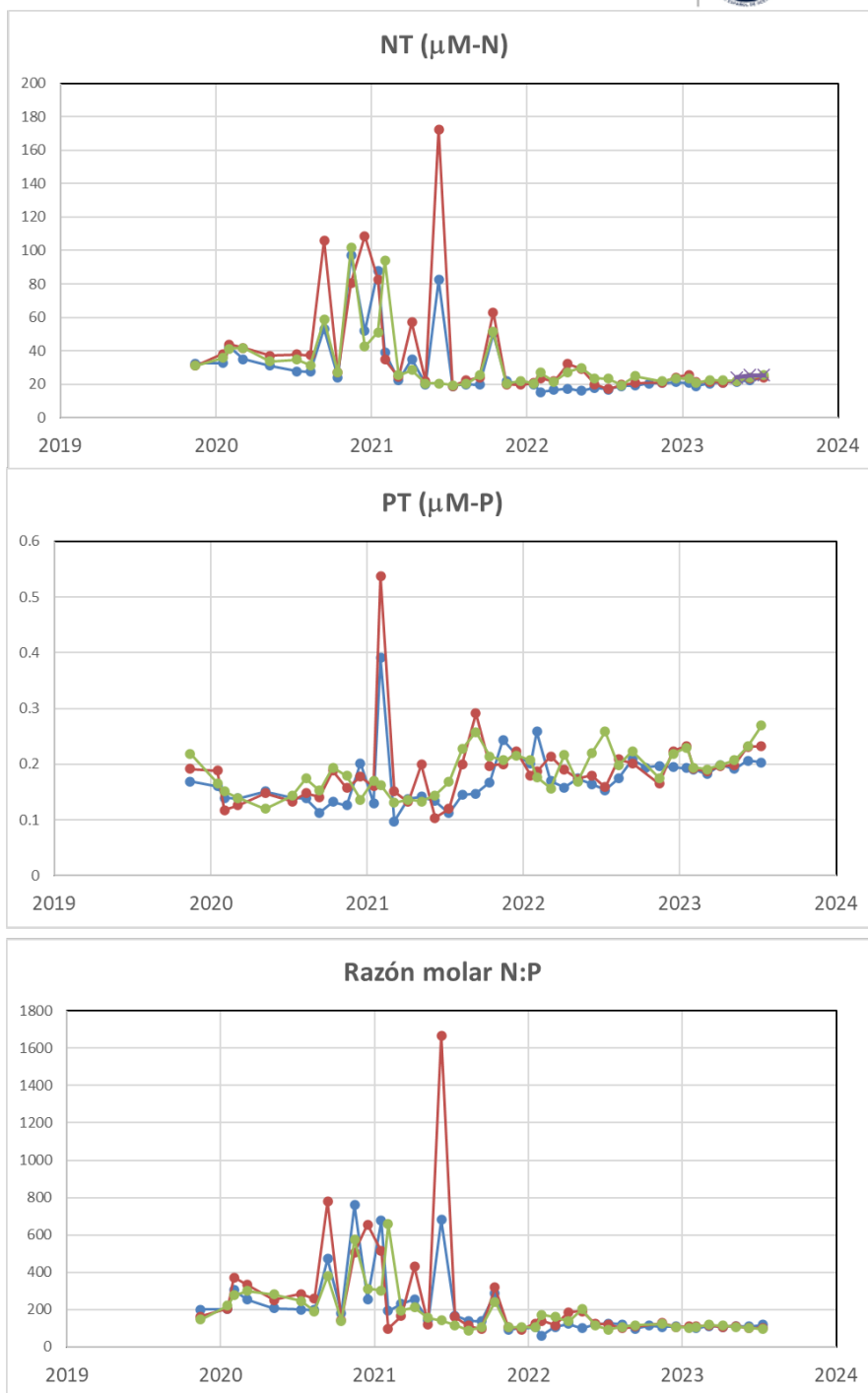
Figura 20: Variabilidad temporal de las concentraciones de nitrógeno (NT, \mu\text{M} ) y fósforo (PT, \mu\text{M} ) total en las tres estaciones de muestreo (azul: estación A; naranja: estación B; verde: estación C). Se muestra también la evolución temporal de la razón molar nitrógeno:fósforo (N:P) calculada a partir de los datos de NT y PT.
