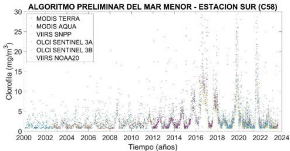
Figura 13: Evolución de la concentración de clorofila-a en una localización significativa de la cubeta sur del Mar Menor aplicando el algoritmo preliminar específico para la laguna para varios sensores satelitales.
