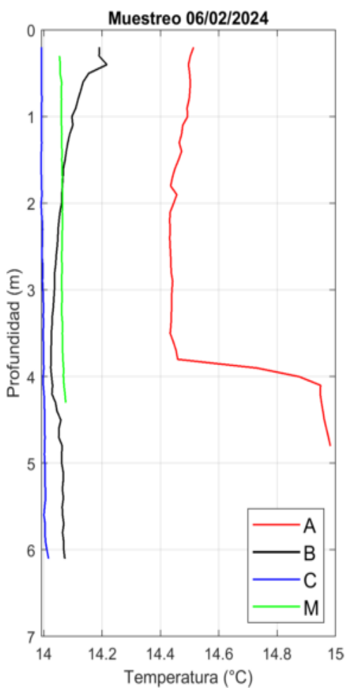
Figura 27. Perfiles de Temperatura obtenidos el día 06/02/24 con el CTD.
