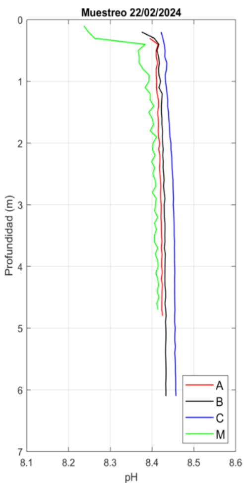
Figura 48. Perfiles de pH obtenidos el día 22/02/24 con el CTD.
