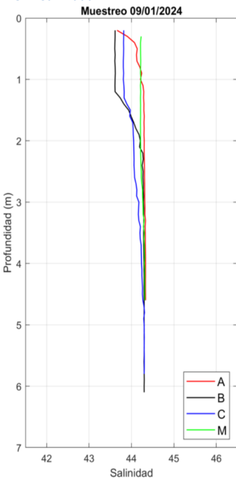
Figura 29. Perfiles de Salinidad obtenidos el día 09/01/24 con el CTD.
