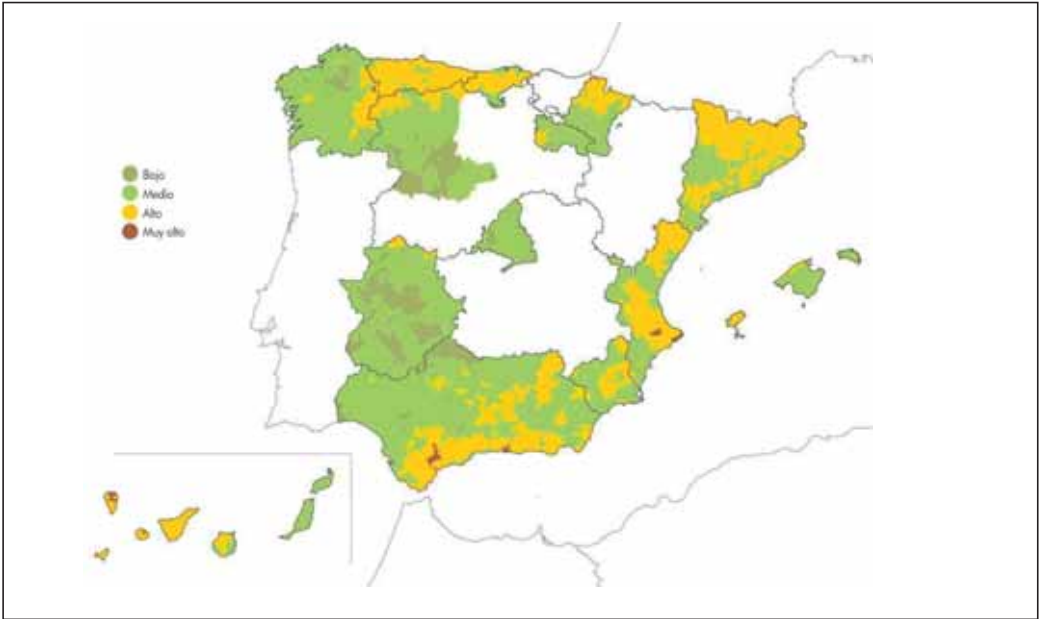
Figura 5. Cartografía de riesgo de erosión en cauces por unidades hidrológicas.
