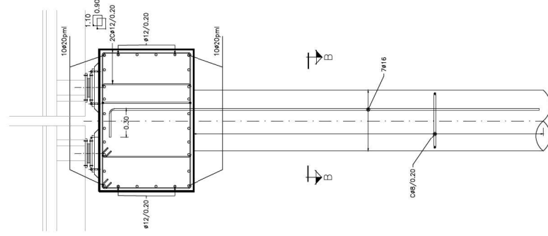
SECCIÓN B-B (NOTA: TODAS LAS COTAS ESTÁN EN METROS)
