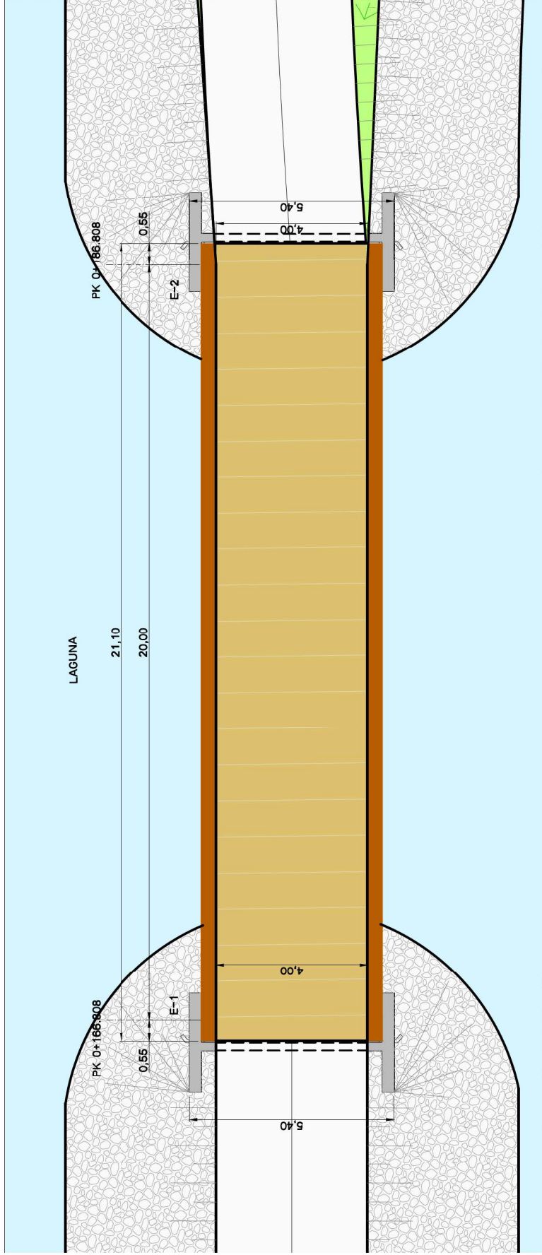
PLANTA
