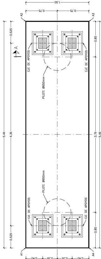
PLANTA (NOTA: TODAS LAS COTAS ESTÁN EN METROS)
