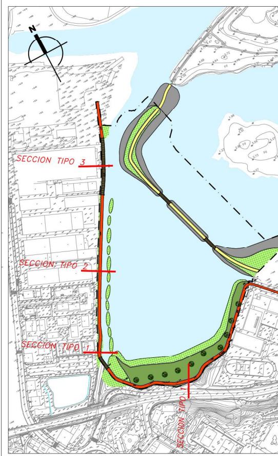
PLANTA A1: 1/2.000 A3: 1/4.000
