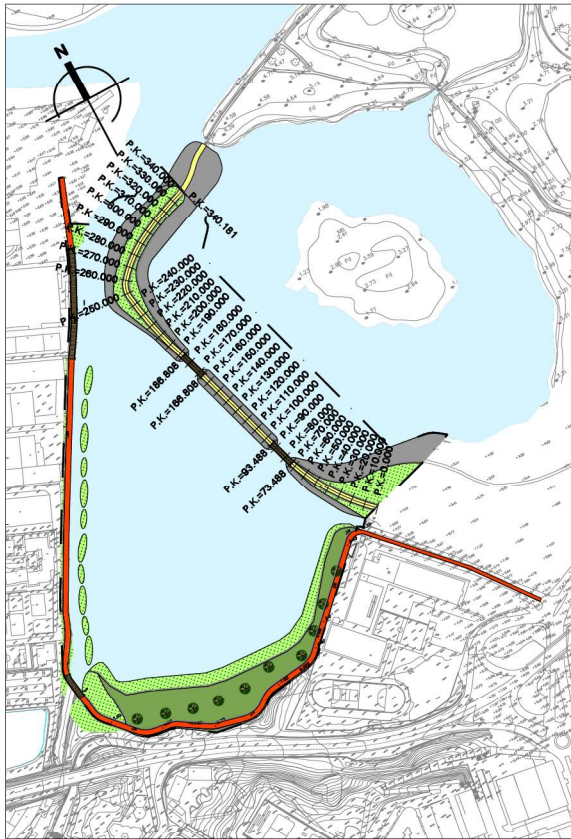
PLANTA A1: 1/2.000 A3: 1/4.000
