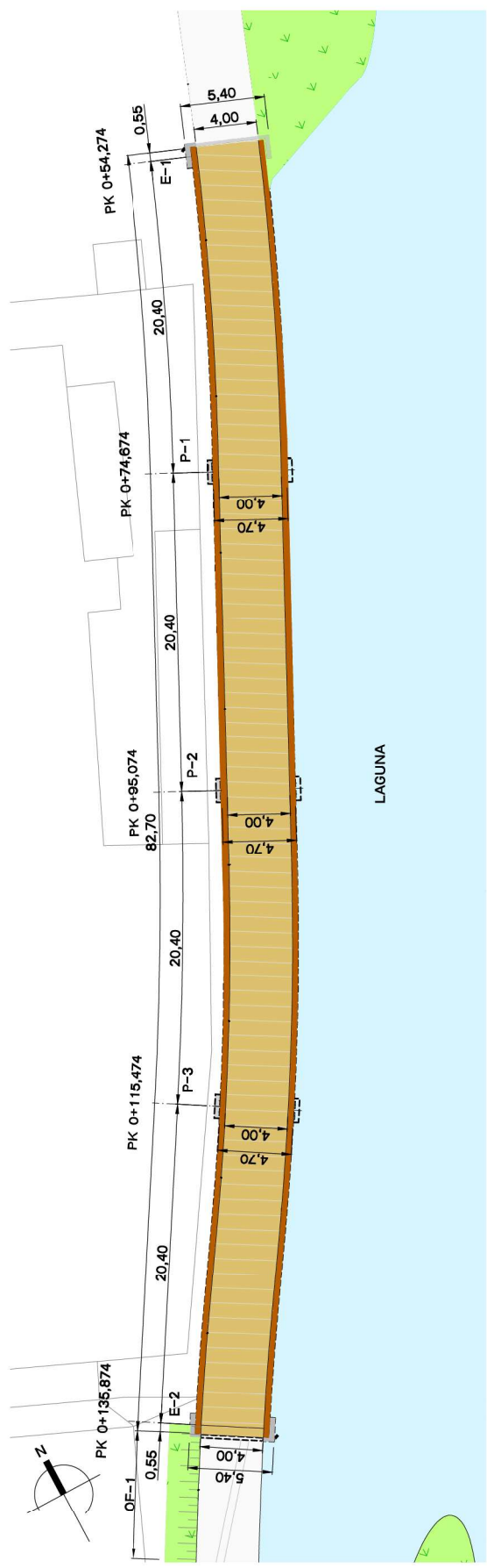
PLANTA
