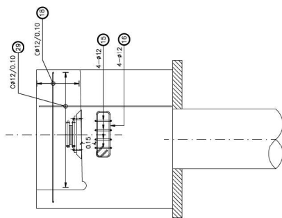
VISTA LATERAL ESCALA 1:20 (NOTA: TODAS LAS COTAS ESTÁN EN METROS)
